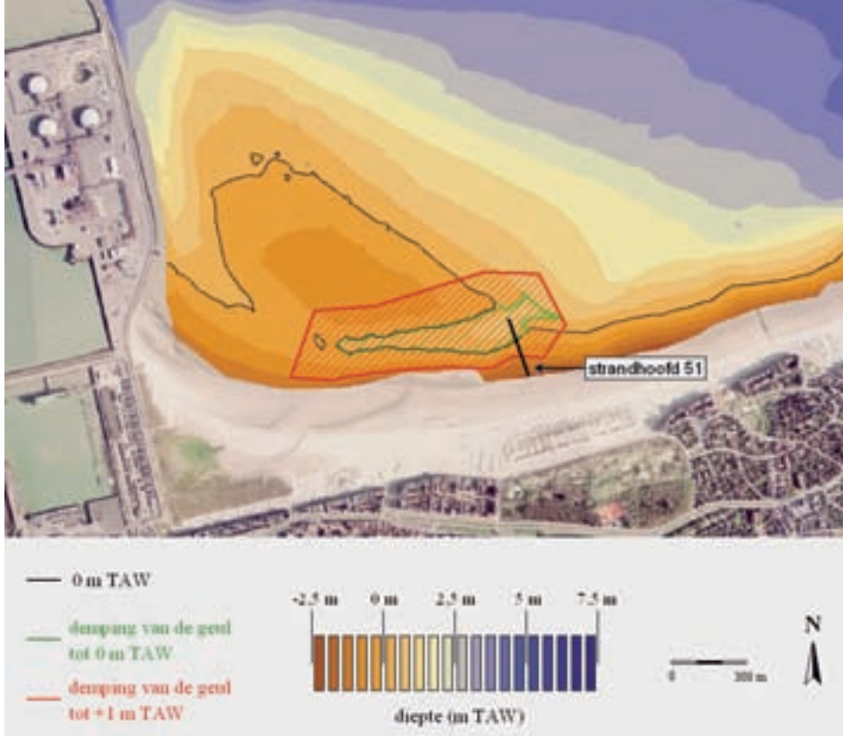
■ Demping van de geul tussen zandbank en strand – om zo het gevaar van de daar heersende sterke stromingen te bezweren – levert weinig resultaat op, blijkt uit een computersimulatie (twee opvulsscenario's, gebaseerd op vooroeverlodgingen in april 2008)
