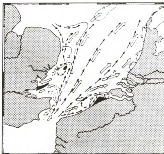
Fig. III.7. Algemeen beeld van transport van gesuspendeerd materiaal in de Zuidelijke Bocht, met: gehalten (isoplethen in \text{mg l}^{-1} ); lange termijn reststroompatroon (kleine pijlen); afgeleide transportroutes (witte pijlen); 'mud' afzettingen (minstens 50% materiaal kleiner dan 50 \mu\text{m} ; zwarte gebieden); en gebieden waar meer dan 2% materiaal kleiner dan 50 \mu\text{m} aanwezig is in het bodemsediment (omstippelde gebieden) (Eisma & Kalf, 1979).
