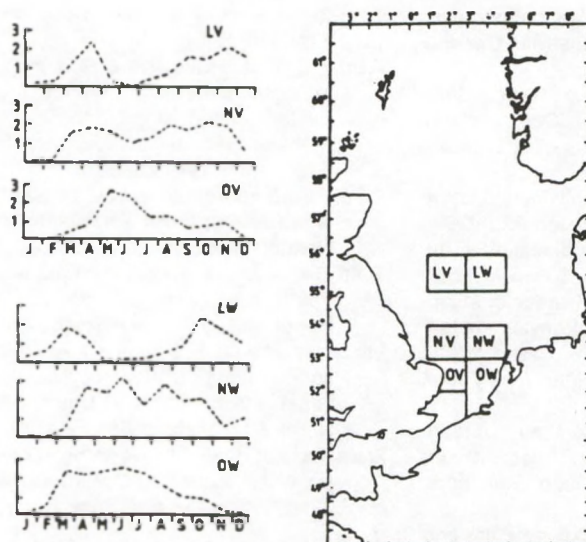
Fig. III.10. Seizoensvariatie in de fytoplankton standing stock op 10 m diepte, gemiddeld over de jaren 1949-1960, in zes deelgebieden van de Noordzee. Eenheden: arbitrair, mate van groenkleuring op gazen van de Continuous Plankton Recorder (uit: Cushing, 1973).
