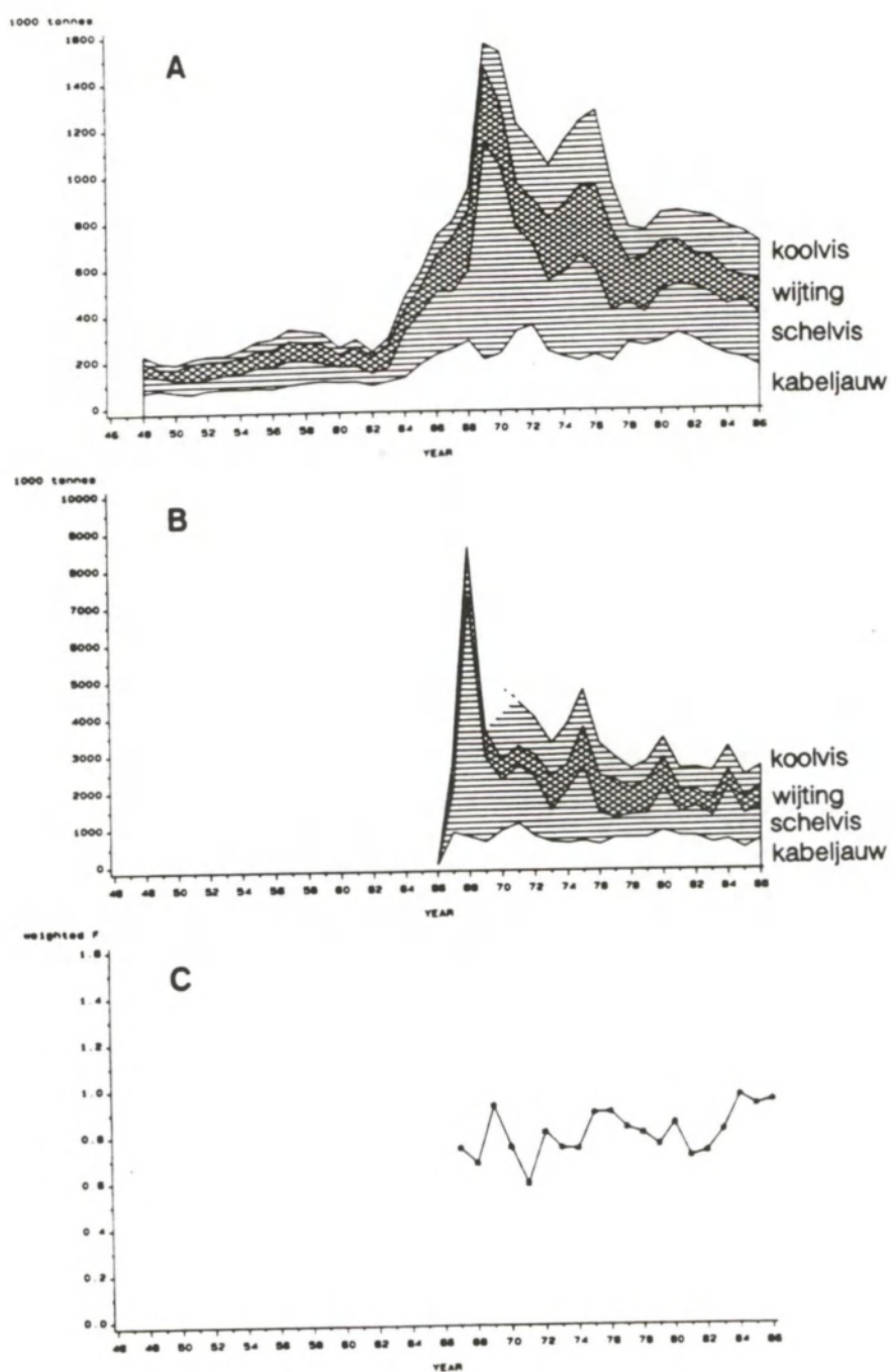
Fig. III.25. Internationale vangsten (A) en biomassa (B) van koolvis ( Pollachius virens ), wijting ( Merlangius merlangus ), schelvis ( Melanogrammus aeglefinus ) en kabeljauw ( Gadus morhua ) in de Noordzee; gewogen visserijmortaliteitscoëfficiënt (C) van deze vissoorten (bron: Daan e.a., 1990).
