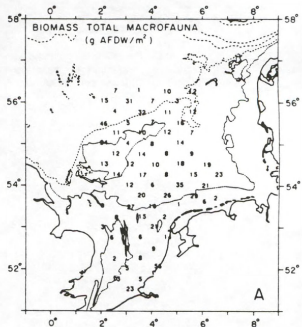
Fig. III.16. Biomassa ( \text{g AFDW} \cdot \text{m}^{-2} ) verdeling van de macrofauna (infauna) (Duineveld e.a., 1990).
