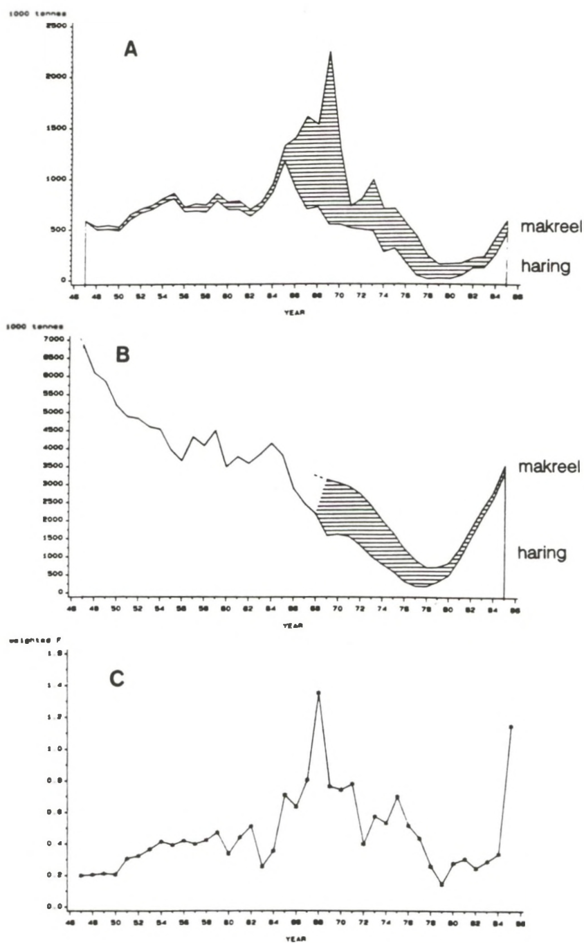
Fig. III.27. Internationale vangsten (A) en biomassa (B) van makreel ( Scomber scombrus ) en haring ( Clupea harengus ) in de Noordzee; gewogen visserijmortaliteitscoëfficiënt (C) van deze vissoorten (bron: Daan e.a., 1990).
