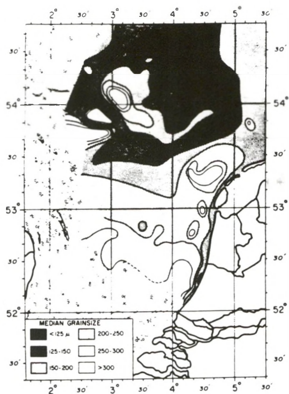
Fig. III.6. Verdeling van sedimenten op basis van mediane korrelgrootte (Creutzberg e.a., 1984).
