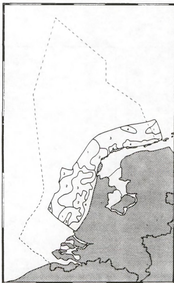
Fig. III.14. Een weergave van de clusters die voor het meiobenthos in de kustzone werden onderscheiden via een TWINSpan clusteranalyse (gemodificeerd naar Groenewold & van Scheppingen, 1990). Cluster 1: soortenrijk, totale dichtheid 180 \text{ ind-cm}^{-2} ; cluster 2: soortenrijk, totale dichtheid 90 \text{ ind-cm}^{-2} ; cluster 3: soortenarm, totale dichtheid 110 \text{ ind-cm}^{-2} ; cluster 4: soortenarm, totale dichtheid 260 \text{ ind-cm}^{-2} .
