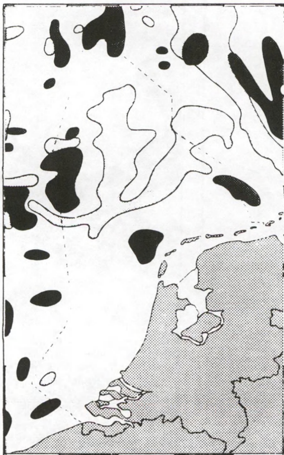
Fig. 3.3. Sedimenten in de Nederlandse sector van de Noordzee.
