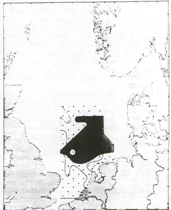
Fig. 4.4. Gebieden met uiteenlopende aantallen OBM-gevoelige soorten per station. In deze analyse zijn 17 OBM-gevoelige soorten betrokken: Montacuta ferruginosa , Scalibregma inflatum , Pholoë minuta , Amphiura filiformis , Echinocardium cordatum , Mysella bidentata , Nephtys hombergi , Lumbrineris latreilli , Chaetozone setosa , Owenia fusiformis , Nucula turgida , Gattyana cirrosa , Harpinia antennaria , Lagis koreni , Glycinde nordmanni , Cylichna cylindracea en Harmothoe longisetis .
