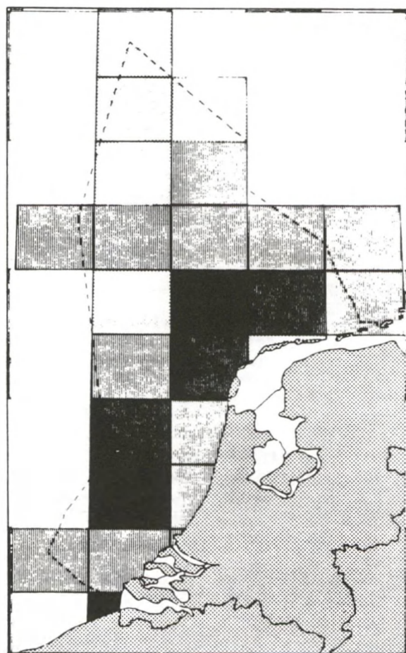
Fig. IV.1. Ruimtelijke verdeling van de boomkorvisserij over de Nederlandse sector van de Noordzee in 1982. De intensiteit in de ICES-kwadranten is uitgedrukt in aantal on gecorrigeerde visuren per 100 Mijl 2 (ca. 340 km 2 ). (Naar Wellemans, 1989).
