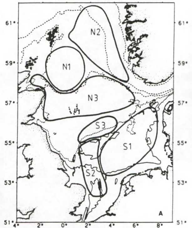
Fig. III.20. Epibenthische zones in de Noordzee naar Dyer e.a. (1983). Deze auteurs wijzen op de volgende overeenkomst met de classificatie van Glémarec (1973): S1, S2, S3 = 'infralittorale étage'; N3 = 'kust-étage' en N1, N2 = 'open-zee-étage' (Duineveld & van Noort, 1990).
