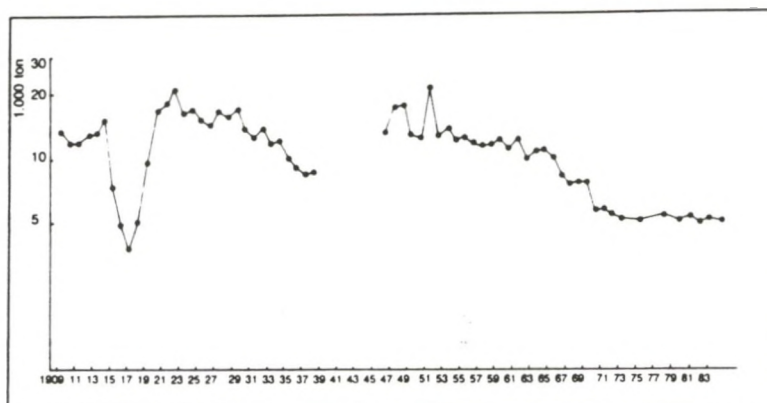
Fig. III.31. Totale vangst aan roggen en vleten in de Noordzee ( \times 10^3 ton) (naar Holden, 1978; Bull. Stat.).
