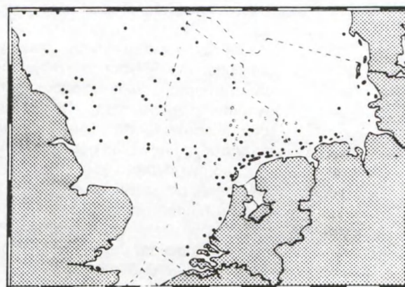
Fig. 3.12. Waarnemingen van bruinvissen ( P. phocoena ) in de Noordzee, 1984-1990.
