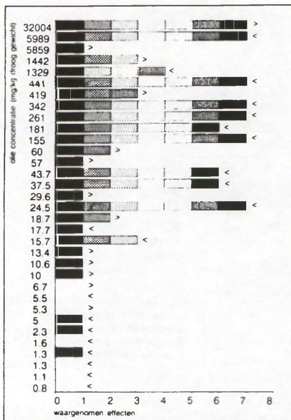
Fig. IV.5. Samenvatting van de waargenomen typen effecten bij contaminatie variërend van 0,8 tot 32.000 mg olie (uit OBM) per kg sediment.
