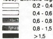
Fig. III.8. Troebeling (lichtextinctie) met het reststroompatroon in de zuidelijke Noordzee. Men ziet twee advectieve 'mud'stroom, één overstekend, en één noordwaarts trek-kend langs de Nederlandse kust. In de laatste zijn de totale sedimentconcentraties het hoogst van de twee (McCave, 1983). Extinctie tegen gedistilleerd water:
