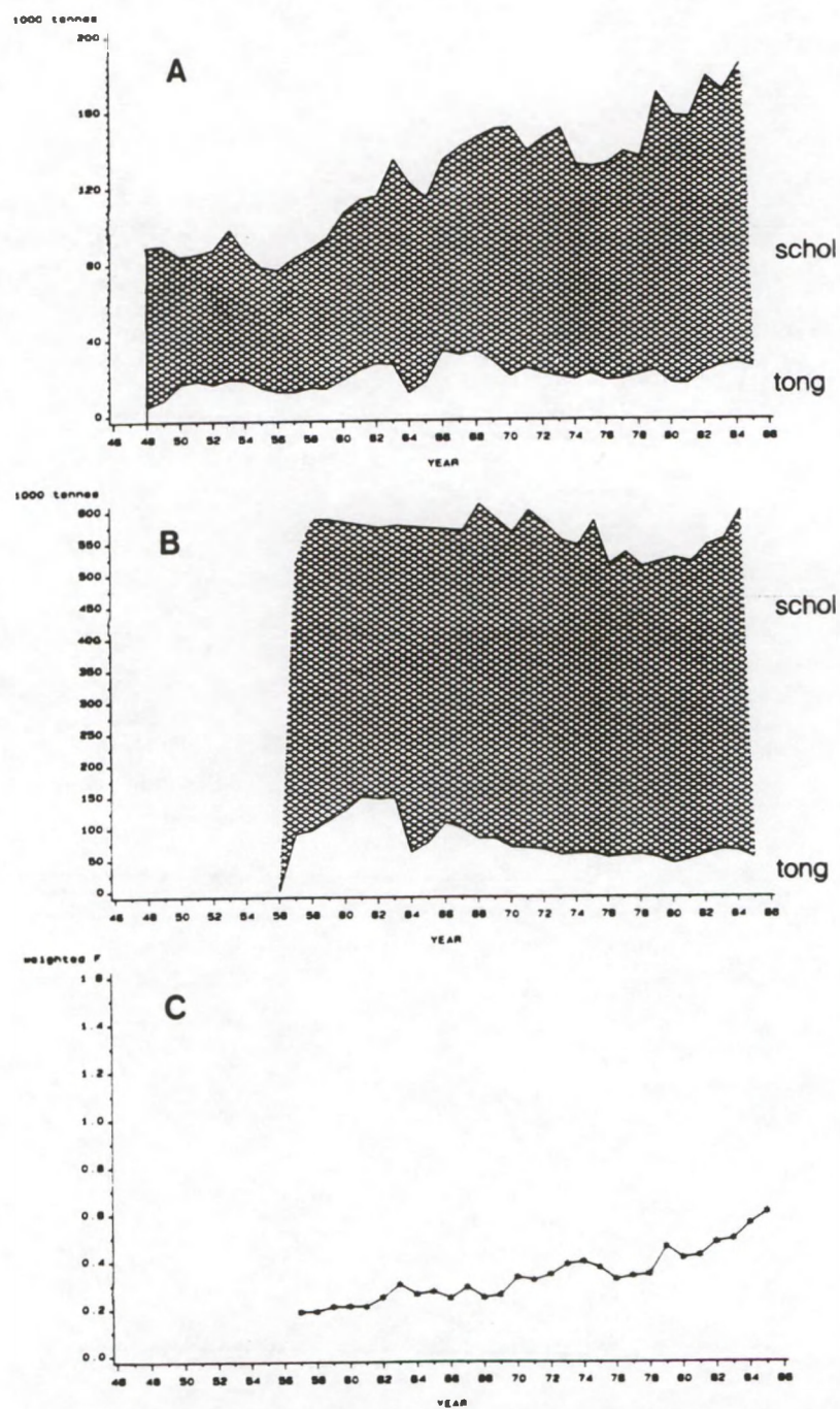
Fig. III.30. Internationale vangsten (A) en biomassa (B) van schol ( Pleuronectes platessa ) en tong ( Solea solea ) in de Noordzee; gewogen visserijmortaliteitscoëfficiënt (C) van deze vissoorten (bron: Daan e.a., 1990).
