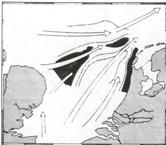
Fig. III.8. Troebeling (lichtextinctie) met het reststroompatroon in de zuidelijke Noordzee. Men ziet twee advectieve 'mud'stroom, één overstekend, en één noordwaarts trek-kend langs de Nederlandse kust. In de laatste zijn de totale sedimentconcentraties het hoogst van de twee (McCave, 1983). Extinctie tegen gedistilleerd water:
