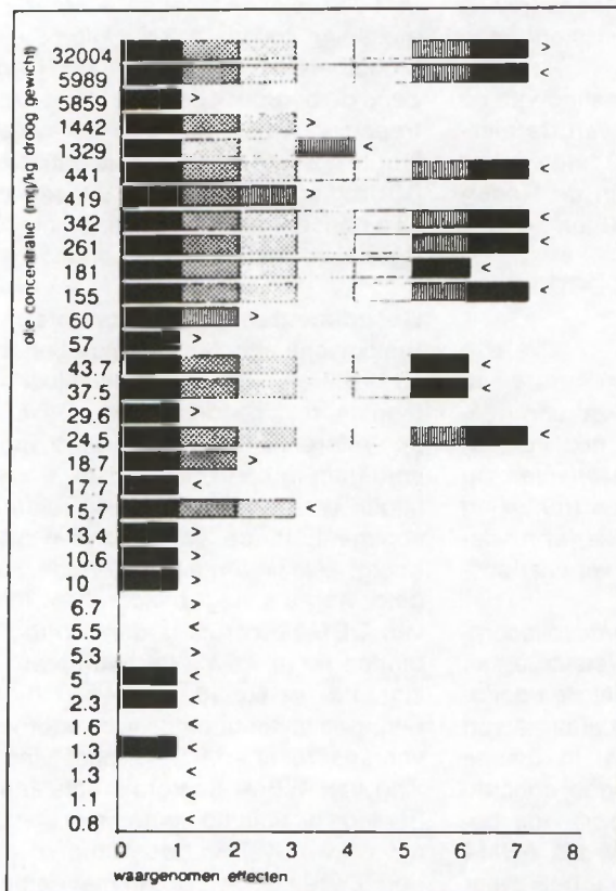
Fig. 4.3. Samenvatting van de waargenomen typen effecten bij contaminatie variërend van 0,8 tot 32.000 mg olie (uit OBM) per kg sediment.
