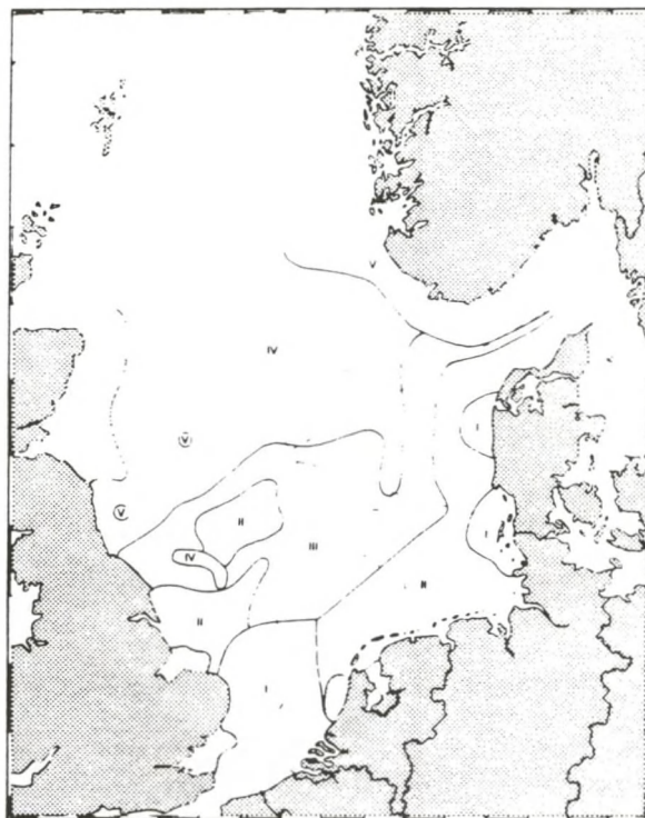
Fig. III.13. Clusterindeling van copepoden (meiobenthos) in de Noordzee, gebaseerd op dichtheden, soortensamenstelling en diversiteit; — niet bemonsterde gebieden (naar Huys e.a., 1990).
