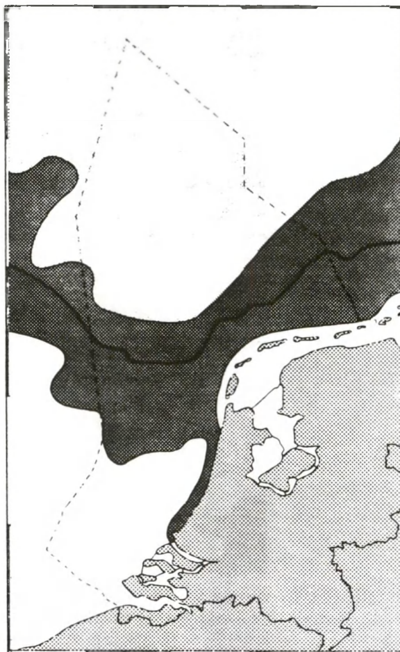
Fig. III.2. Theoretische ligging van het zomerse getijdefront in de Nederlandse sector van de Noordzee.
