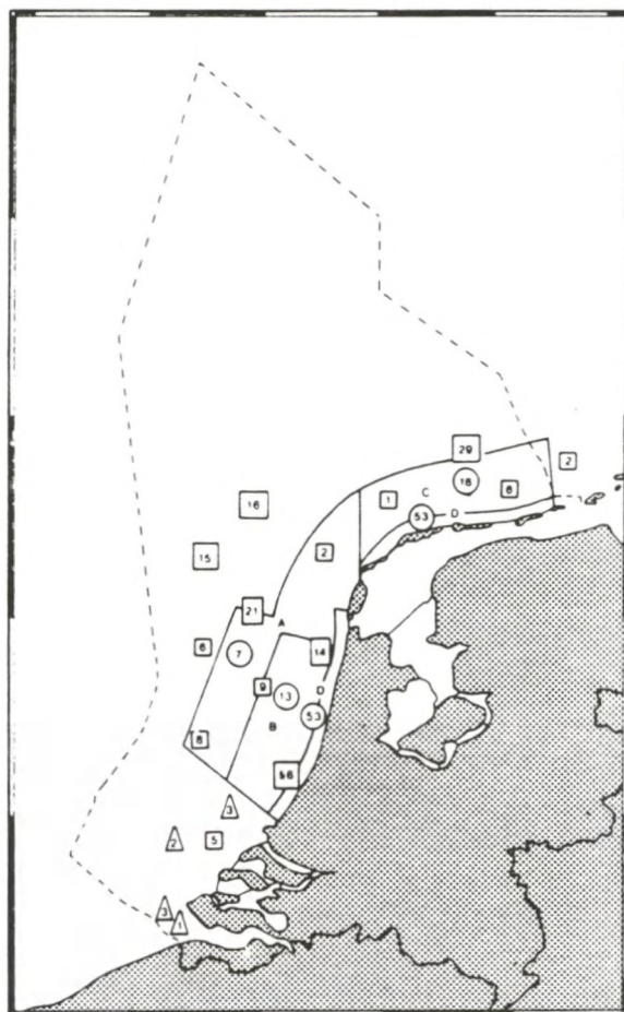
Fig. III.18. Clusterindeling en biomassa ( \text{g AFDW} \cdot \text{m}^{-2} ) van het macrobenthos (infauna) in de Zuidelijke Bocht en het Nederlandse kustgebied.
