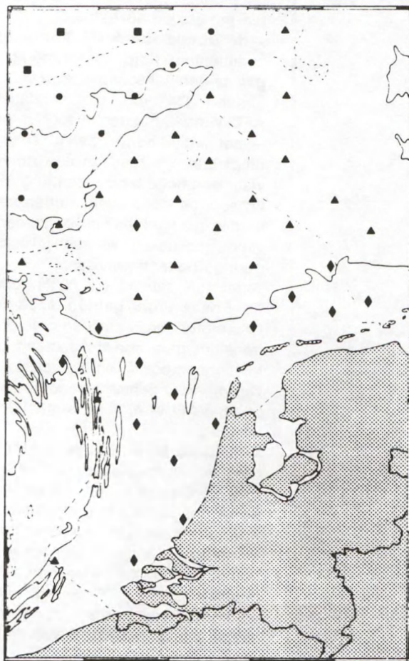
Fig. 3.8. Indeling van de epifauna in de Nederlandse sector van de Noordzee in clusters.
