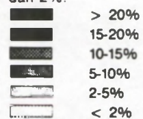
Fig. III.9. De Oostergonden, globaal te omschrijven als een gebied met een 'mud'gehalte (deeltjes < 50 \mu\text{m} ) van meer dan 2%.
