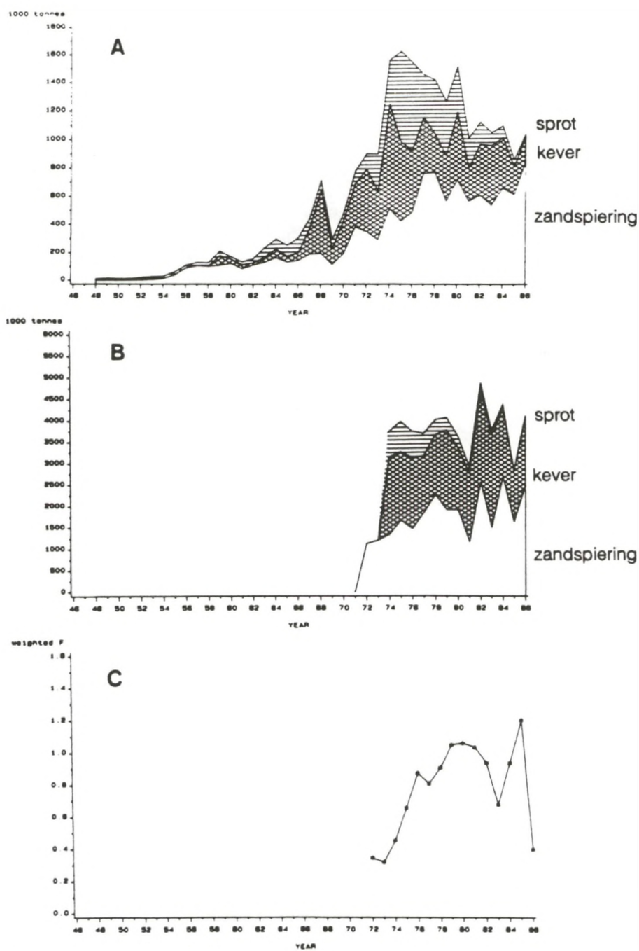
Fig. III.29. Internationale vangsten (A) en biomassa (B) van sprot ( Sprattus sprattus ), kever ( Trisopterus esmarkii ) en zandspiering ( Ammoditydæ ) in de Noordzee; gewogen visserij-mortaliteitscoëfficiënt (C) van deze vissoorten (bron: Daan e.a., 1990).
