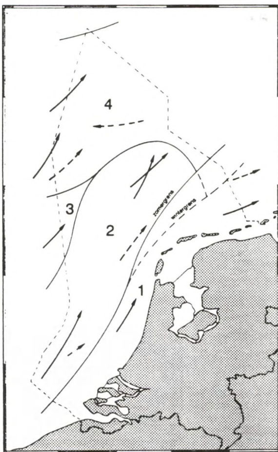
Fig. 3.1. De verschillende watermassa's in de Nederlandse sector van de Noordzee in zomer en winter: 1 Continentaal kustwater; 2 Kanaalwater; 3 Engels kustwater; 4 Centrale Noordzeewater —→ oppervlakte-reststroom ---→ bodem-reststroom (naar Laevastu, 1963).
