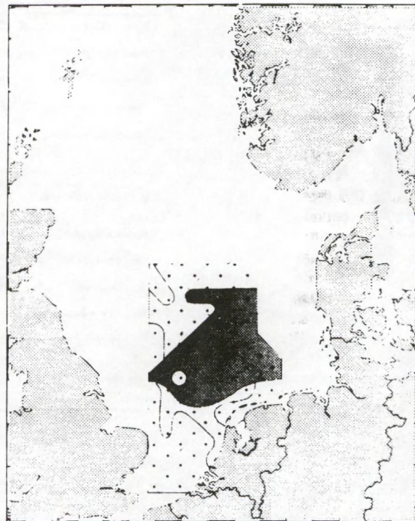
Fig. IV.6. Gebieden met uiteenlopende aantallen OBM-gevoelige soorten per station. In deze analyse zijn 17 OBM-gevoelige soorten betrokken: Montacuta ferruginosa , Scalibregma inflatum , Pholoë minuta , Amphiura filiformis , Echinocardium cordatum , Mysella bidentata , Nephtys hombergi , Lumbrineris latreilli , Chaetozone setosa , Owenia fusiformis , Nucula Turgida , Gattyana cirrosa , Harpinia antennaria , Lagis koreni , Glycinde nordmanni , Cylichna cylindracea en Harmothoe longisetis .
