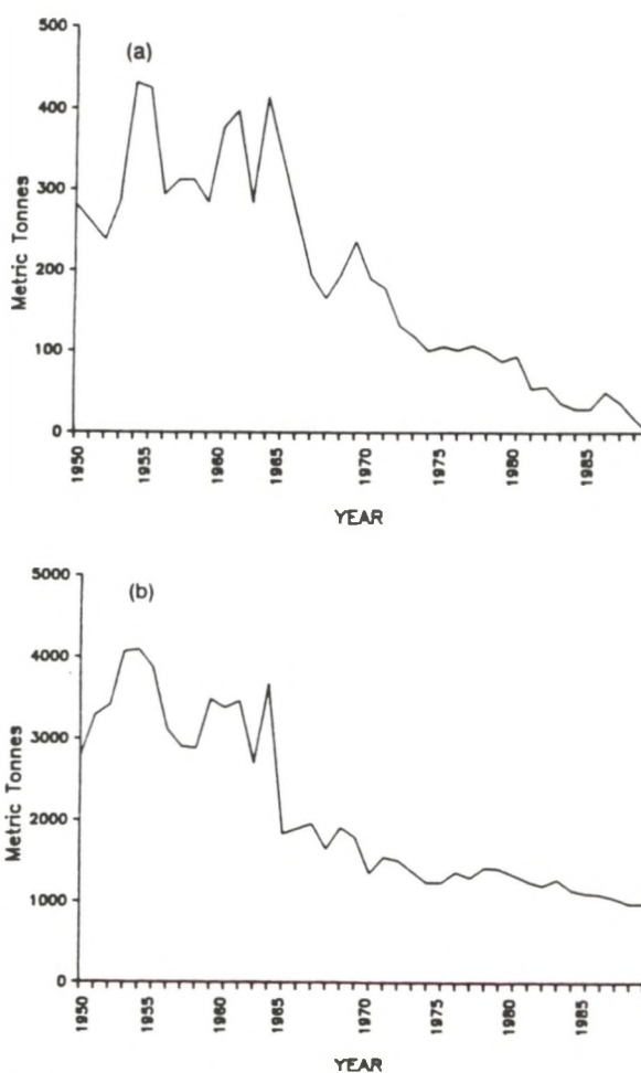
Fig. III.32. Totale aanvoer van rog en vleet vanuit: (a) Doggersbank; (b) hele Noordzee (Purdon & Garrod, 1990).
