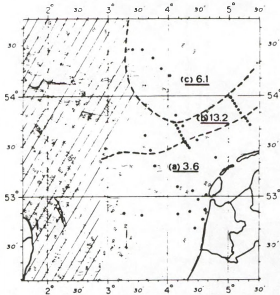
Fig. III.19. Gemiddelde biomassa (g AFDW \text{m}^{-2} ) van de macrofauna in: (a) Zuidelijke Bocht (b) Friese Front gebied (c) Oestergronden (Creutzberg e.a., 1984).
