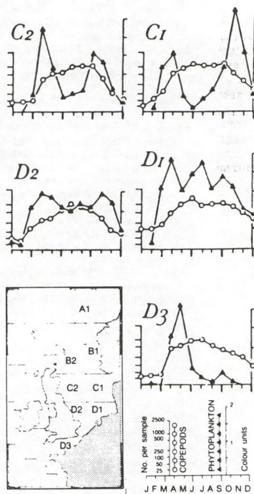
Fig. III.11. Gemiddelde seizoensvariatie (over 1948-1960) van dichtheid van fytoplankton en copepoden in de zg. standard areas (N.B.: ongelijk aan de deelgebieden van Fig. III.10. !) (uit: Colebrook & Robinson, 1965)
