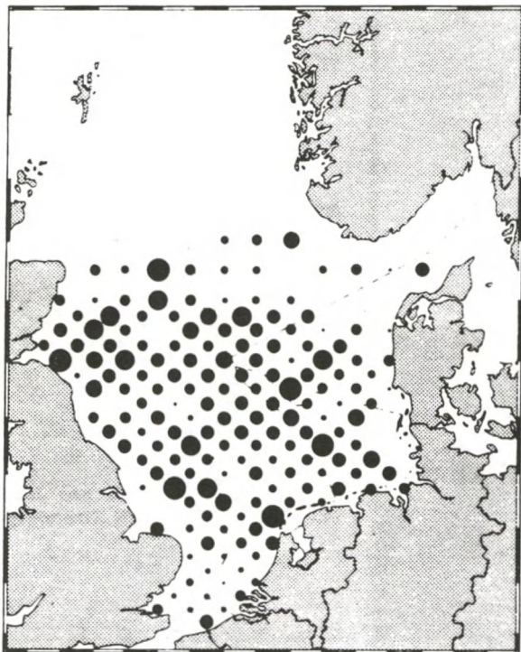
Fig. III.12. De relatieve dichtheid van nematoden in de Noordzee (straal van de cirkel is evenredig aan \log(\text{dichtheid}+1) ) (Huys e.a., 1990).
