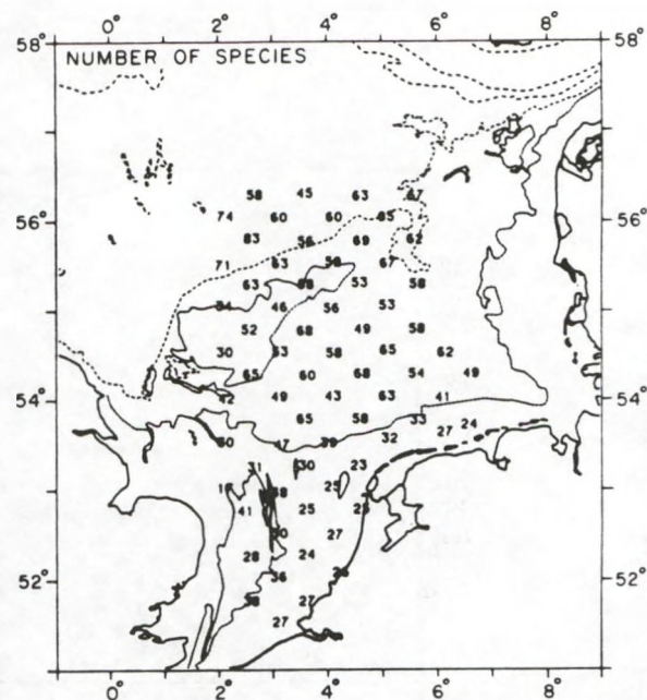
Fig. III.15. Soortenrijkdom van de macrofauna (infauna) (aantal soorten in 0.3 \text{ m}^2 ) (Duineveld e.a., 1990).
