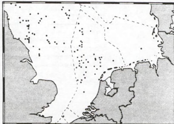
Fig. III.35. Waarnemingen van witsnuitdolfijnen ( L. albirostris ), witflankdolfijnen ( L. acutus ) en niet geïdentificeerde dolfijnen ( L. spec. ) in de Noordzee, 1984-1990. ● waarnemingen vanaf een schip; ○ waarnemingen vanuit een vliegtuig (naar ongepubliceerde gegevens van H.J.M. Baptist, C.J. Camphuysen en M.F. Leopold).
