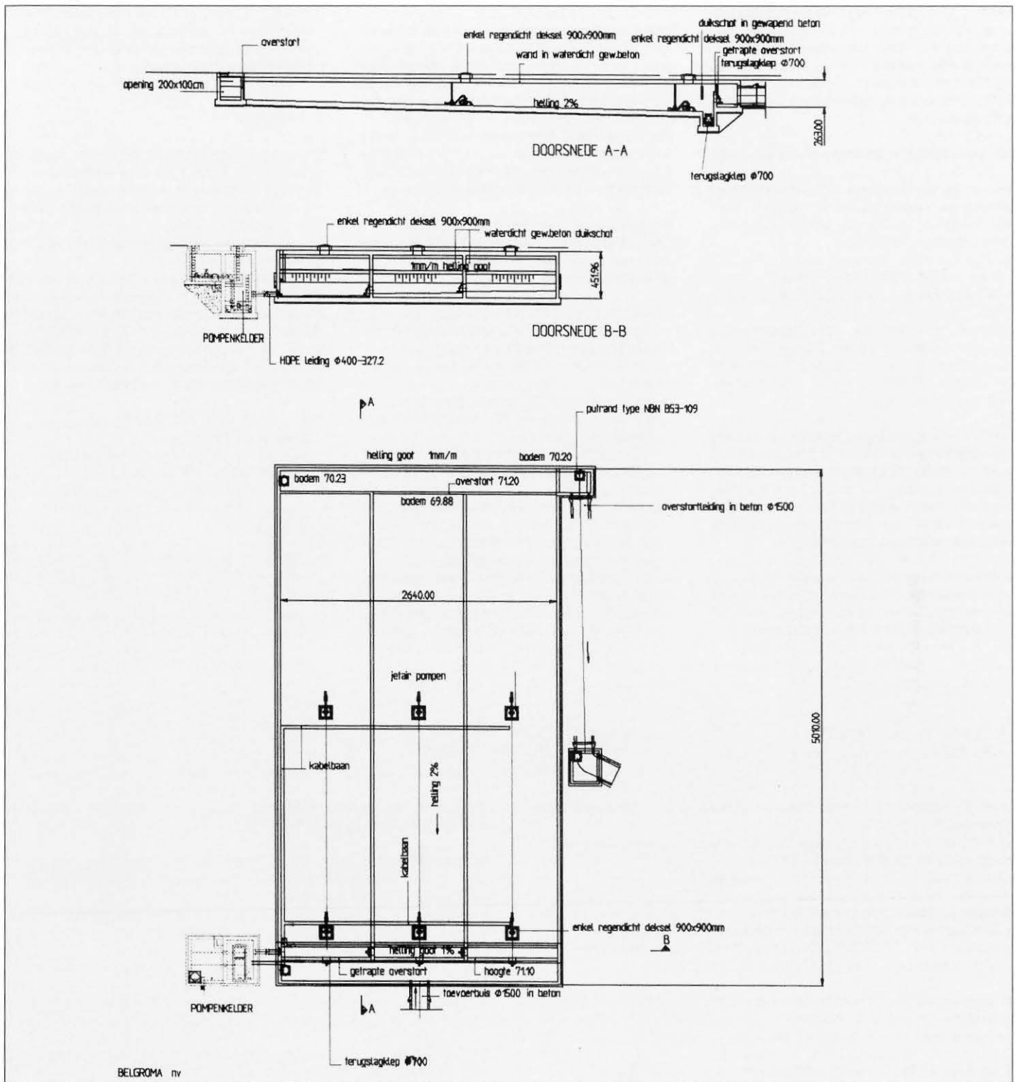
Fig. 3 : Bergbezinkbassin.
