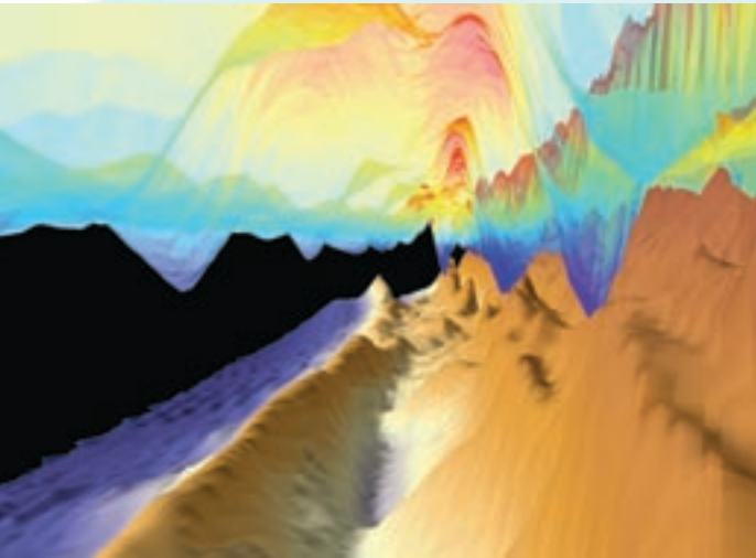
3D-weergave van de bodem bij Terschelling. Een blik in de trog tussen de buitenste twee banken. In het midden, als een bult, de onderwatersuppletie van 1993. (Hemel: verschilbeeld bodemligging tussen 2000 en 1993. Rood: sedimentatie; blauw: erosie.)
