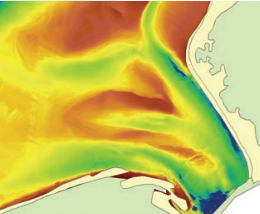
Bodemmetingen in de Haringvlietmonding (1970 en 2000) illustreren hoe het gebied al veranderde onder invloed van het afsluiten van het Haringvliet. (Blauw: diep; rood: ondiep.)
