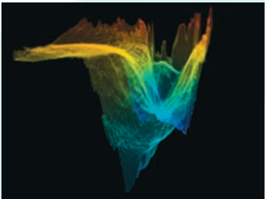
Deel van een geulbodem (geul bij Hansweert in de Westerschelde).
