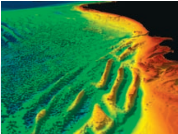
De Noordzeebodem met rechts de Nederlandse kust.
