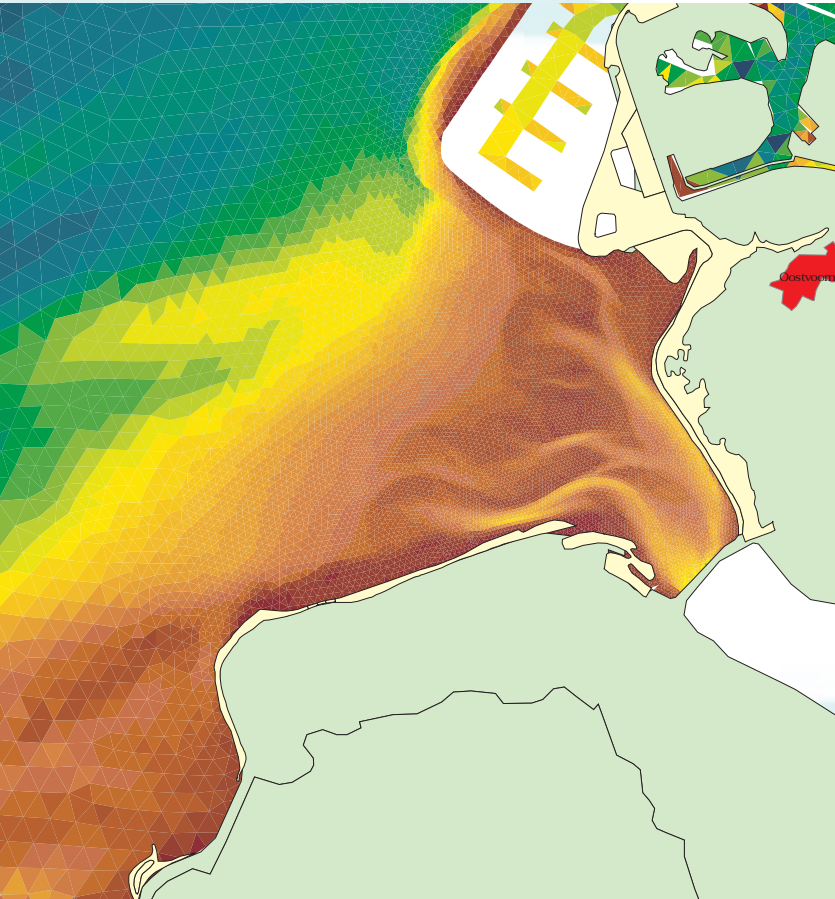
Voorspellingen volgens twee modelmethodieken voor de bodemligging in 2010, scenario Maasvlakte II en gedeeltelijk sluisopening (getemd getij.) Let op de verschillen in het geulenpatroon in de Haringvlietmonding.
