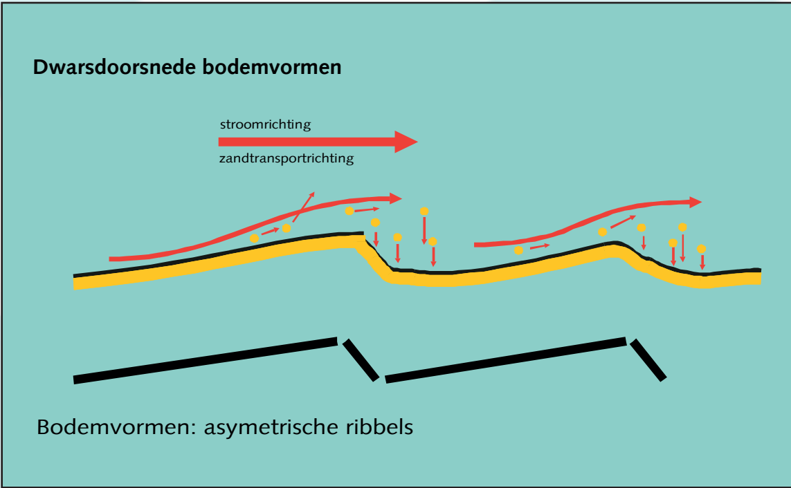
Asymmetrische bodemvormen verraden de stroomrichting
