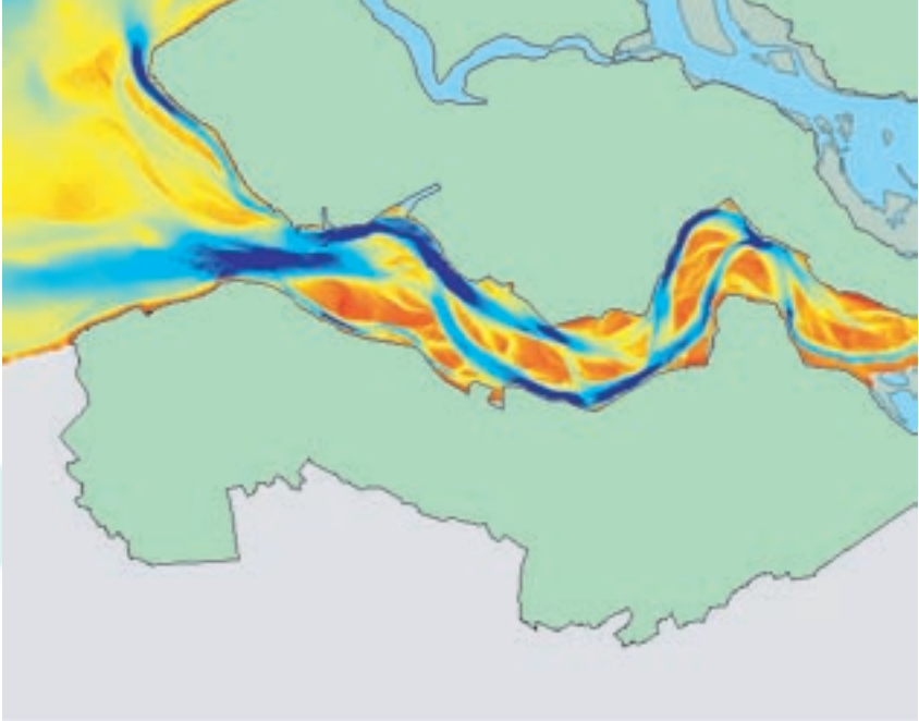
De bodemligging in 1968 en 1998 en het verschilbeeld (onderste plaatje). De bodem in dit dynamisch gebied is duidelijk veranderd (rood: aanzanding, blauw: verdieping).
