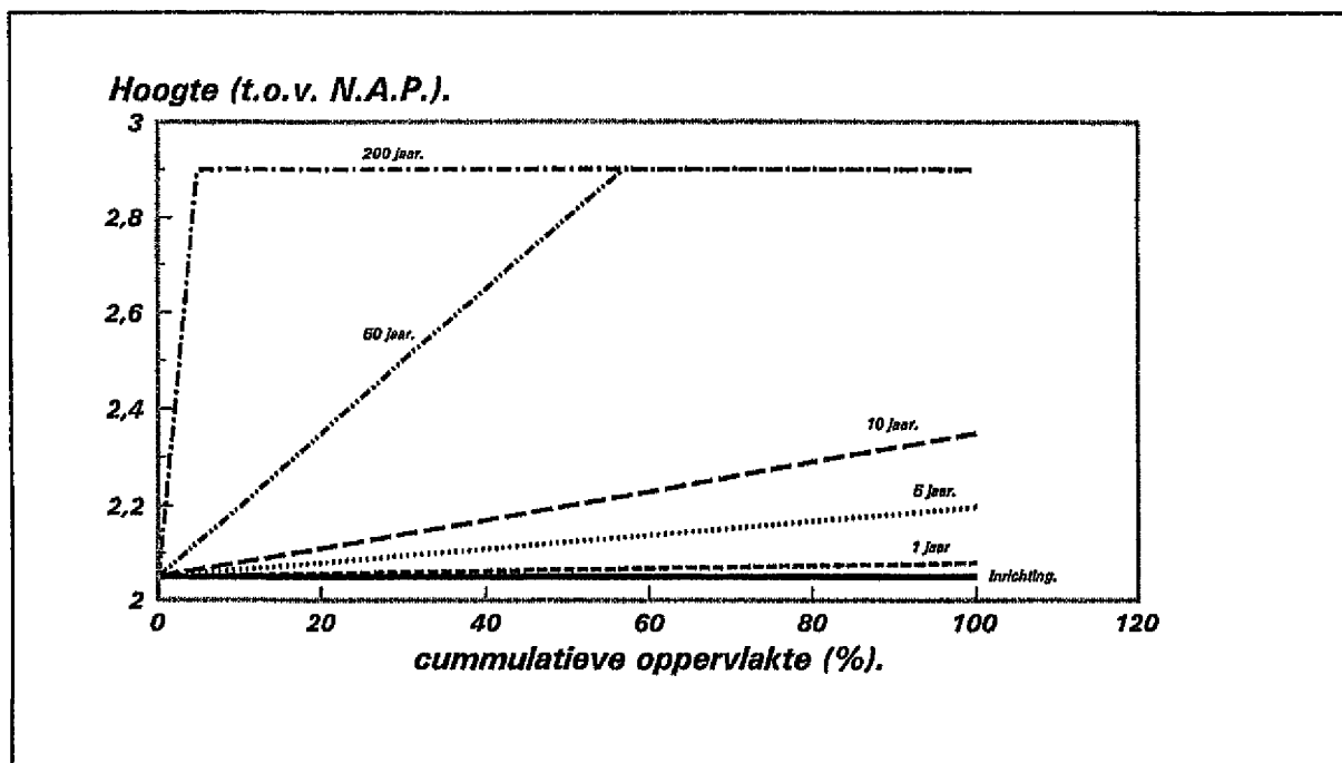
Grafiek 4.5.: Verloop oppervlakte per hoogte in de tijd.
