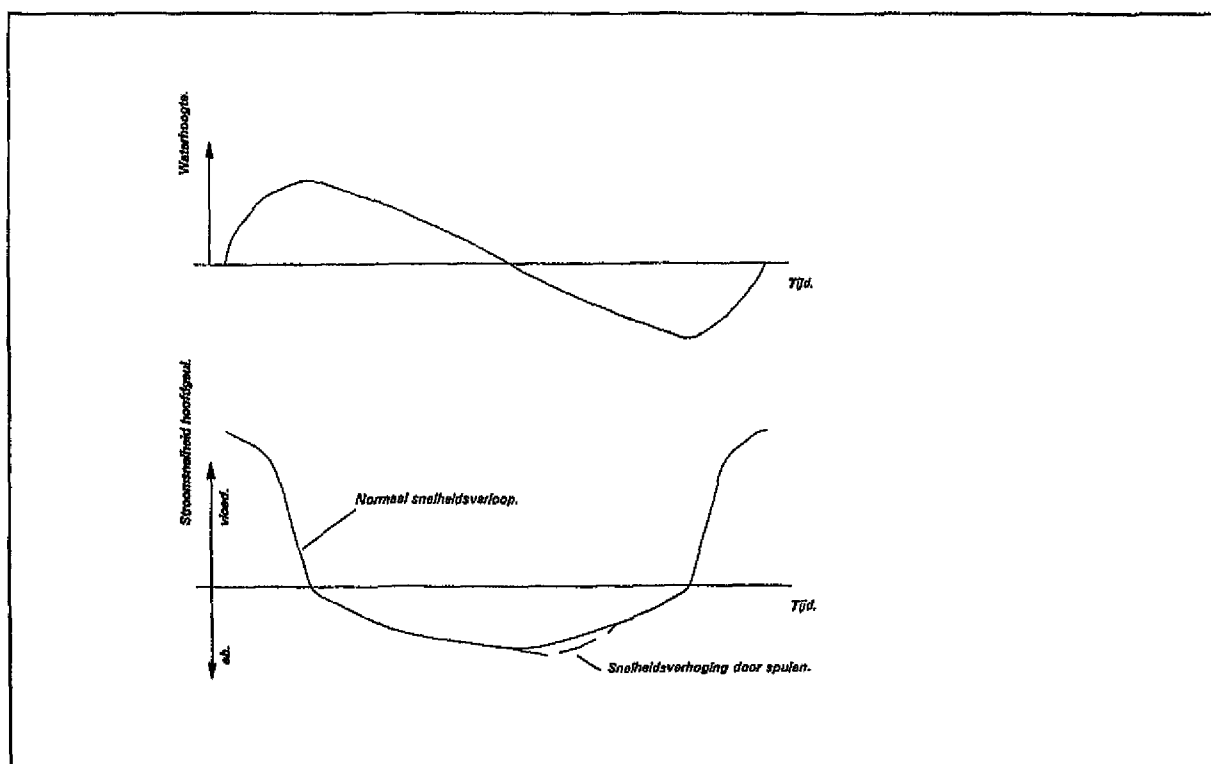
Figuur 2.4.: Invloed van een spuiком op het snelheidsverloop in de hoofdgeul.
