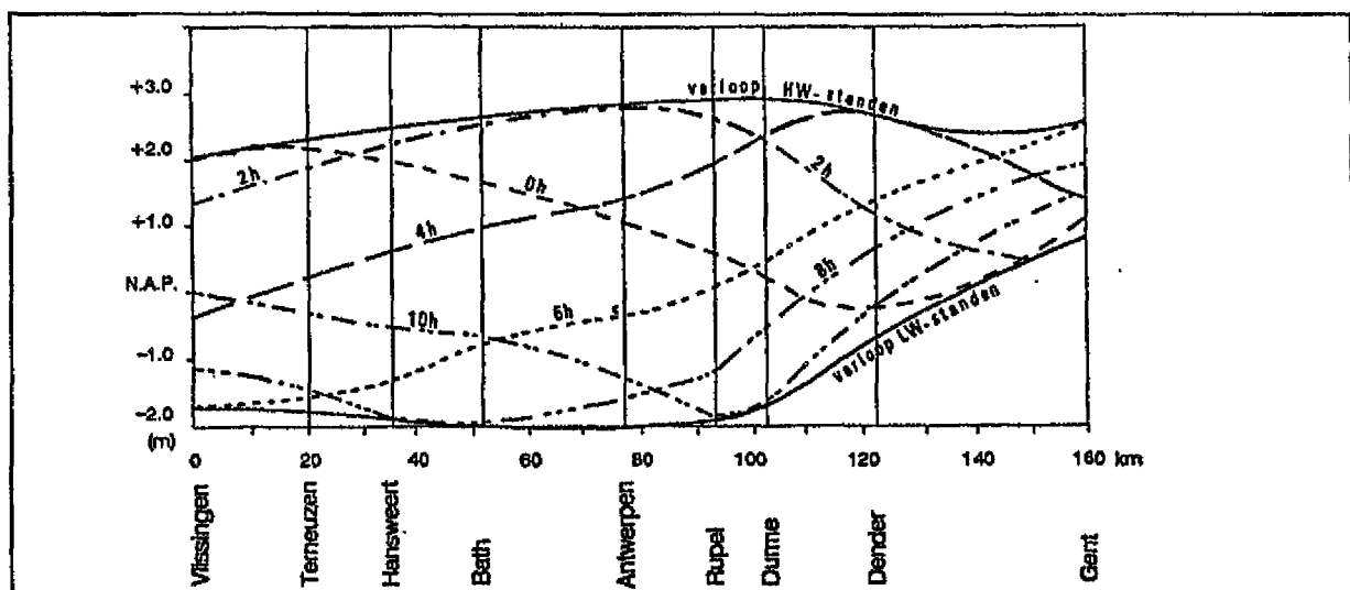
Figuur 1.3.: Verloop waterstanden over de Westerschelde [Pieters et al., 1991].
