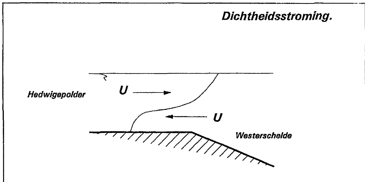
Figuur 3.9.: Dichtheidsstroming.
