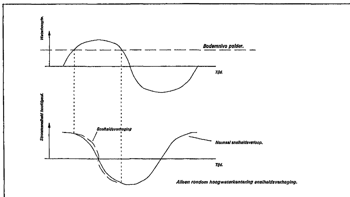
Figuur 2.3.b.: Snelheidsverloop in de hoofdgeul voor de polder bij een hoge bodemligging van de polder.
