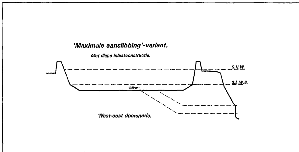
Figuur 4.5.: Inrichting ten behoeve van maximale sedimentatie met afsluitbare diepe inlaat.
