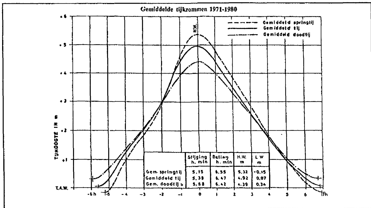
Figuur 1.9.: Gemiddelde waterstandskromme voor de Hedwigepolder (Prosperpolder), [Claessens, 1984]. De peilen zijn ten opzichte van T.A.W.-nivo aangegeven (T.A.W. = N.A.P.-2,33 m).
