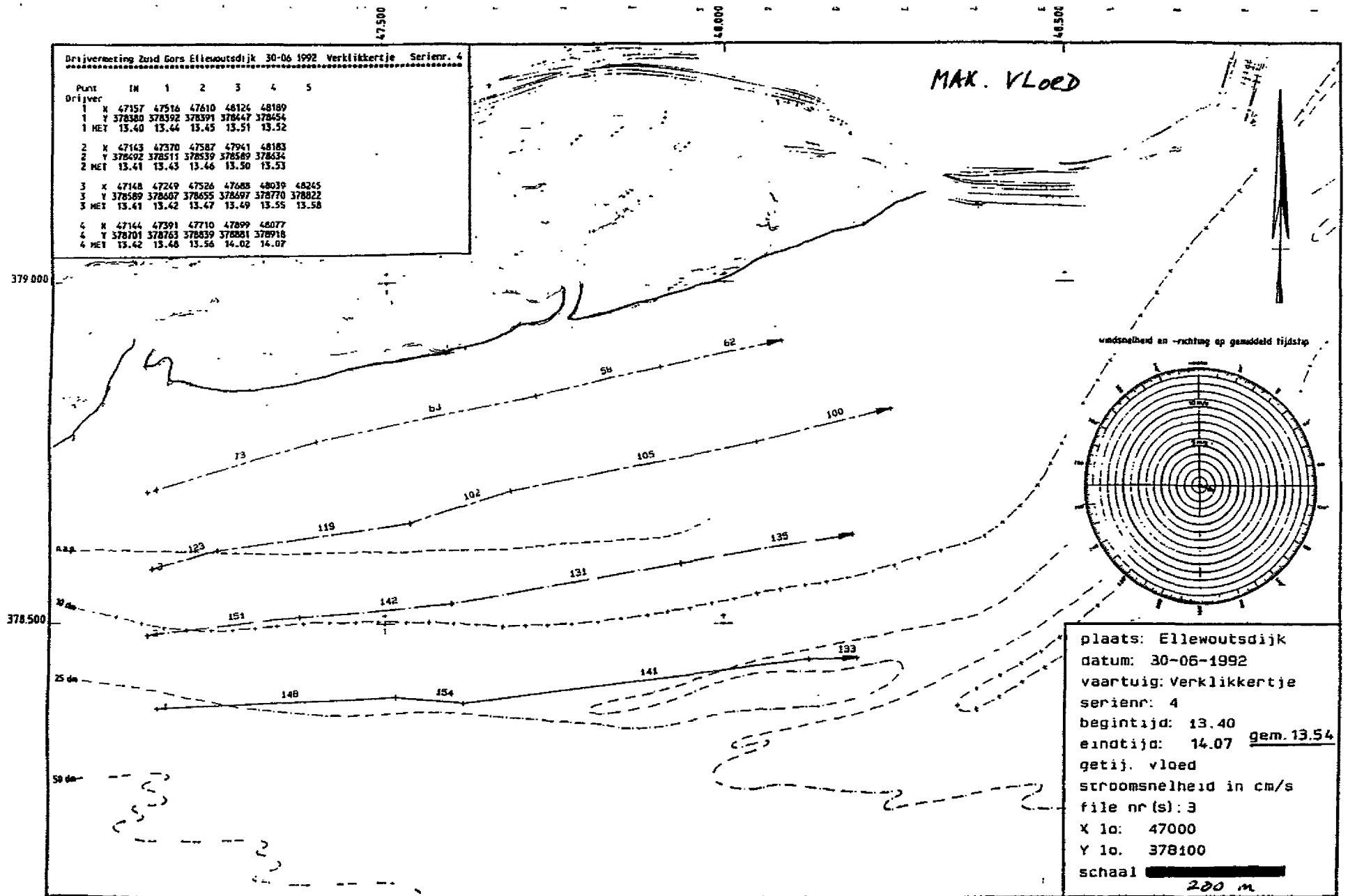
Figuur 4.12 Stroomsnelheden aan het oppervlak bij het Zuidgors tijdens maximum vloed; resultaat drijfvermeting 30 juni 1992.
