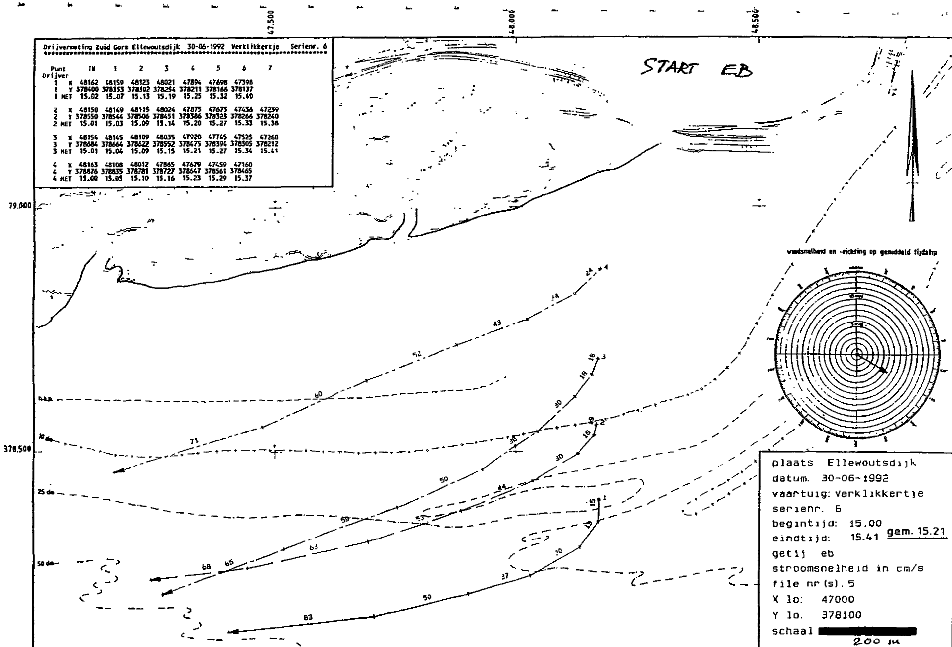
Figuur 4.13 Stroomsnelheden aan het oppervlak bij het Zuidgors tijdens het begin van de eb; resultaat drijvmeting 30 juni 1992.
