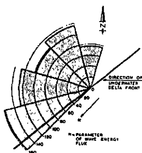
Figuur 3.2: Golfenergie flux voor verschillende richtingen op basis van golfgegevens van het lichtschip Goeree.
