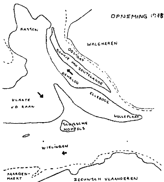
Figuur 5.1: Reststroom in de buitendelta van de Westerschelde volgens De Looff en Verhagen (1986).
