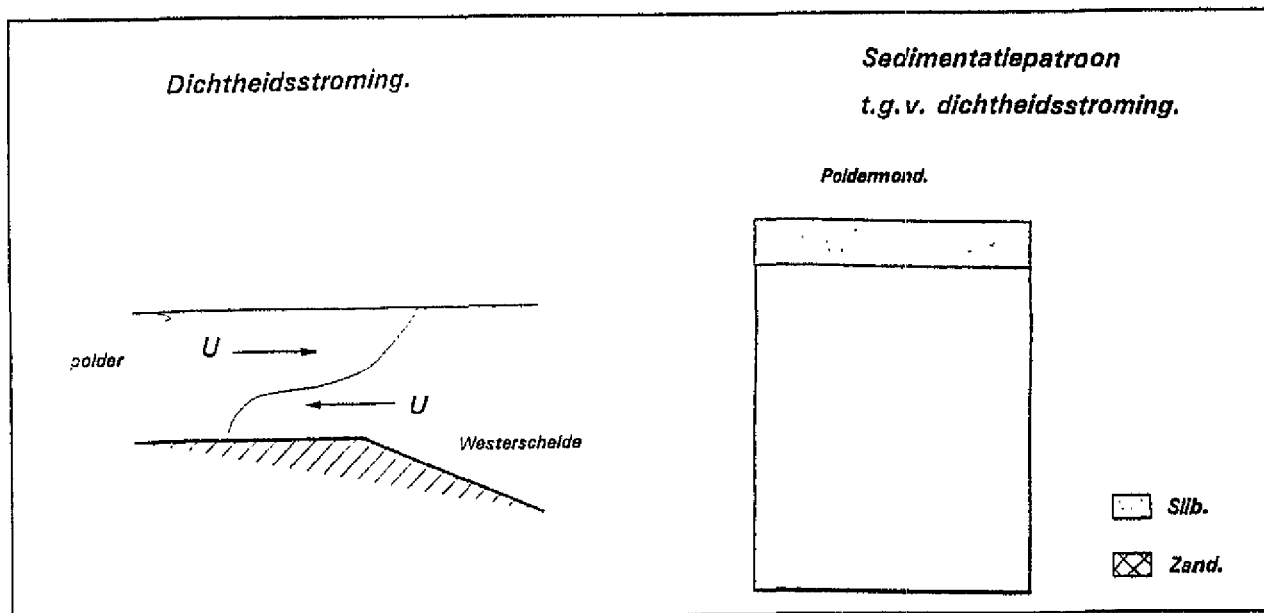
Figuur 5.2 Stromings- en sedimentatiepatroon t.g.v. dichtheidsstroming
