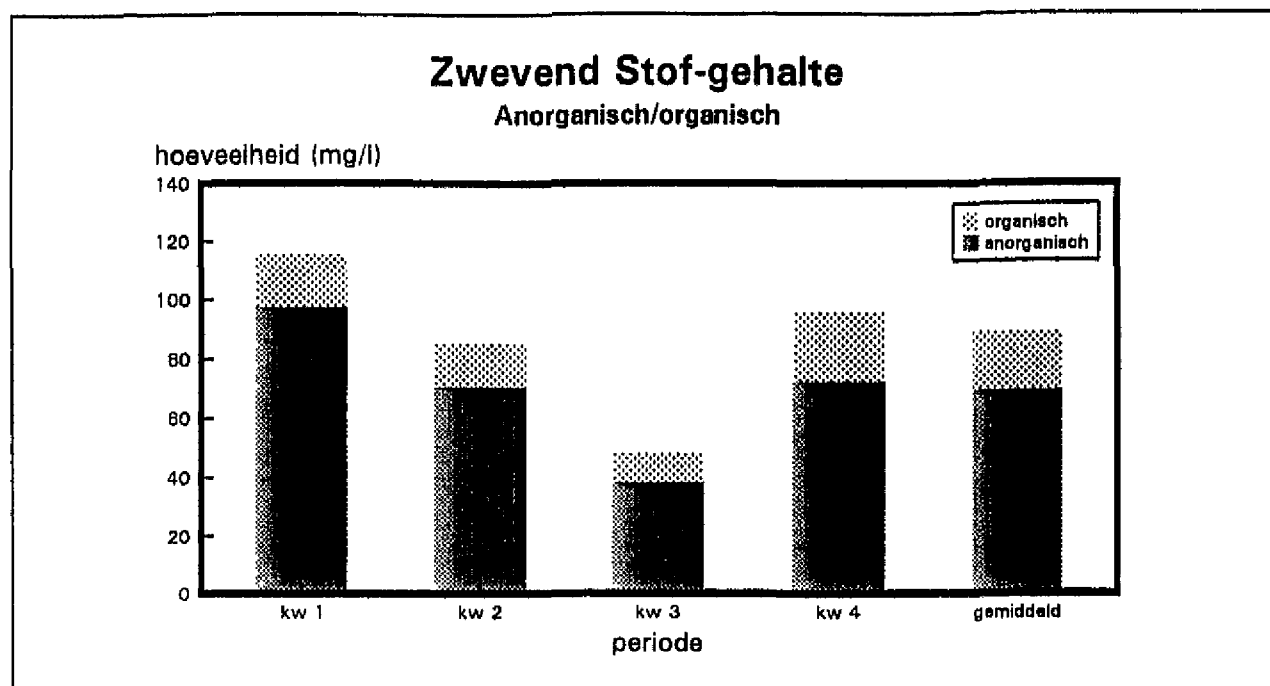
Figuur 2.9 Verdeling van het Zwevend Stof naar anorganisch en organisch materiaal voor de Selenapolder (Schaar van Ouden Doel). Gemiddeldes over de jaren 1987-1991 (DGW, Waterkwaliteitsgegevens)
