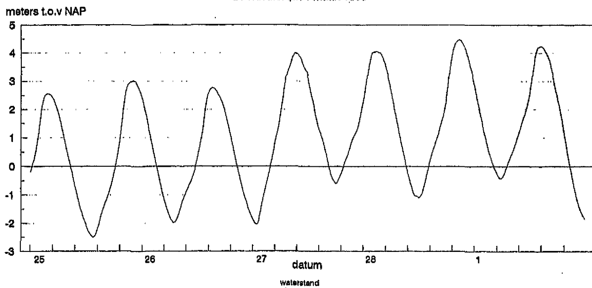
figuur 6.2: Windsnelheden, windrichtingen en waterstanden van 25 februari tot en met 1 maart 1990 (storm 2)
