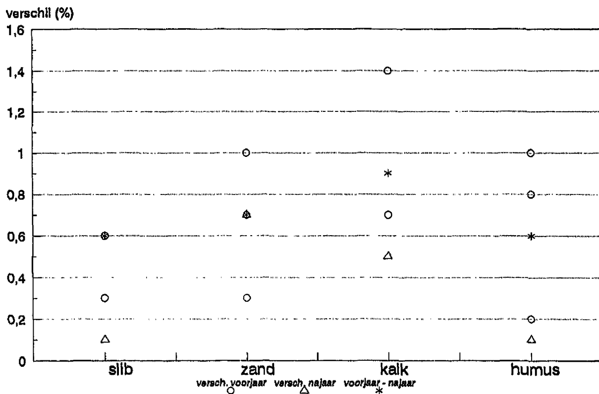
Figuur 5.1: De verschillende gehalten per bodemparameter tussen de voorjaarsmetingen onderling (o) en tussen de najaarsmetingen onderling (driehoekje). En het verschil per parameter tussen alle voorjaarsmetingen en alle najaarsmetingen (*).
