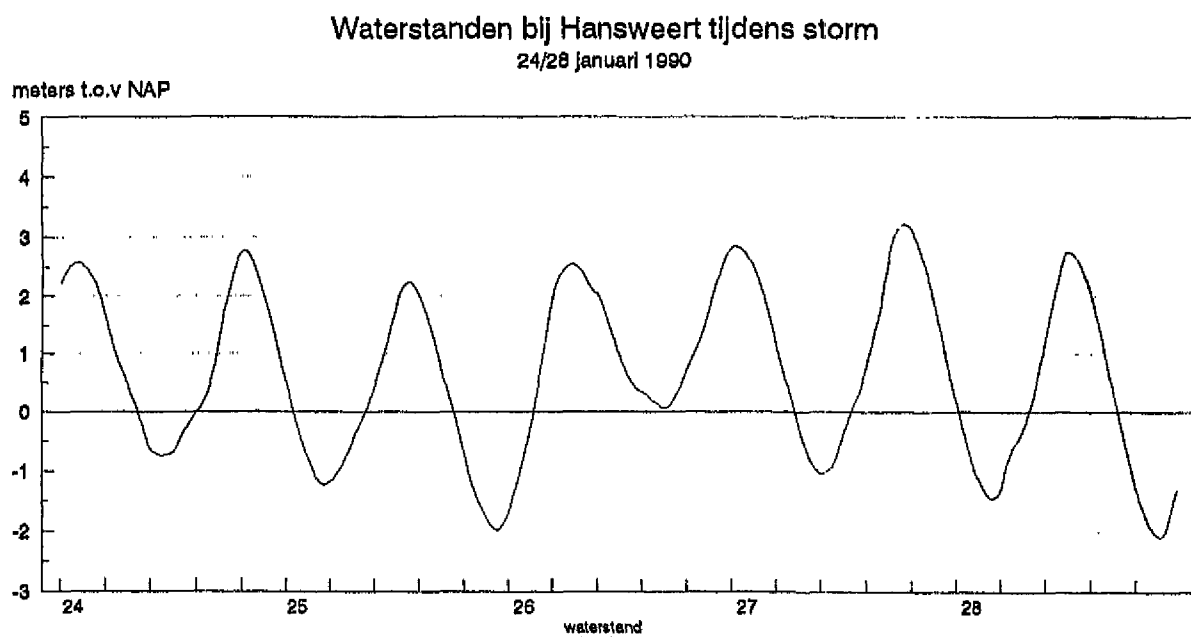
figuur 6.1: Windsnelheden, windrichtingen en waterstanden van 24 tot en met 28 januari 1990 (storm 1)
