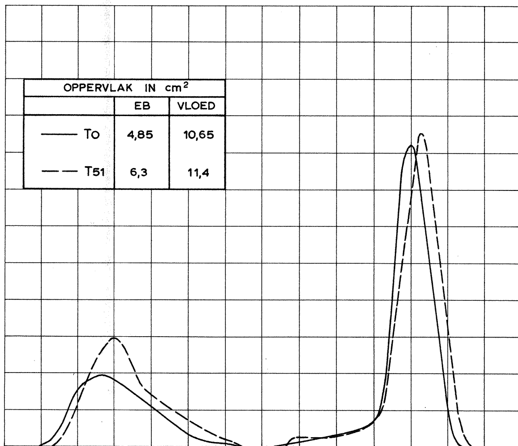
GEM. SNELHEID OPPERVLAKTEDRUVERS IN RAAI DOOR HET SCHAAR VAN WAARDE TUSSEN DIEPTELUNEN N.A.P. -10 m VOLGENS MODELPROEVEN GETJ: SPRINGTJ 4-11-1967
