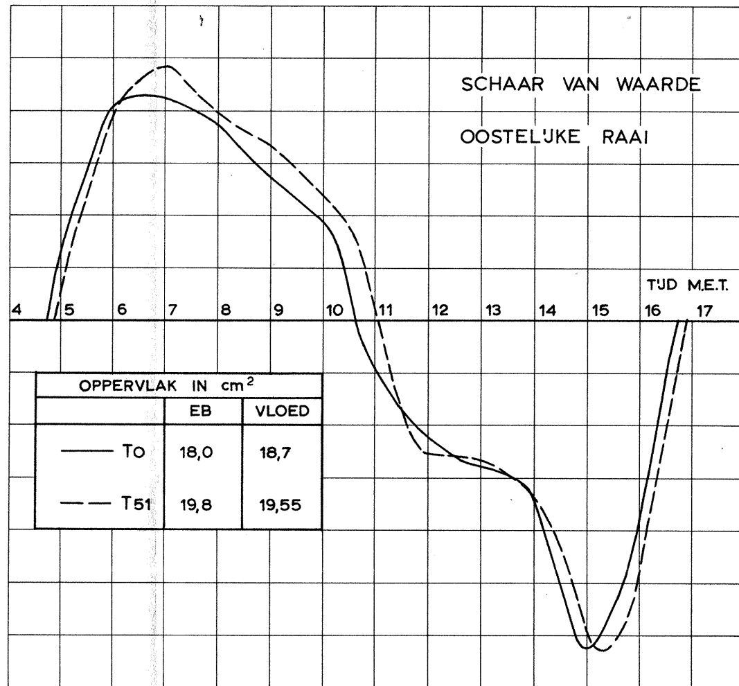
GEM. SNELHEID OPPERVLAKTEDRUVERS IN RAAI DOOR HET SCHAAR VAN WAARDE TUSSEN DIEPTELUNEN N.A.P. -10 m VOLGENS MODELPROEVEN GETJ: SPRINGTJ 4-11-1967
