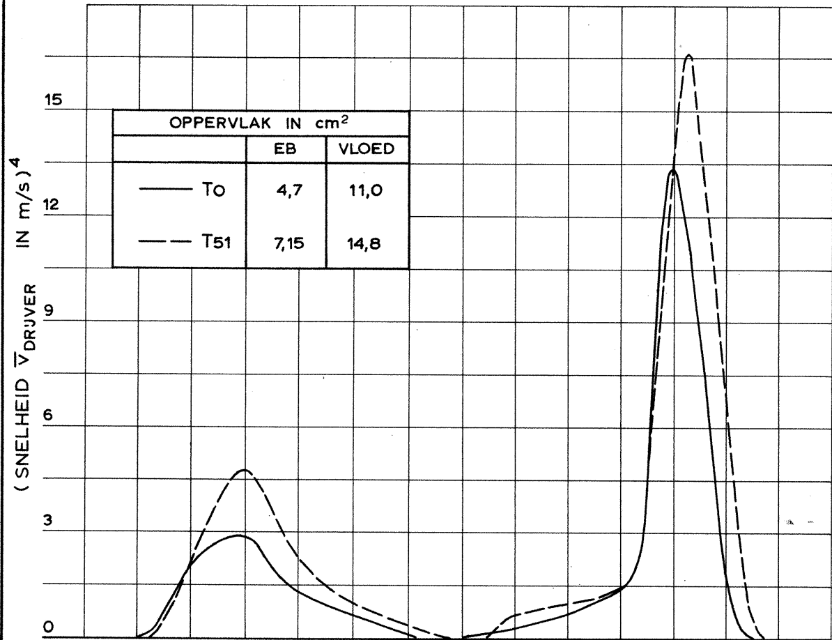
GEM. SNELHEID OPPERVLAKTEDRUVERS IN RAAI DOOR HET SCHAAR VAN WAARDE TUSSEN DIEPTELUNEN N.A.P. -10 m VOLGENS MODELPROEVEN GETJ: SPRINGTJ 4-11-1967
