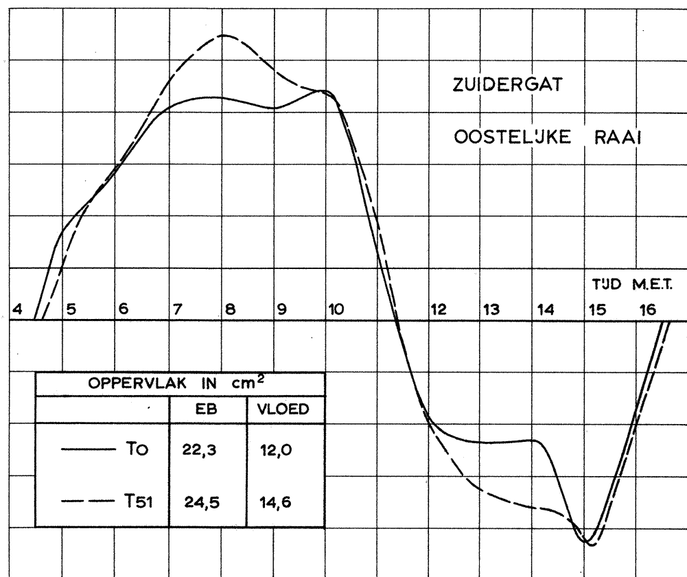
GEM. SNELHEID OPPERVLAKTEDRUVERS IN RAAI DOOR HET ZUIDERGAT TUSSEN DIEPTELUNEN N.A.P. -10 m VOLGENS MODELPROEVEN GETJ: SPRINGTJ 4-11-1967
