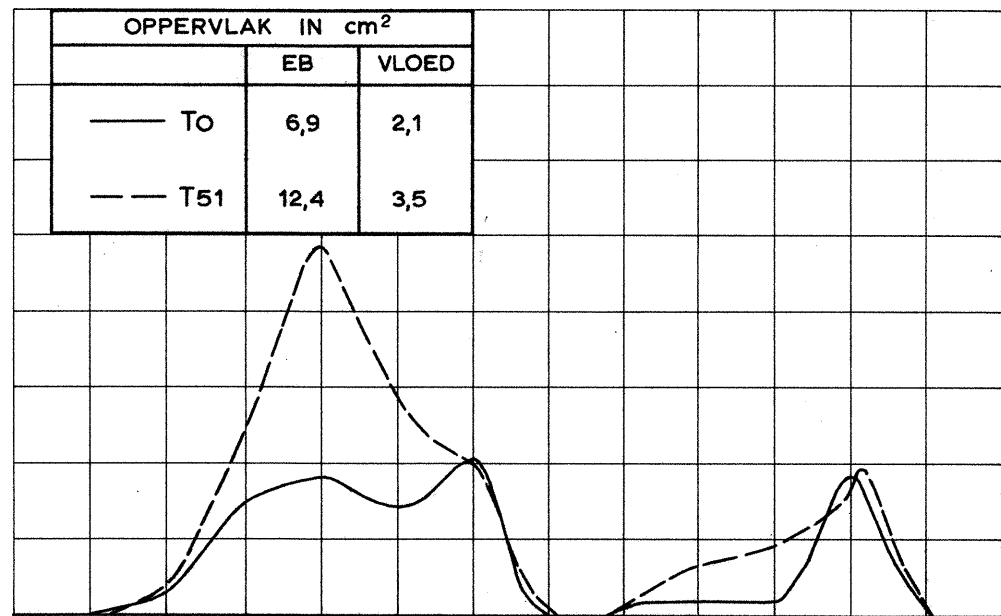
GEM. SNELHEID OPPERVLAKTEDRUVERS IN RAAI DOOR HET ZUIDERGAT TUSSEN DIEPTELUNEN N.A.P. -10 m VOLGENS MODELPROEVEN GETJ: SPRINGTJ 4-11-1967
