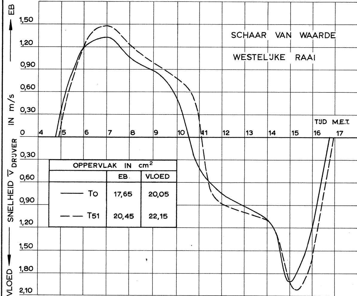
GEM. SNELHEID OPPERVLAKTEDRUVERS IN RAAI DOOR HET SCHAAR VAN WAARDE TUSSEN DIEPTELUNEN N.A.P. -10 m VOLGENS MODELPROEVEN GETJ: SPRINGTJ 4-11-1967
