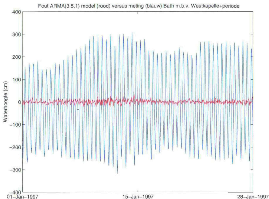
Figuur 2.15: Waargenomen waterstand in Bath en fout in voorspelling op basis van 15 periodiciteiten en de waterstand in Westkapelle
