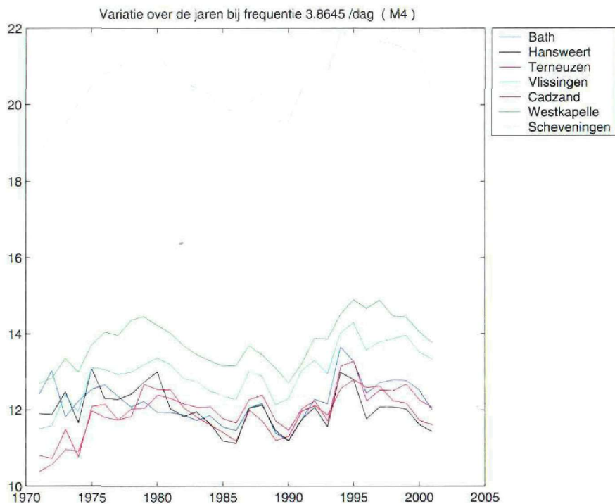
Figuur 2.12: Amplitudeverloop van het M4-getij
