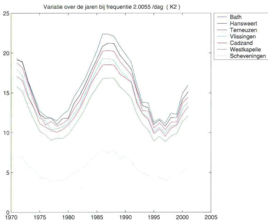
Figuur 2.5: Amplitudeverloop van het K2-getij
