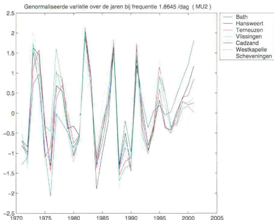
Figuur 2.11: Relatief amplitudeverloop van het MU2-getij
