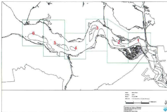
Figuur 3.1: Onderverdeling van de Westerschelde in 6 vakken
