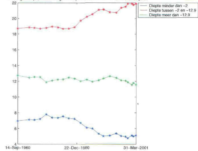
Omvang ondiepe, middelmatige en diepe stukken in Mm 2 in vak 4 over de jaren
