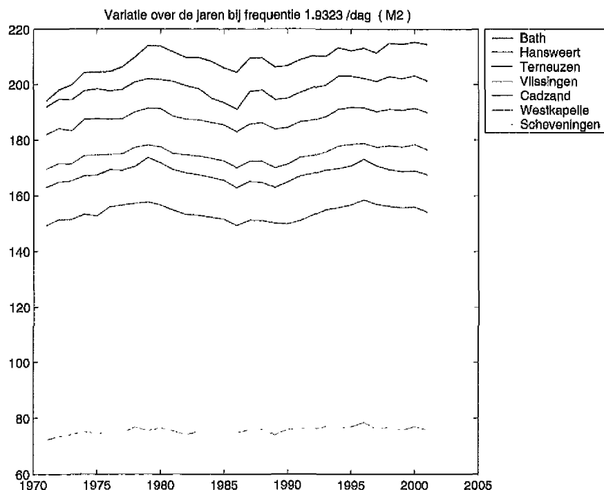
Figuur 2.3: Amplitudeverloop van het M2-getij
