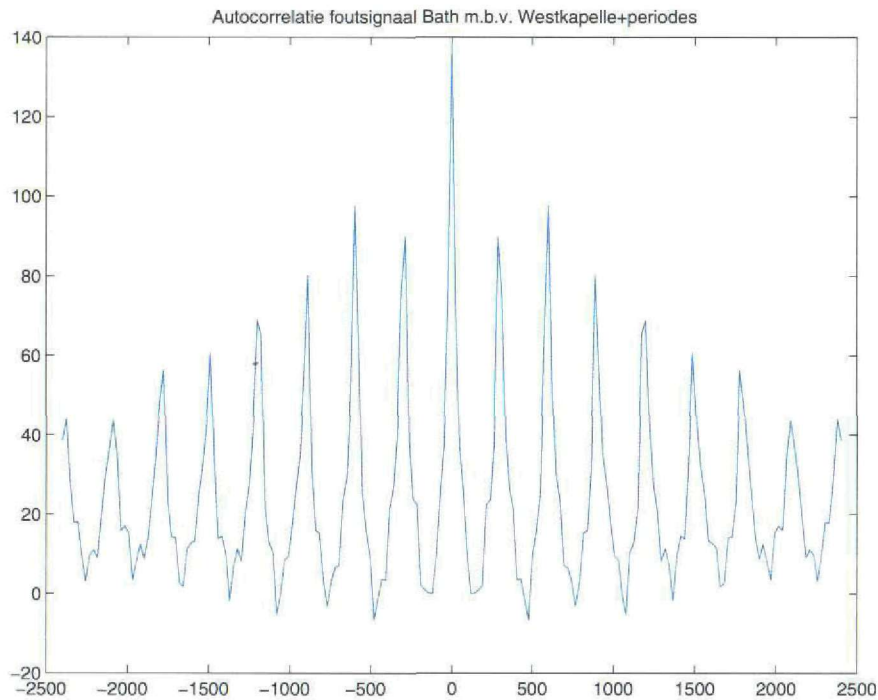
Figuur 2.16: Autocorrelatie foutsignaal in Bath op basis van 15 periodiciteiten en de waterstand in Westkapelle
