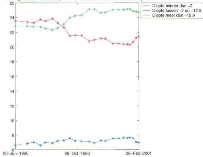
Omvang ondiepe, middelmatige en diepe stukken in Mm 2 in vak 5 over de jaren
