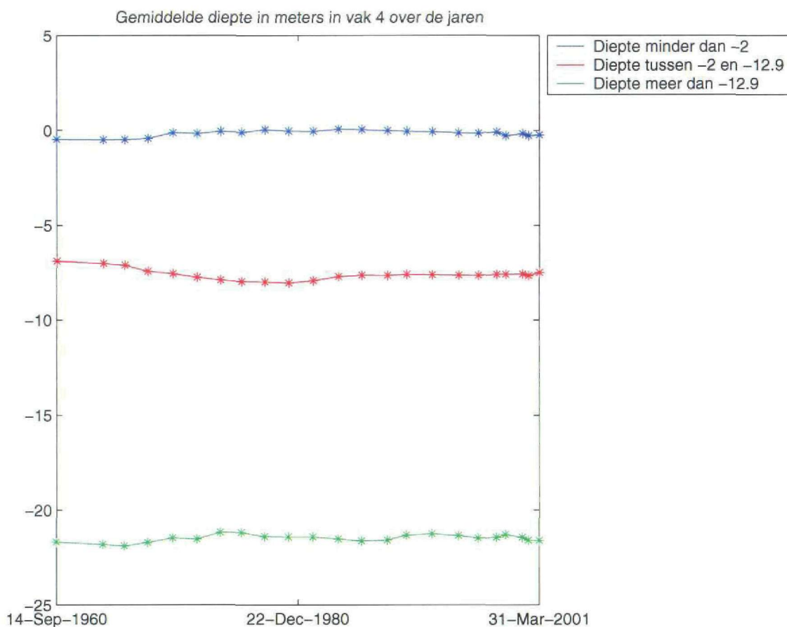
Figuur 3.4: Gemiddelde diepte t.o.v. NAP van ondiepe, middelmatige diepe en diepe gebieden in de Westerschelde binnen vak 4.
