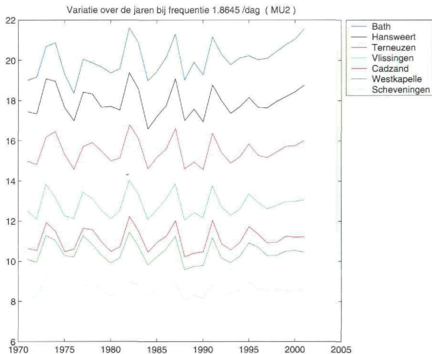
Figuur 2.10: Amplitudeverloop van het MU2-getij
