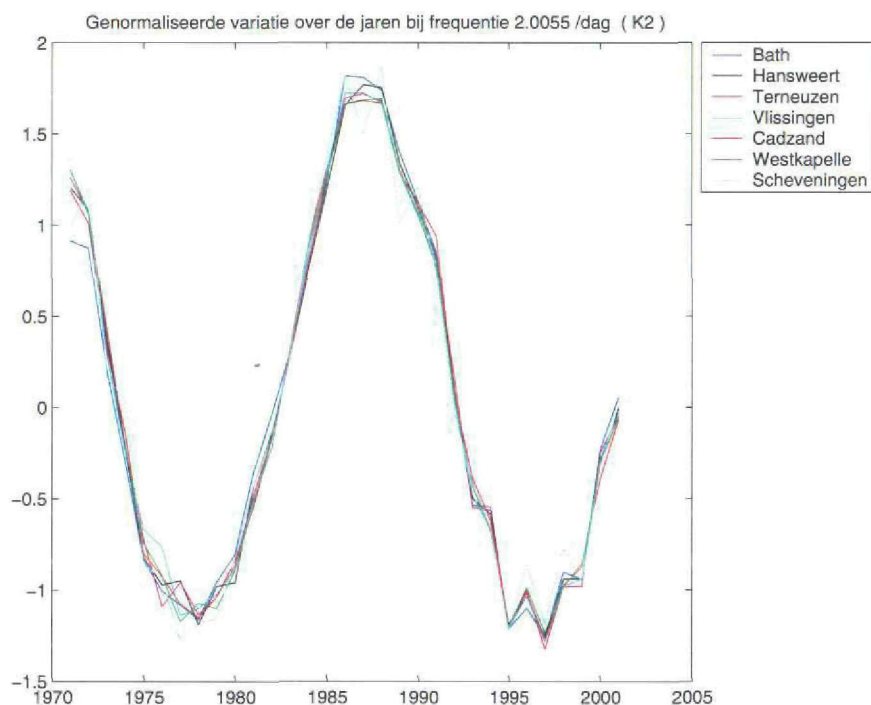
Figuur 2.6: Relatief amplitudeverloop van het K2-getij
