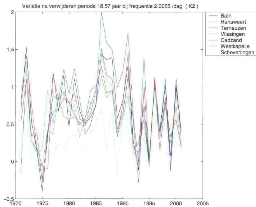
Figuur 2.7: Amplitudeverloop van het K2-getij na verwijdering periodiciteit
