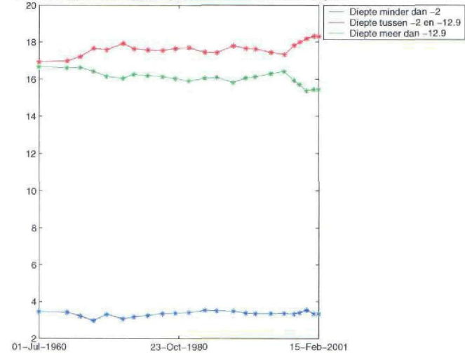
Omvang ondiepe, middelmatige en diepe stukken in Mm 2 in vak 6 over de jaren
