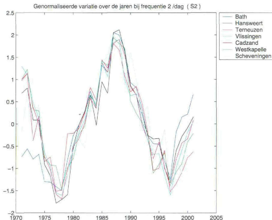
Figuur 2.9: Relatief amplitudeverloop van het S2-getij
