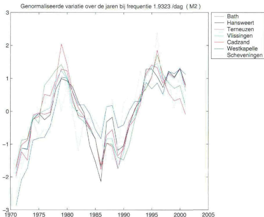
Figuur 2.4: Relatief amplitudeverloop van het M2-getij
