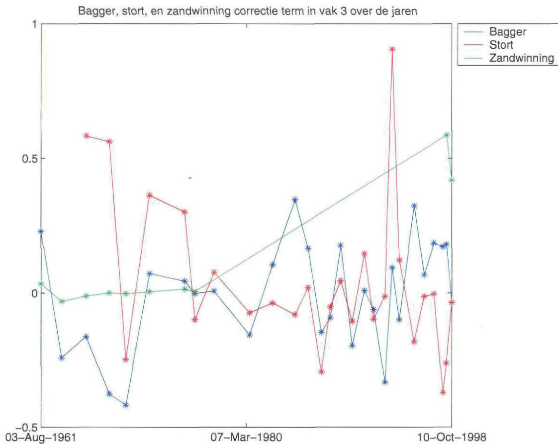
Figuur 3.3: Correctiewaarden voor effecten bagger, stort en zandwinningen op de diepte van de Westerschelde binnen vak 3
