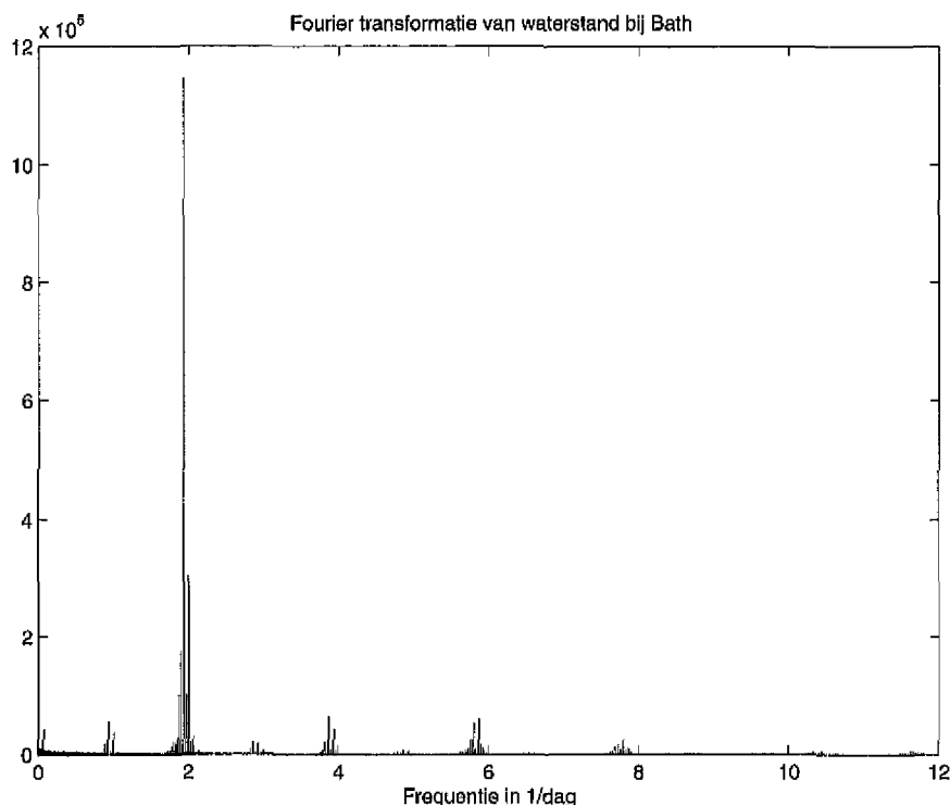
Figuur 2.1: Fouriergetransformeerde van de eenmaal per uur gemeten waterstand in Bath
