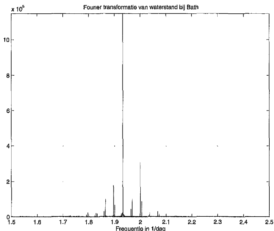
Figuur 2.2: Fouriergetransformeerde van de eenmaal per uur gemeten waterstand in Bath (detail)
