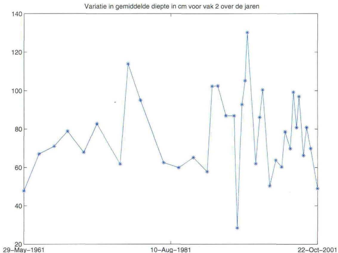
Figuur 3.2: Gemiddelde verandering per jaar in cm van de diepte van de Westerschelde binnen vak 2
