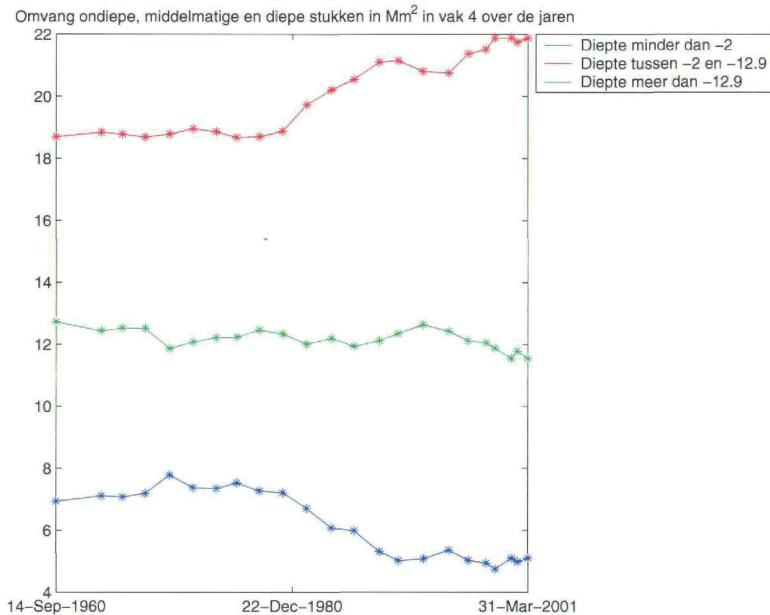
Figuur 3.5: Omvang van ondiepe, middelmatige diepe en diepe gebieden in de Westerschelde binnen vak 4
