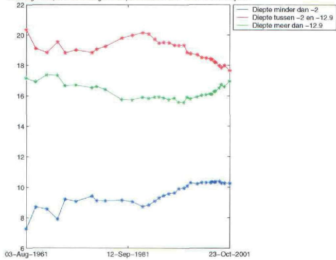
Omvang ondiepe, middelmatige en diepe stukken in Mm 2 in vak 3 over de jaren
