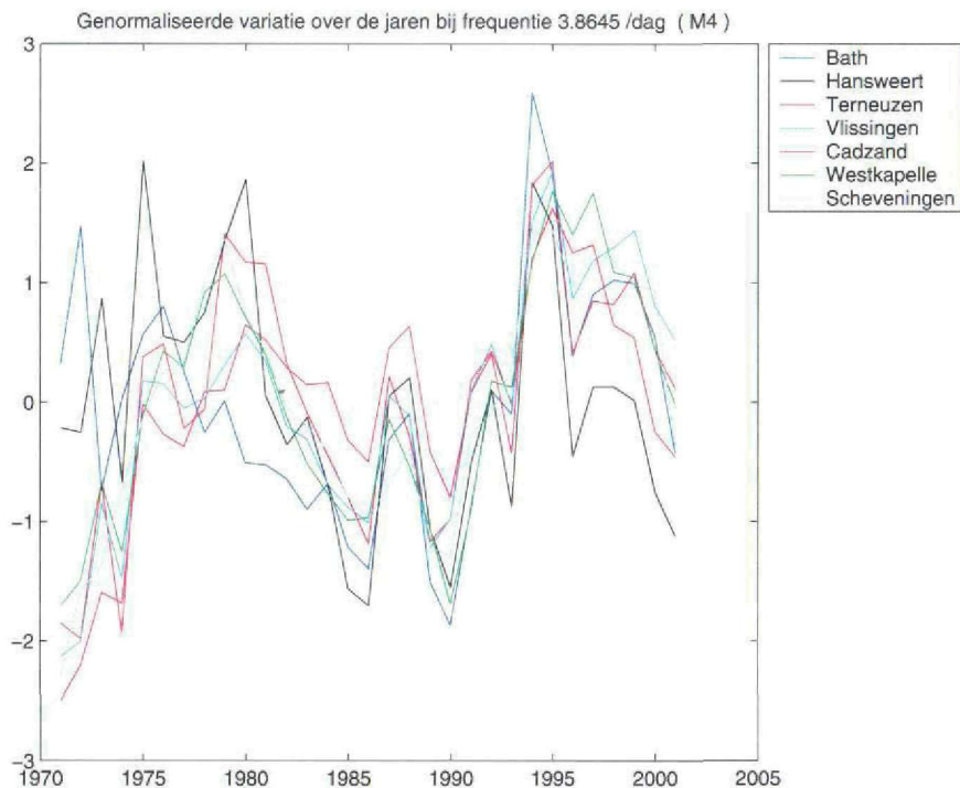
Figuur 2.13: Relatief amplitudeverloop van het M4-getij
