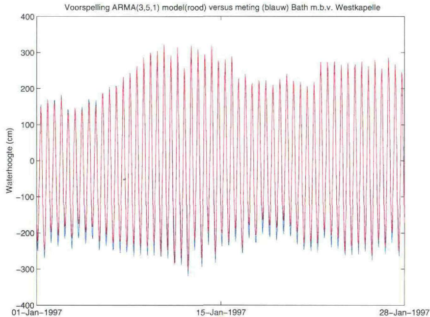
Figuur 2.14: Voorspelling van de waterstand in Bath op basis van de waterstand in Westkapelle m.b.v. een ARMA (3, 5, 1)-model
