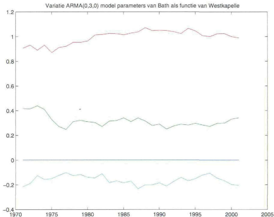
Figuur 2.17: Tijdsverloop parameters in MA (0, 3, 0)-model voor voorspelling van het restsignaal in Bath op basis van het restsignaal in Westkapelle
