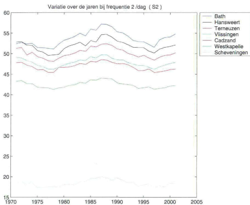
Figuur 2.8: Amplitudeverloop van het S2-getij
