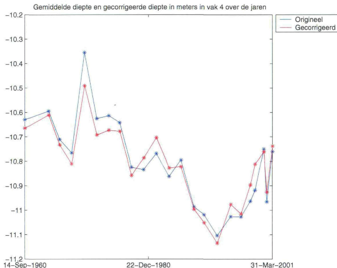
Figuur 3.6: Gemiddelde diepte en gecorrigeerde diepte binnen vak 4
