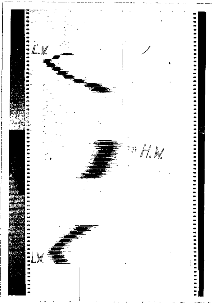
Afb. 5: Registratie golf- amplitudeschrijver (Wemelsfelder)
