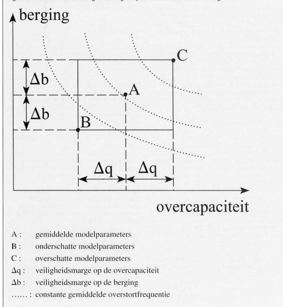
Figuur 6: inrekenen van de veiligheidsmarges bij de selectie van korte neerslagreeksen.
