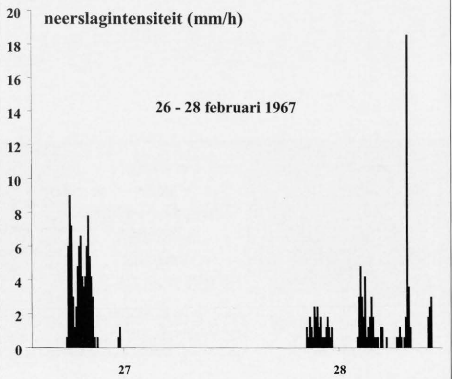
Figuur 1: voorbeeld van een korte neerslagreeks.
