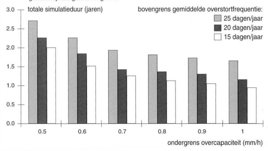
Figuur 4: invloed op de totale simulatieduur vanwege de minimale overcapaciteit en de maximale overstortfrequentie voor een veralgemeende set van korte neerslagreeksen (de andere grenzen zijn aangeduid in figuur 3).
