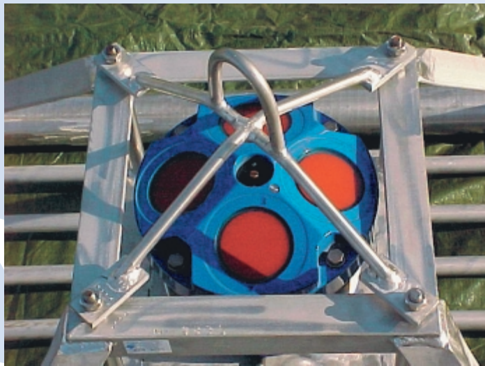
ACME-meettoestel
