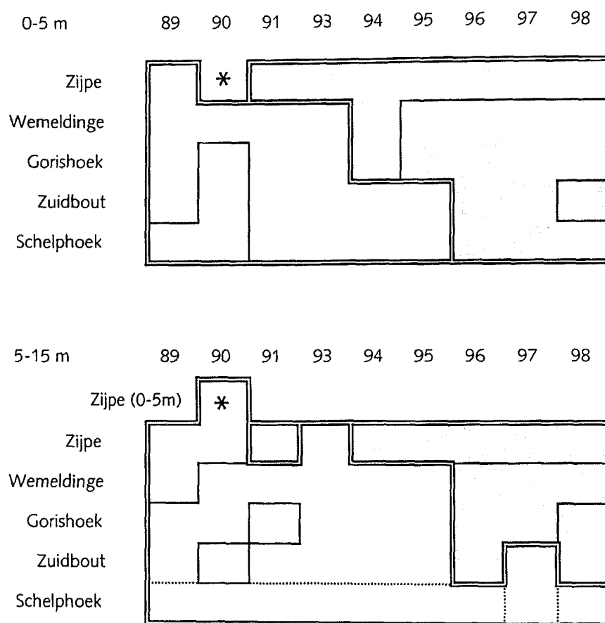
Fig. 3. Overzicht TWINSpan analyse Oosterschelde, periode 1989-'98: maximale bedekkingen in de zone 0-5 m (boven) en 5-15 m (onder). Dubbele lijnen onderscheiden clusters op het eerste niveau. Enkele en onderbroken lijnen clusters op het tweede, respectievelijk derde niveau.
