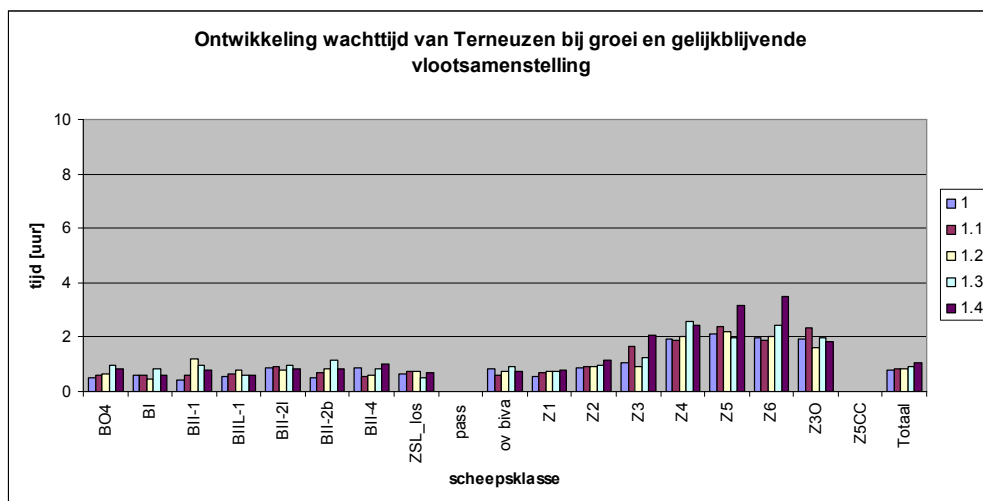
Figuur 12.8 – Gelijkblijvende vlootsamenstelling – wachttijd van Terneuzen
