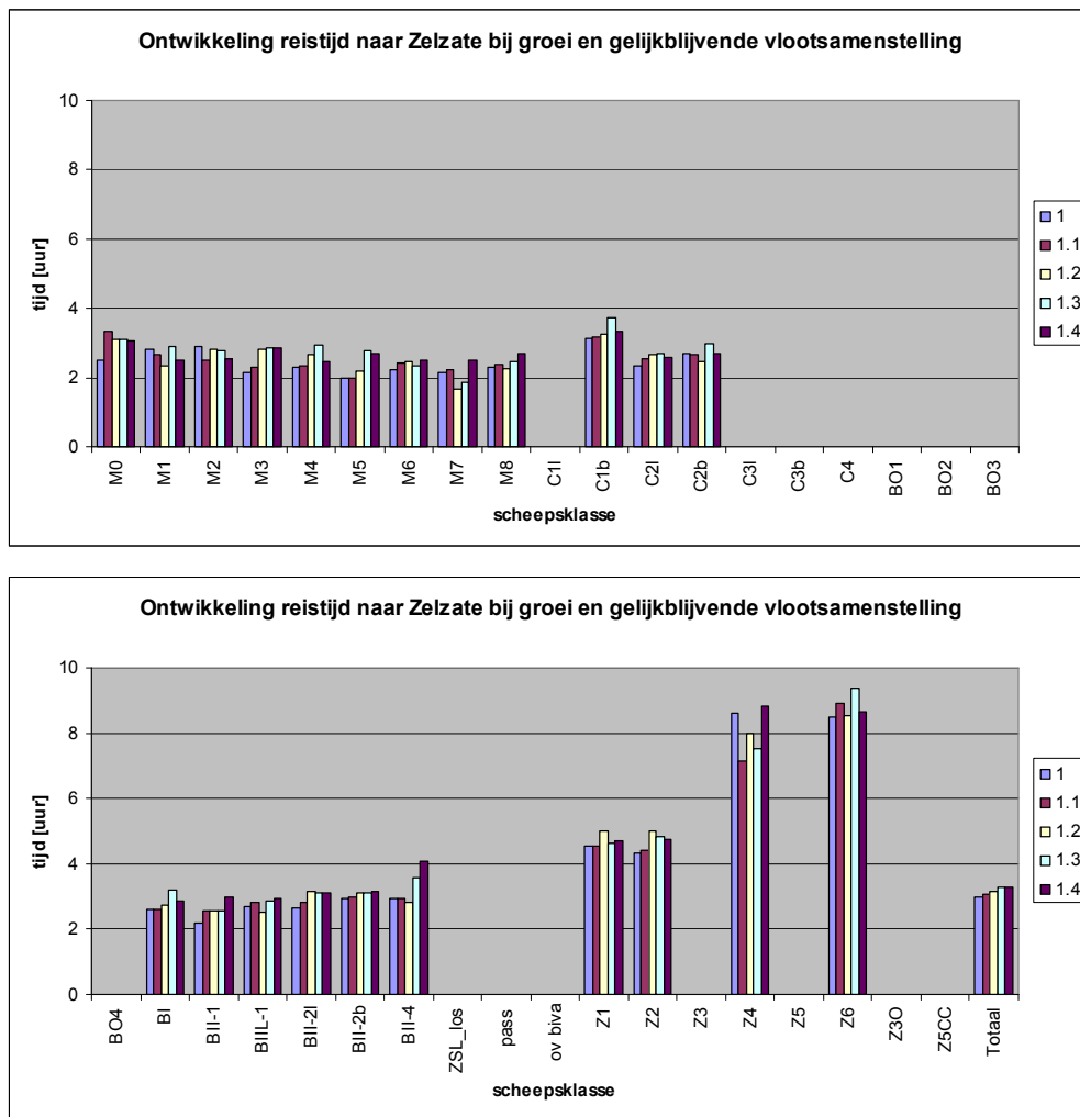
Figuur 12.16 – Gelijkblijvende vlootsamenstelling – reistijd naar Zelzate
