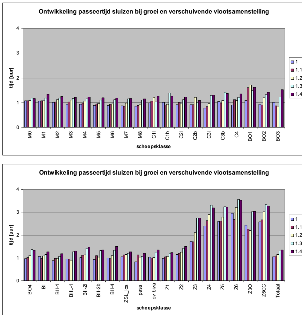
Figuur 7.4 – Verschuivende vlootsamenstelling – passeertijd sluizen
