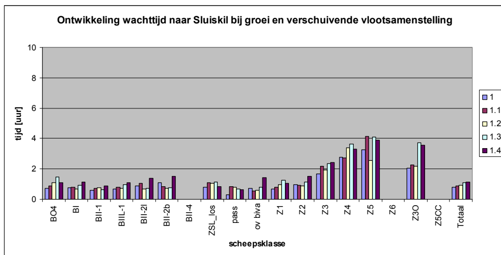
Figuur 13.11 – Verschuivende vlootsamenstelling – wachttijd naar Sluiskil
