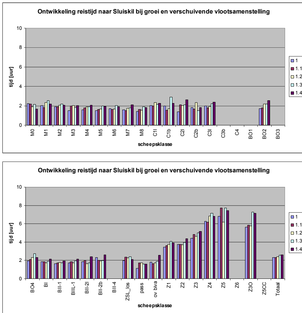
Figuur 13.10 – Verschuivende vlootsamenstelling – reistijd naar Sluiskil
