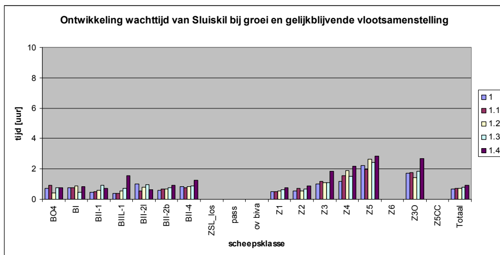
Figuur 12.14 – Gelijkblijvende vlootsamenstelling – wachttijd van Sluiskil
