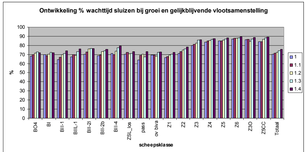
Figuur 12.3 – Gelijkblijvende vlootsamenstelling – percentage wachttijd sluizen
