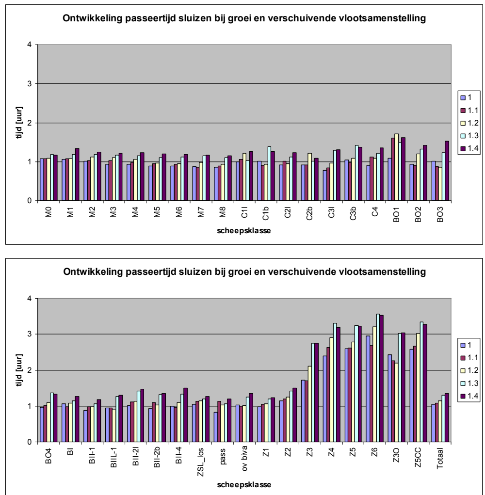
Figuur 13.1 – Verschuivende vlootsamenstelling – passeertijd sluizen
