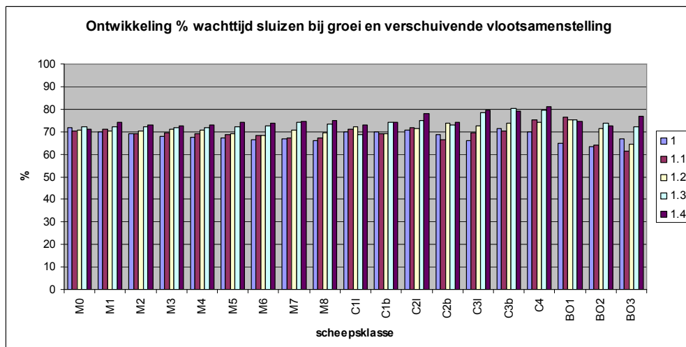
Figuur 13.2 – Verschuivende vlootsamenstelling – wachttijd sluizen
