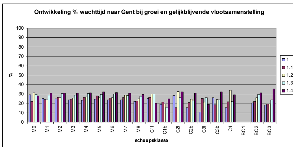
Figuur 12.23 – Gelijkblijvende vlootsamenstelling – wachttijd naar Gent
