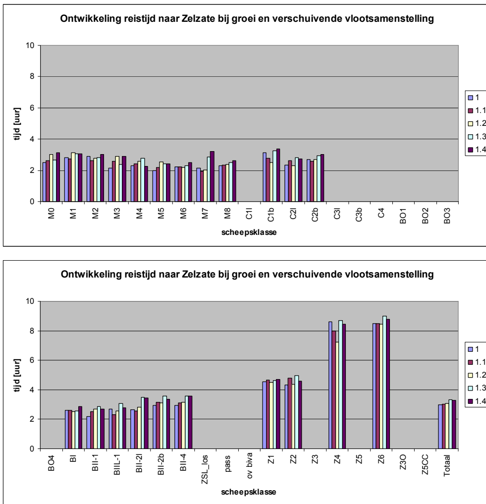
Figuur 13.16 – Verschuivende vlootsamenstelling – reistijd naar Zelzate
