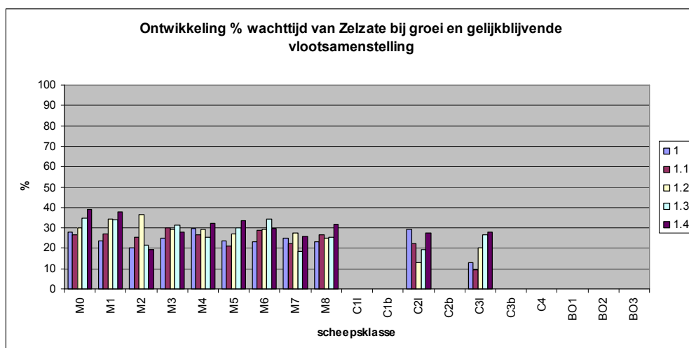
Figuur 12.20 – Gelijkblijvende vlootsamenstelling – wachttijd van Zelzate
