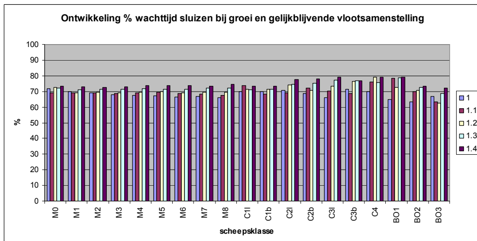
Figuur 7.2 – Gelijkblijvende vlootsamenstelling – wachttijd sluizen
