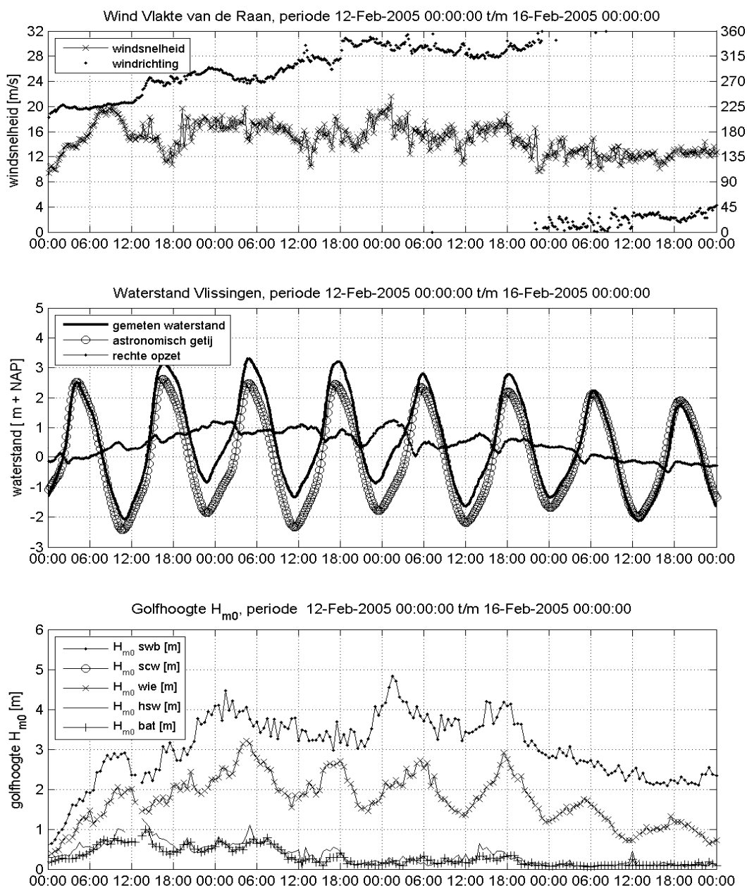
Figuur 6.6: Tijdseries van de wind-, waterstandmetingen en golfparameter H_{m0} voor de periode 12-2-2005 12:00 tot 16-2-2005.
