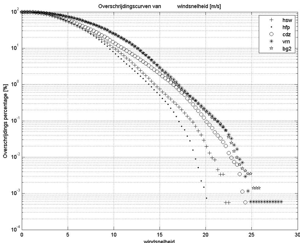
Figuur 5.2: Overschrijdingscurven van de windsnelheid op de windmeetlocaties.
