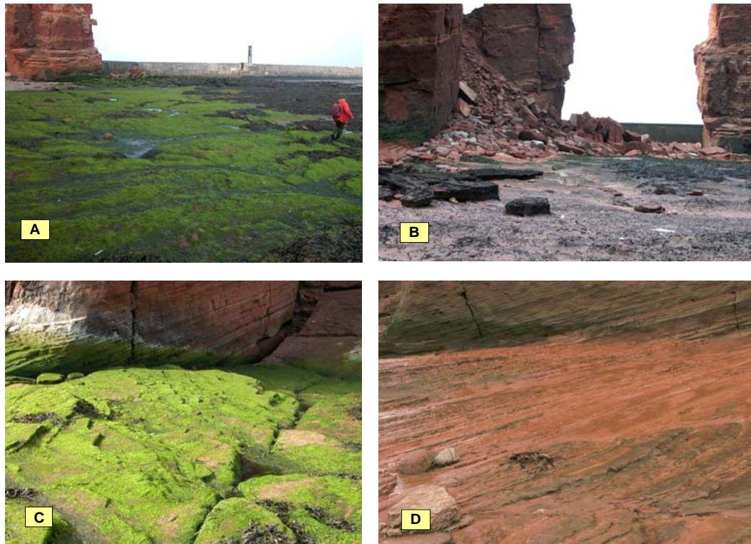
Abb. 14: Veränderung der Enteromorpha -Flächen im westlichen Teil des oberen Eulitorals zwischen 2005 und Februar 2007. Fotos: R. Kühlenkamp A: Juli 2005; Dichte Bedeckung im Enteromorpha -Polygon mit Enteromorpha . B: Februar 2007; Dasselbe Gebiet wie A mit neuem Geröllfeld durch Felsabsturz und sehr geringem Enteromorpha -Bewuchs. C: Juli 2005; Dichter Enteromorpha -Bewuchs bis an die senkrechte Felskante D: Dez 2006; Gleiches Gebiet wie in C mit fast unbewachsenem Substratum durch Geröllabrieb (veränderter Blickwinkel wodurch die Felsspalten nicht zu sehen sind).
