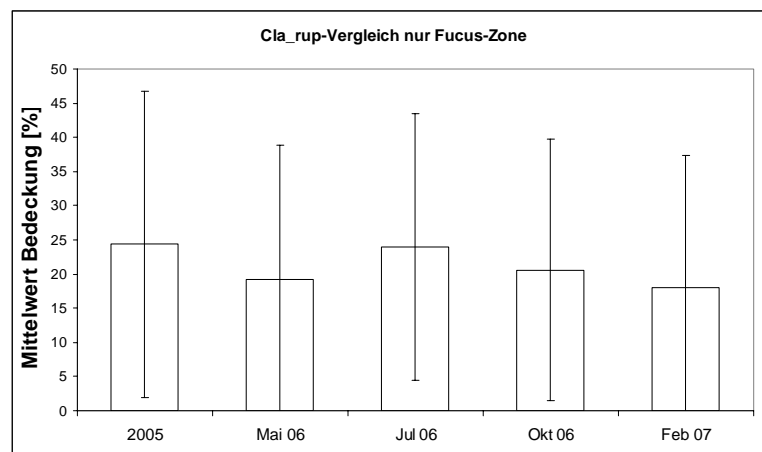
Abb. 10: Cladophora rupestris : Mittelwerte der Bedeckung aller Quadrate in der dichten Fucus -Zone zum jeweiligen Probennahmezeitpunkt und Standardabweichung.
