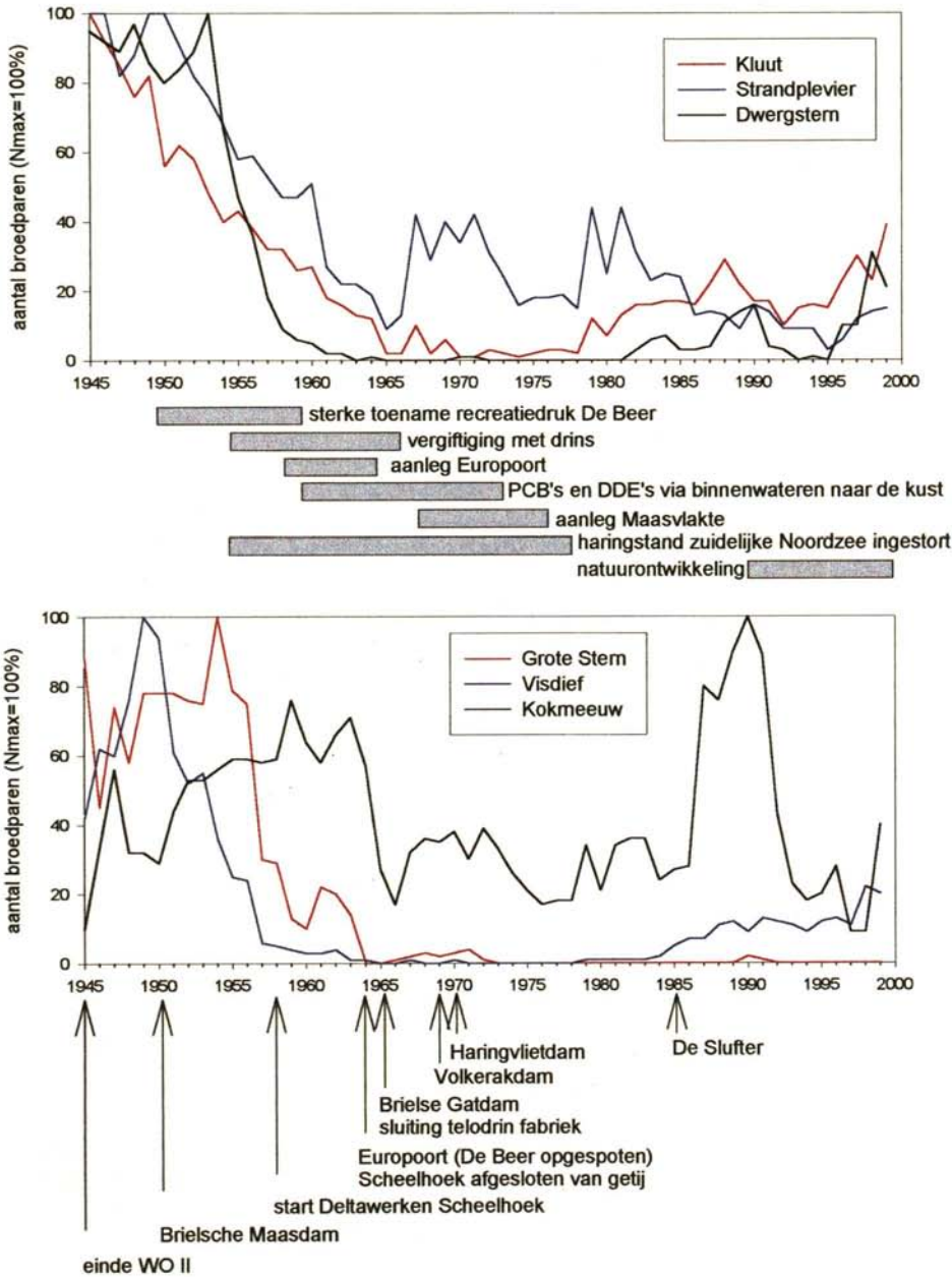
Figuur 32 Trends van de belangrijkste kustbroedvogels in de periode 1945-2000, alsmede de belangrijkste factoren die (wellicht) een rol hebben gespeeld bij de populatieontwikkeling.
