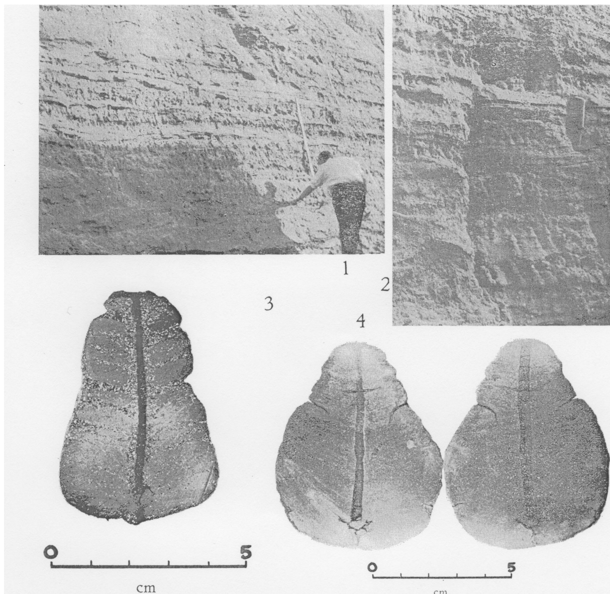
Foto's 1 en 2. Doorsneden in de Ordampolder, tijdens de graafwerken van het kanaaldok. Verscheidene lagen met overvloedige konkreties zijn zichtbaar in het pleistoceen zand.
