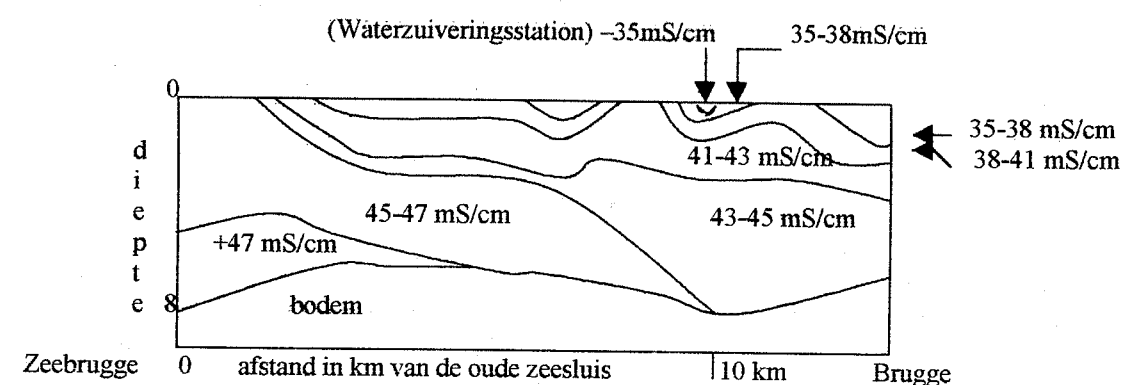
Fig. 3 : Profiel van het geleidingsvermogen in het Boudewijnkanaal (dec 1990, VMM, 1992)
