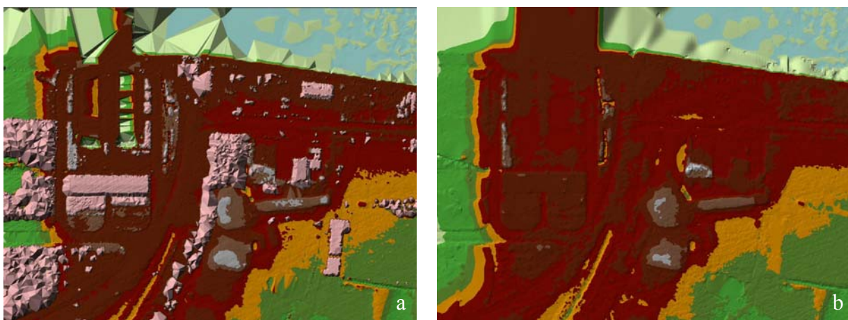
Figuur 51. a) Ruwe laserscandata vlucht 2007 ter hoogte van het Kallosluis. b) Op niet-maaiveldpunten gefilterde laserscandata van hetzelfde gebied.
