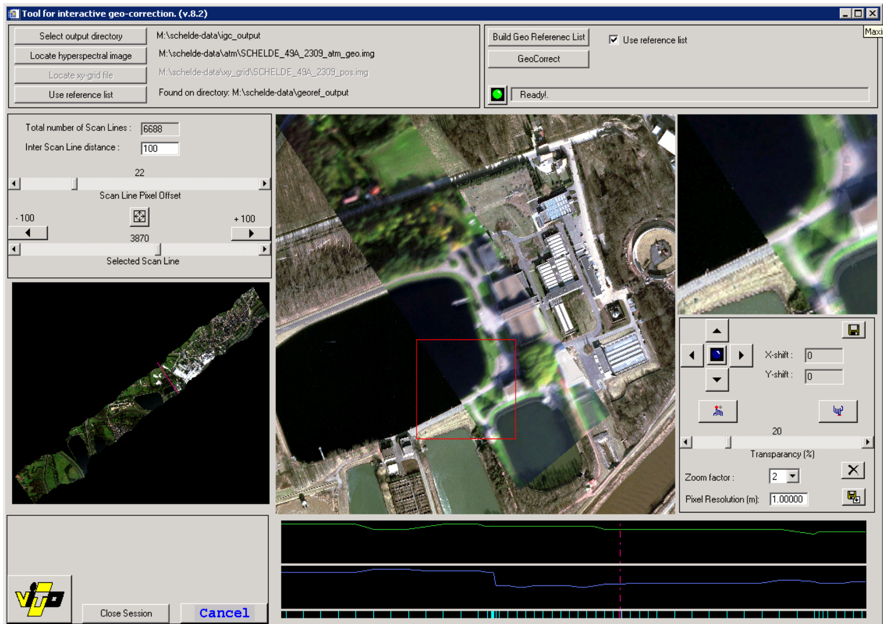
Figuur 54. Software tool voor het manueel interactief geocorrigeren van onnauwkeurig georeferenceerde beelden
