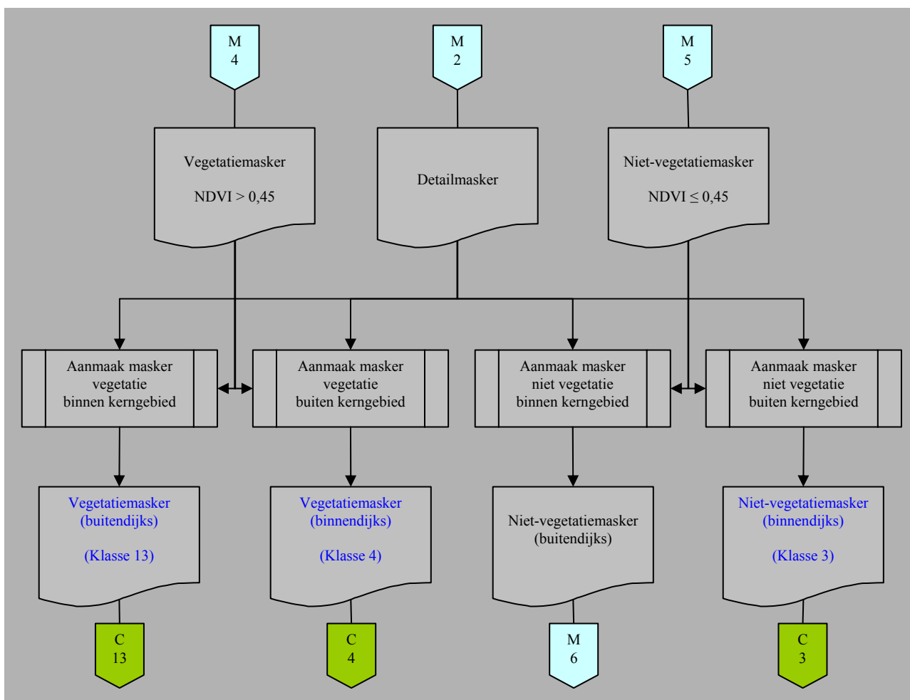
Figuur 15. Schema voor de aanmaak van het binnendijks/buitendijks vegetatie/niet-vegetatiemasker. Gebruik makend van een logische combinatie van het vegetatiemasker (M4), het niet-vegetatiemasker (M5) en het detailmasker (M2) dat het kerngebied afbakt konden de maskers ‘Vegetatie (binnendijks)’ (C4), ‘Niet-vegetatie (binnendijks)’ (C3) en ‘Vegetatie (buitendijks)’ (C13), ‘Niet-vegetatie (buitendijks)’ (M6) aangemaakt worden.
