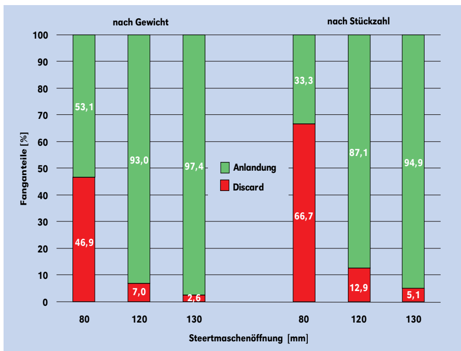
Abbildung 4: Prozentuale, gewichtsmäßige und stückzahlmäßige Anteile von Discard und Markware im Gesamtfang der Schollen bei unterschiedlichen Maschenöffnungen.
