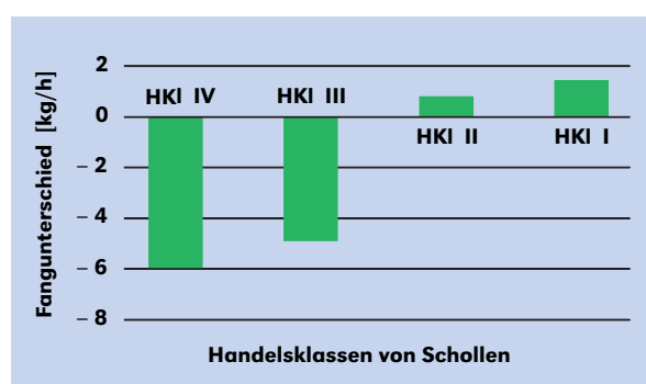
Abbildung 7: Fangverlust pro Schleppstunde des 120 mm Versuchssteertes zum 80 mm Referenzsteert: Aufteilung nach Handelsklassen für Schollen (mittlere Erlöse für Scholle zwischen 1,90 €/kg bis 3,00 €/kg).
