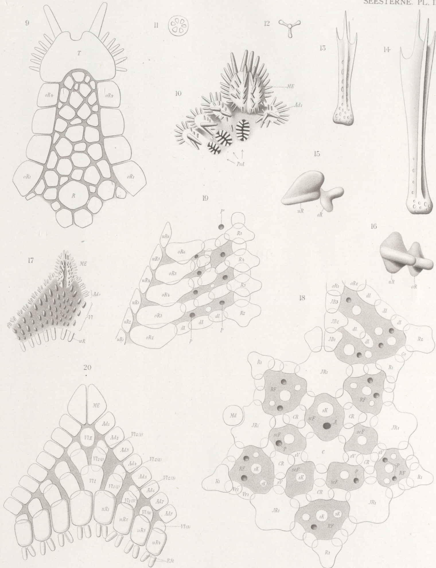
Fig. 9-10. Cheiraster gerlachei n. sp. — Fig. 11-17. Mimaster cognatus Sladen. Fig. 18-20. Porania antarctica E. A. Smith.
