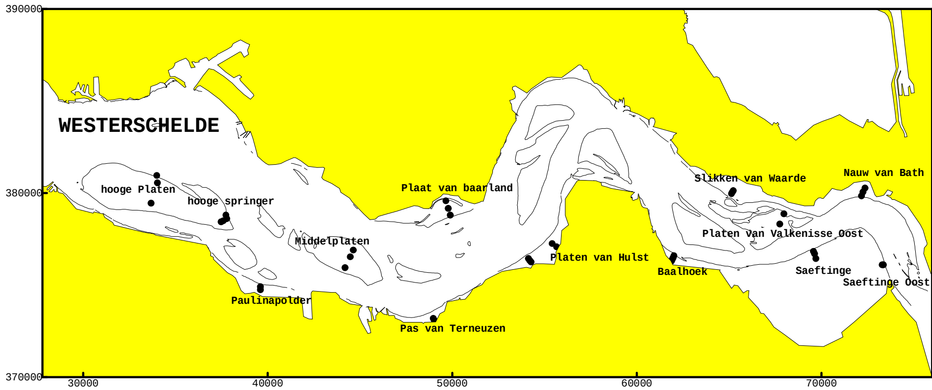
Figuur 2. Ligging van de vaste eutiorale locaties (raaien).
