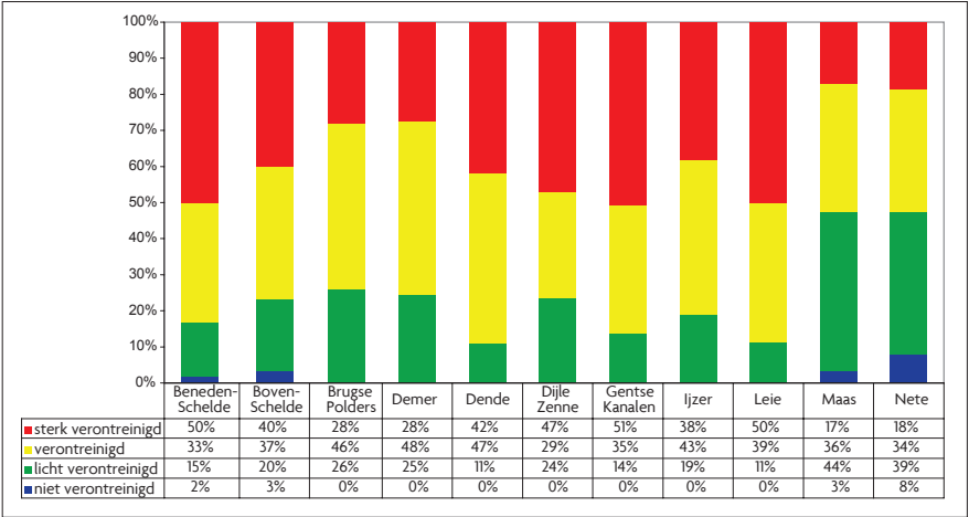
Ecologische waterbodemkwaliteit
