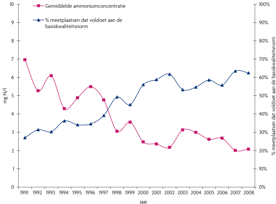
Ammoniumconcentratie
