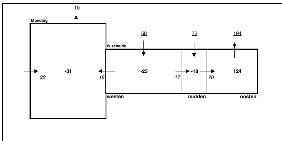
Fig. 3.8 Zand/waterbalans t.o.v. NAP+2m over de totale periode 1999-2030 na derde verdieping, variant c. V_{tot,E} = vet, totale inhoudsverandering berekend door ESTMORF, V_i = onderstreept, totale netto ingreep. I/E = cursief, import/ export van zanduit tussen deelgebieden.
