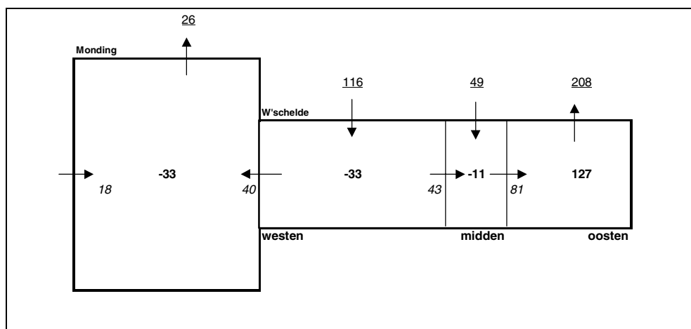
Fig. 3.6 Zand/waterbalans t.o.v. NAP+2m over de totale periode 1999-2030 na derde verdieping, variant b. V_{tot,E} = vet, totale inhoudsverandering berekend door ESTMORF, V_i = onderstreept, totale netto ingreep. I/E = cursief, import/ export van zanduit tussen deelgebieden.
