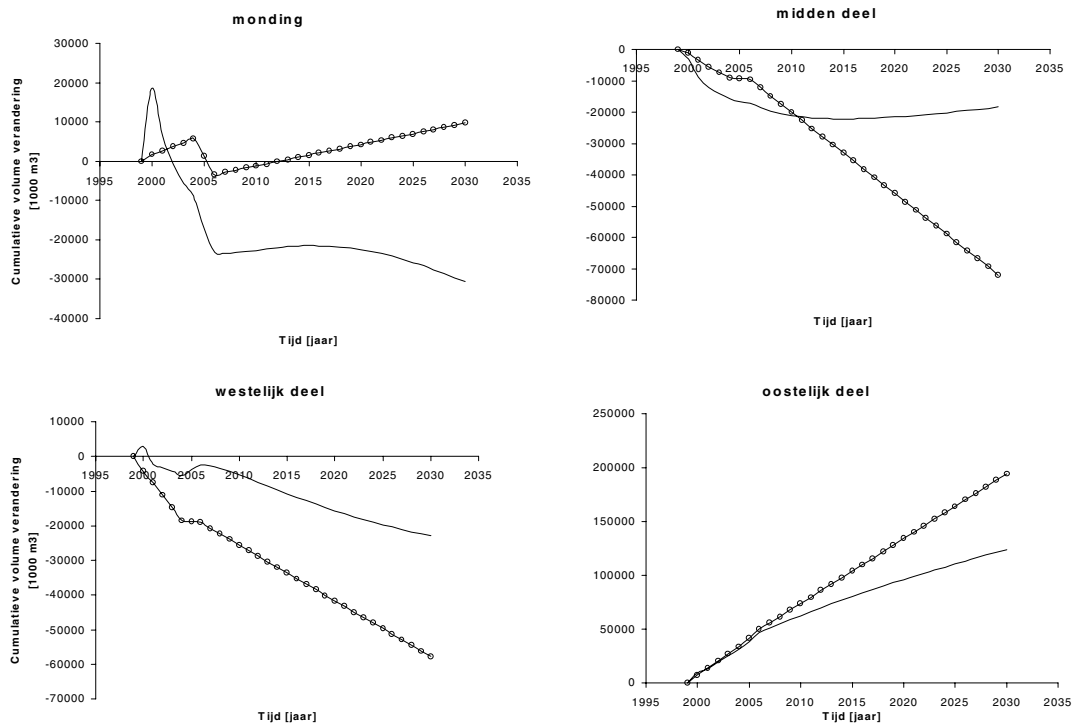
Figuur 3.7 Tijdreeksen van de cumulatieve totale inhoudsveranderingen V_{tot} (—) en de netto ingrepen V_i (---o) als gevolg van de derde verdieping, variant c.
