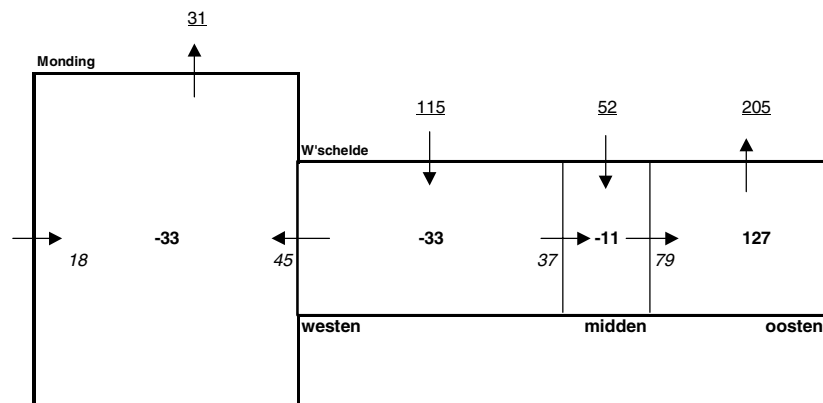
Fig. 3.4 Zand/waterbalans t.o.v. NAP+2m over de totale periode 1999-2030 na derde verdieping, variant a. V_{\text{tot,E}} = vet, totale inhoudsverandering bereknd door ESTMORF, V_i = onderstreept, totale netto ingreep. I/E = cursief, import/ export van zanduit tussen deelgebieden.
