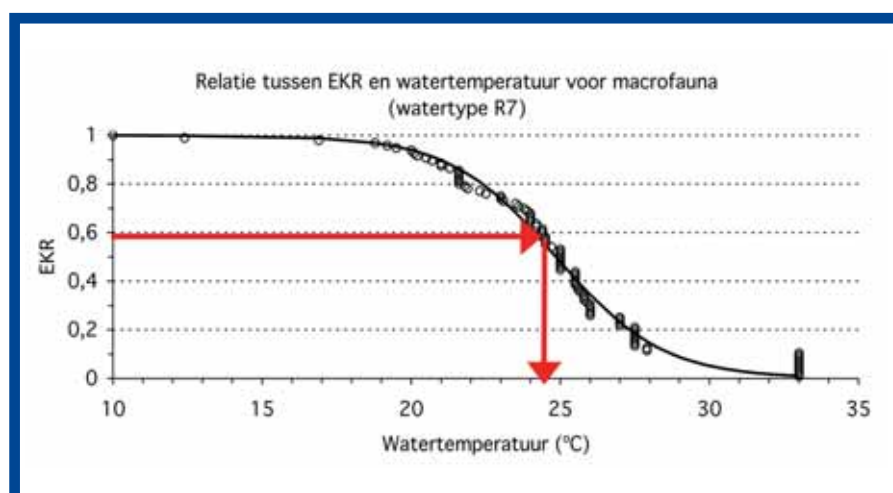
Afb. 2: Relatie tussen de ecologische kwaliteitsratio (EKR) en de watertemperatuur voor macrofaunasoorten uit de R7-watervallen. De EKR wordt berekend op basis van de KRW-maatlat voor macrofauna in R7-watervallen. De grens tussen matige en goede ecologische toestand ligt op een EKR van 0,6. Dit is hiermee de grens voor temperatuur.
