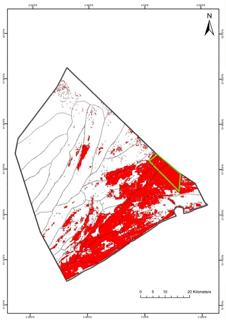
3128 3129 Figuur 4.3 Voorstel tot aanmelding van een habitatrichtlijngebied (groene box) (i.f.v. gemodelleerde 3130 verspreiding van Lanice conchilega aggregaties met rifkenmerken: rood) in het oostelijk deel van het Belgisch 3131 deel van de Noordzee. 3132 3133 3134 3135
