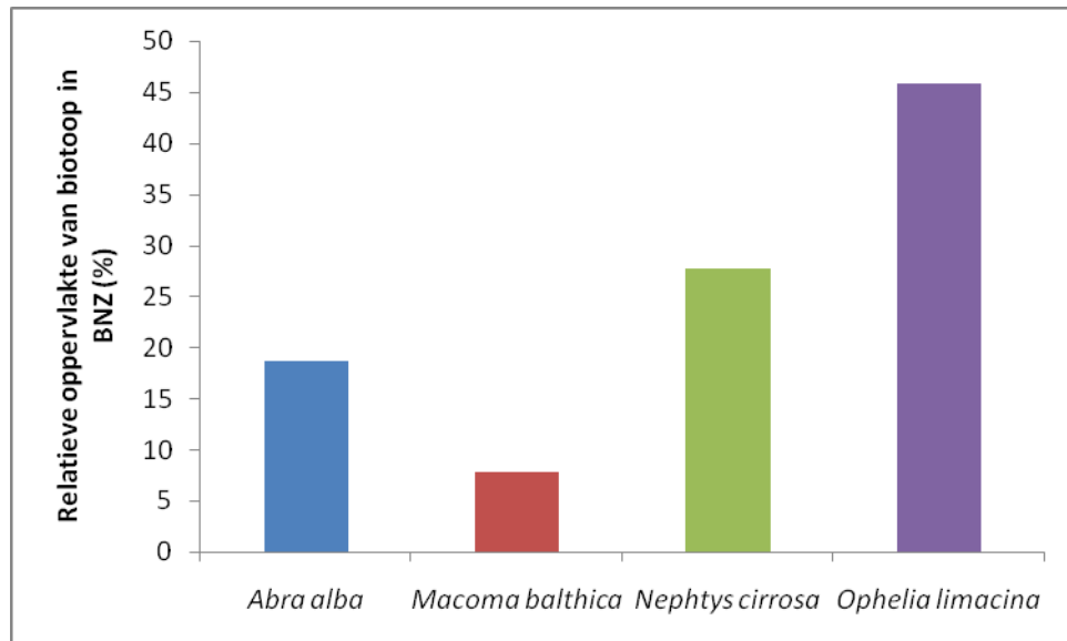
Figuur 1.5 Relatieve oppervlakte van de biotoop in het Habitattype 1110.
