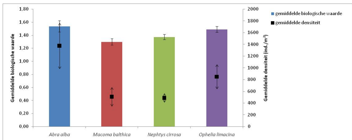
Figuur 1.6 Gemiddelde biologische waarde (histogram, bits) en densiteit (zwart blokje, ind./m²) met standaardfout per biotoop.
