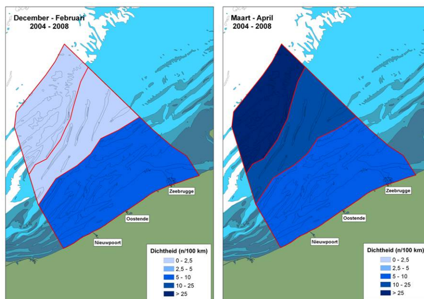
Figuur 2.10: Seizoensale patronen in het voorkomen van de Bruinvis in de Belgische zeegebieden gebaseerd op scheepstellingen van het INBO.
