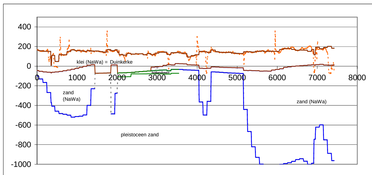
Figuur 4: Geologische doorsnede
