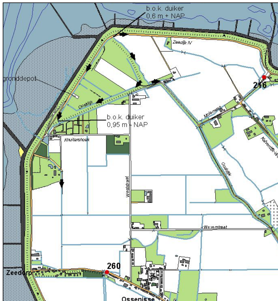
Figuur 7: Huidige situatie van het gebied met het afwateringsstelsel en de ligging van de grondwatermeetpunten en het gronddepot.
