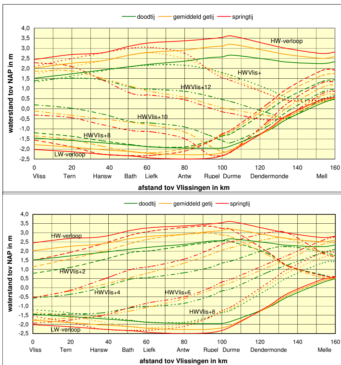
fig. 5.4 waterstandsverhanglijn ebfase HW- en LW- verloop voor dood-, gemiddeld en springtij
