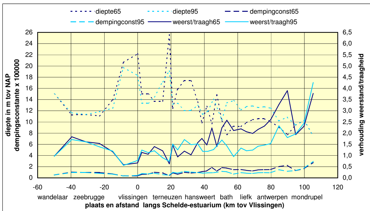
fig. 6.8 veranderingen 1965-1995 van diepte / hydraulische straal en met HARMSCHEDES gesimuleerde veranderingen van dempingsconstante en golfgetal
