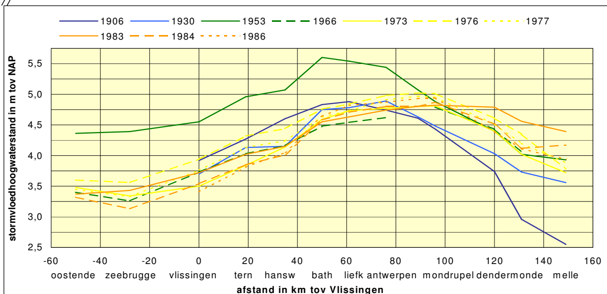
fig. 5.16 doordringing in het Schelde-estuarium van buitengewone stormvloed van 1983, 1984 en 1986, vergeleken met doordringing in periode 1906-1977
