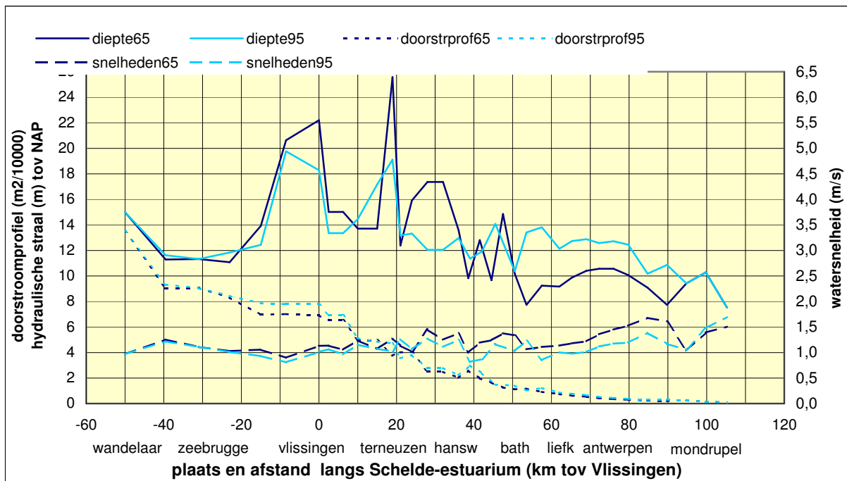
fig. 6.7 veranderingen 1965-1995 diepte / hydraulische straal, doorstrooprofien en met HARMSCHEDES gesimuleerde snelheden
