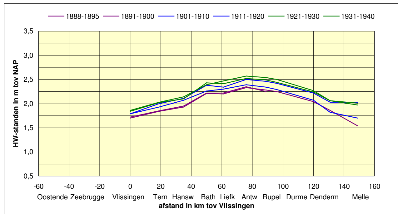
fig. 5.6 ontwikkeling HW-standen gemiddeld getij tussen 1888 en 1940
