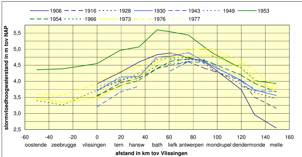
fig. 5.15 doordringing in het Schelde-estuarium van buitengewone stormvloed 1973, 1976 en 1977 vergeleken met doordringing in periode 1906 - 1966
