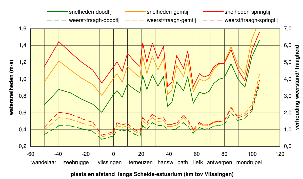
fig. 6.4 simulaties watersnelheden en verhouding weerstand / traagheid bij dood-, gemiddeld en springtij, met HARMSCHELDE95
