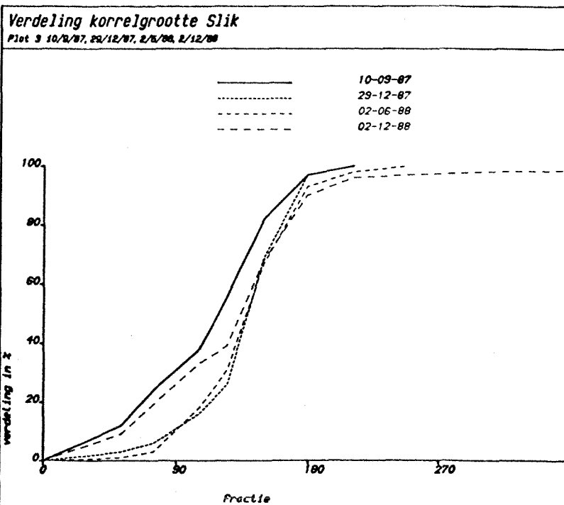
Figuur 9 Korrelgrootte verdeling plot 1, 2 en 3
