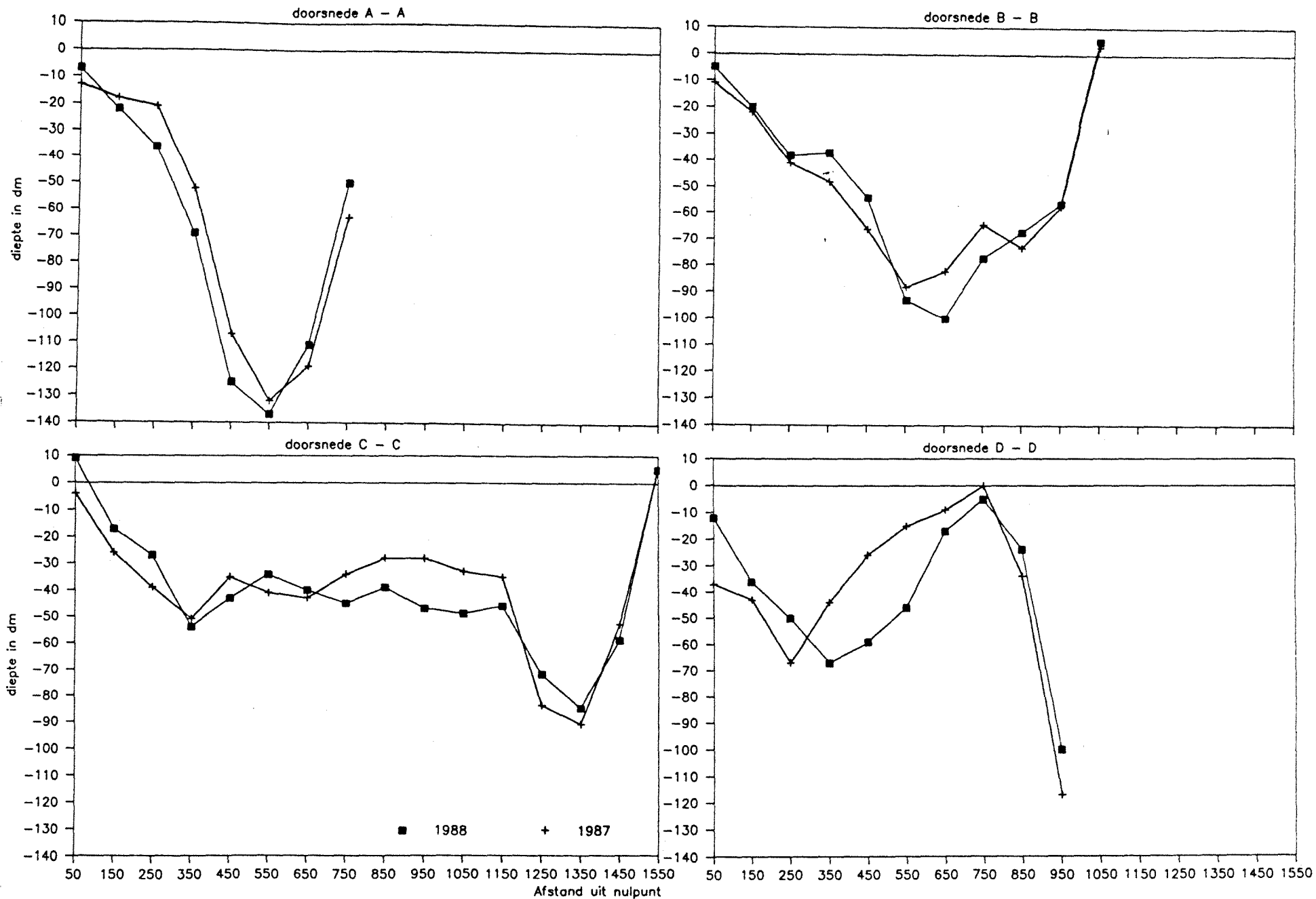
Figur 5b. Bodemligging '87-'88 in diverse doorsneden Schaar v. Valkenisse
