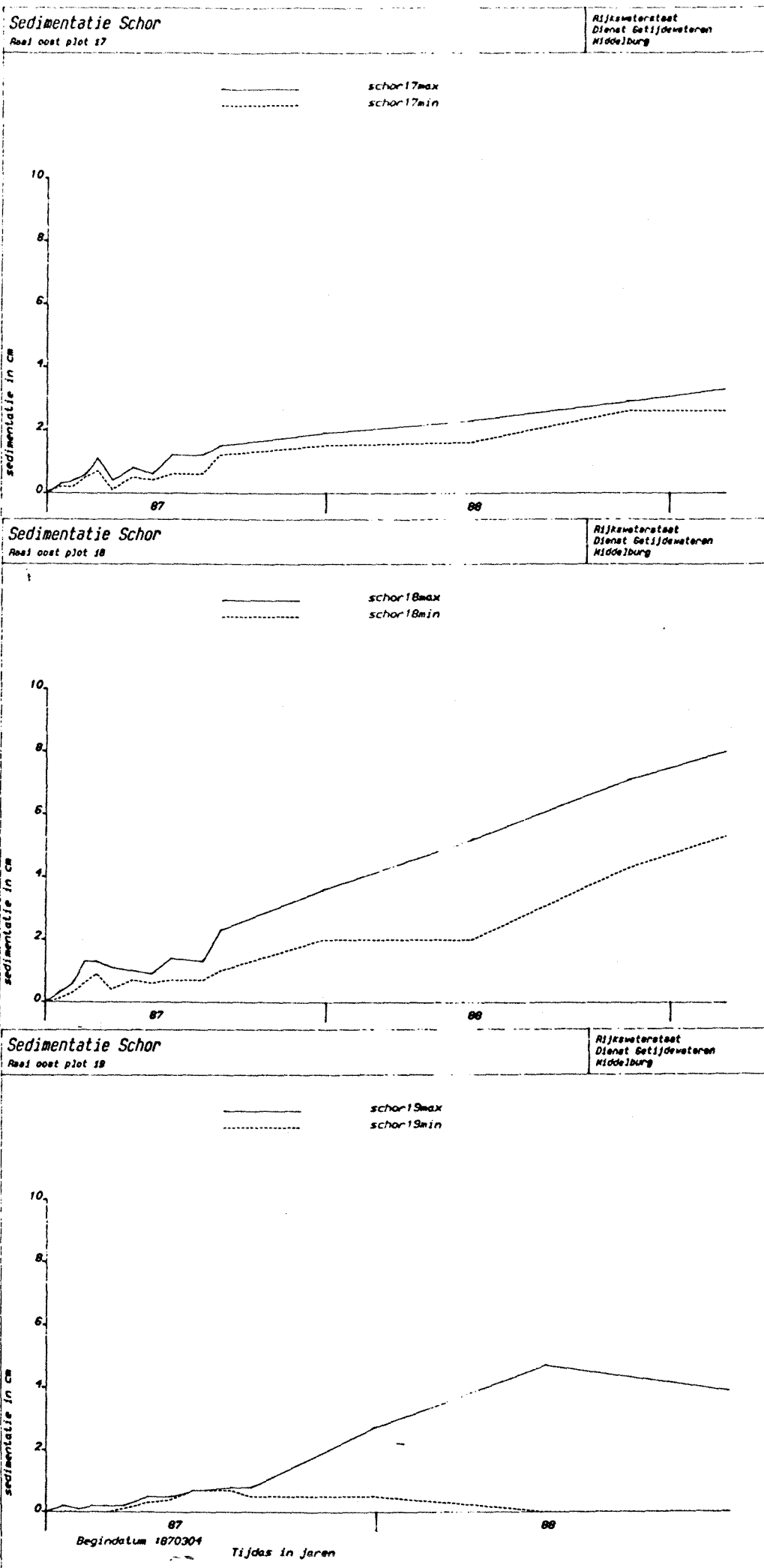
Flauur 14. Sedimentatie op het schor in plot 17, 18 en 19
