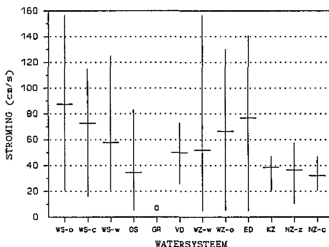
Figuur 15: De stroomsnelheden in de onderzochte watersystemen.
