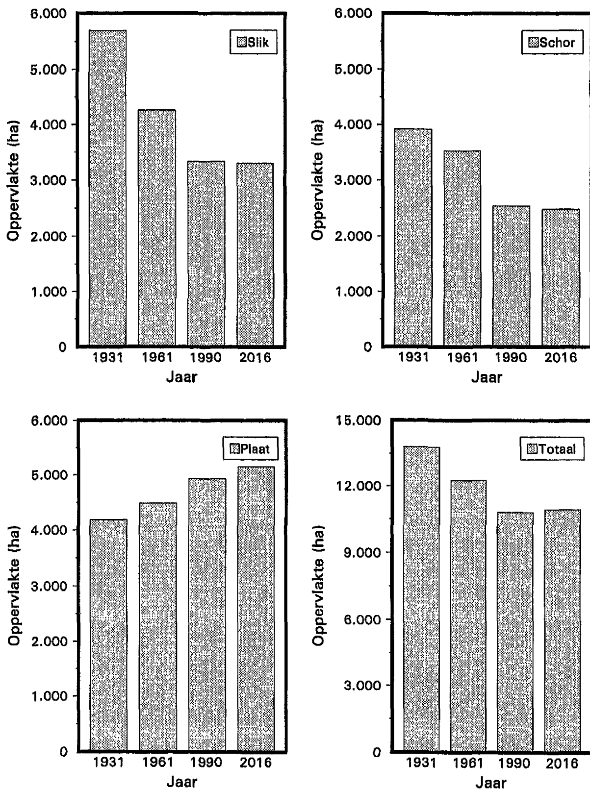
Figuur 3a: Historische ontwikkeling in de arealen intergetijdgedied in de Westerschelde.
