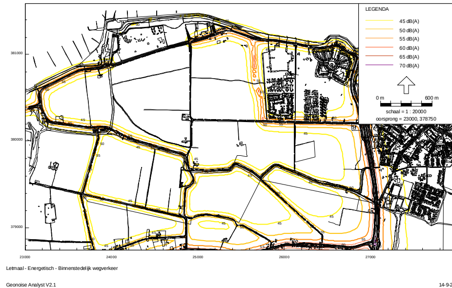
Figuur 7-13 Geluidscontouren voor Natuurlijk, inclusief aftrek art 103 Wgh (*)
