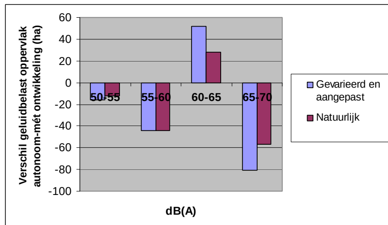
Figuur 7-14 Vershil geluidsbelast oppervlak in autonome situatie en inclusief Waterdunen
