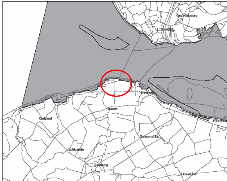
Figuur 5-11 Uitsnede kaart Habitatrictlijngebied Westerschelde
