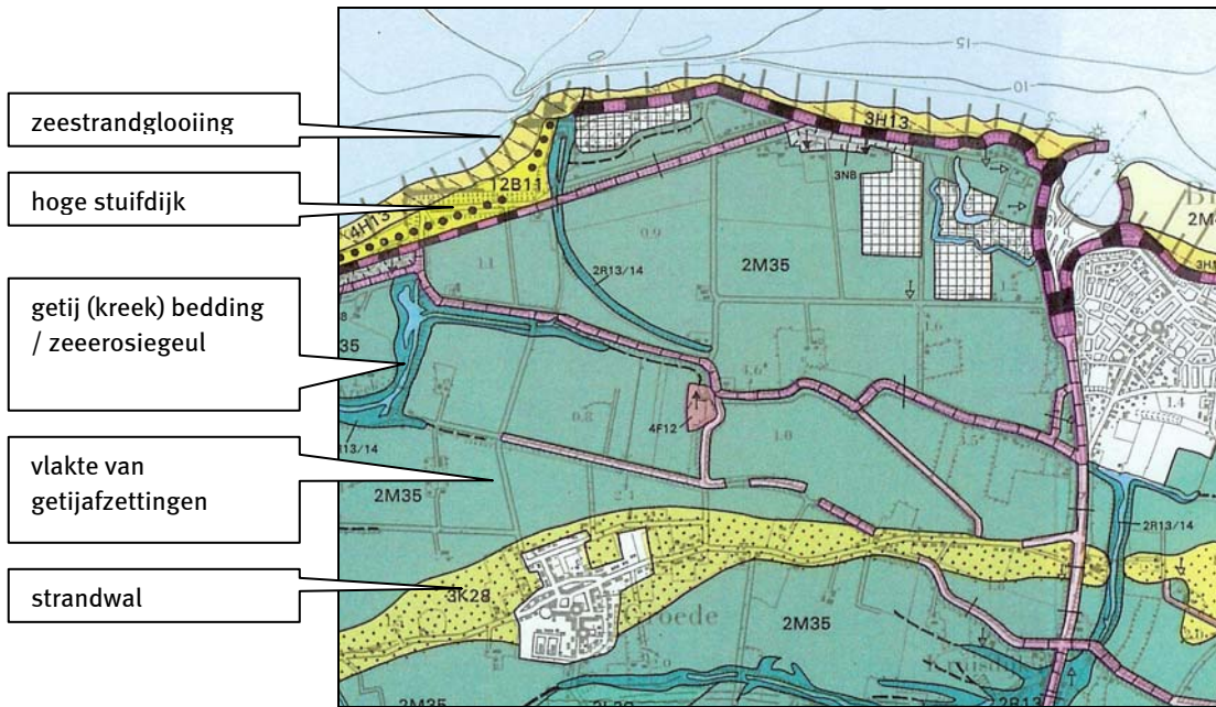
Figuur 5-6 Geomorfologische kaart (Stiboka 1987)
