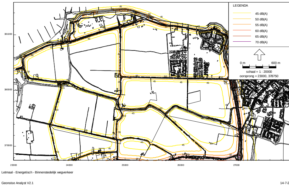
Figuur 5-17 Huidige situatie geluidbelasting plangebied en omgeving, inclusief aftrek art 103 Wgh
