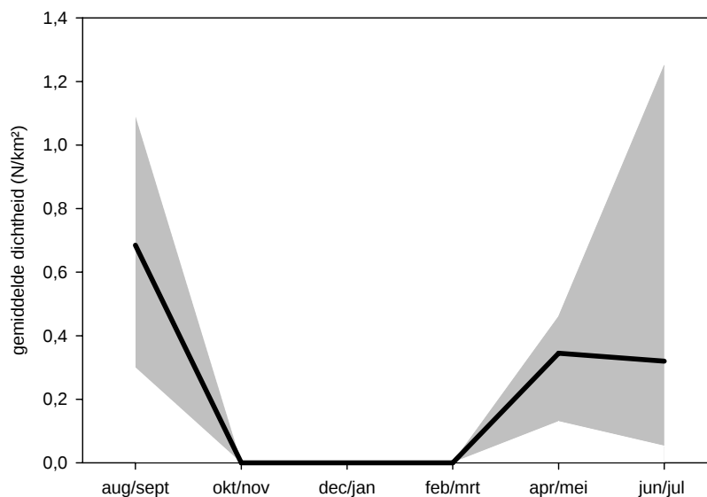
Figuur 3.7.2. Gemiddelde voorspelde dichtheid (lijn) en minimum/maximum voorspelde dichtheid (grijs vlak) in 2003-2008 van de Visdief/Noordse Stern op het Nederlands Continentaal Plat (NCP). Average predicted density (line) and minimum/maximum predicted density in 2003-2008 of the Common Tern/Arctic Tern on the Dutch Continental Shelf.
