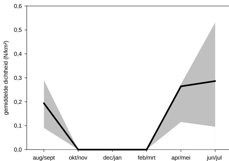
Figuur 3.6.2. Gemiddelde voorspelde dichtheid (lijn) en minimum/maximum voorspelde dichtheid (grijs vlak) in 2003-2008 van de Grote Stern op het Nederlands Continentaal Plat (NCP). Average predicted density (line) and minimum/maximum predicted density in 2003-2008 of the Sandwich Tern on the Dutch Continental Shelf.
