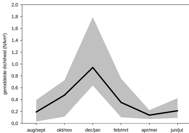
Figuur 3.4.2. Gemiddelde voorspelde dichtheid (lijn) en minimum/maximum voorspelde dichtheid (grijs vlak) in 2003-2008 van de Zilvermeeuw op het Nederlands Continentaal Plat (NCP). Average predicted density (line) and minimum/maximum predicted density in 2003-2008 of the Herring Gull on the Dutch Continental Shelf.
