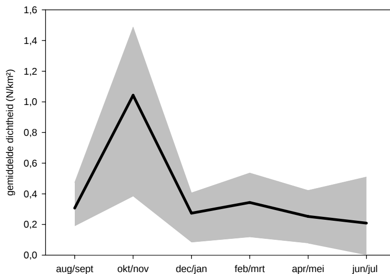
Figuur 3.2.2. Gemiddelde voorspelde dichtheid (lijn) en minimum/maximum voorspelde dichtheid (grijs vlak) in 2003-2008 van de Jan van Gent op het Nederlands Continentaal Plat (NCP). Average predicted density (line) and minimum/maximum predicted density in 2003-2008 of the Northern Gannet on the Dutch Continental Shelf.
