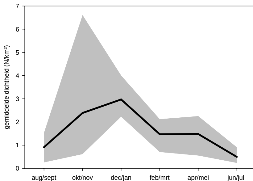
Figuur 3.5.2. Gemiddelde voorspelde dichtheid (lijn) en minimum/maximum voorspelde dichtheid (grijs vlak) in 2003-2008 van de Drieteenmeeuw op het Nederlands Continentaal Plat (NCP). Average predicted density (line) and minimum/maximum predicted density in 2003-2008 of the Kittiwake on the Dutch Continental Shelf.
