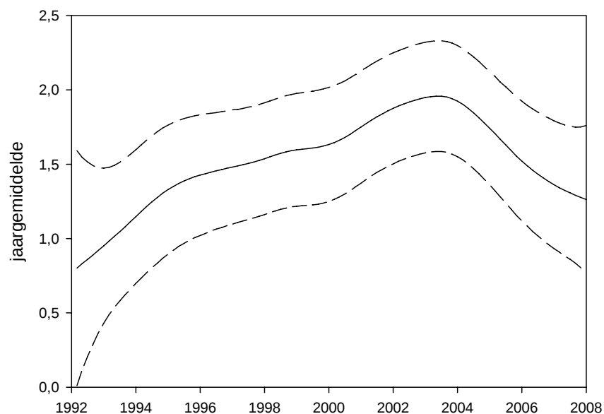
Figuur 3.5.3. Trend en 95% betrouwbaarheidsinterval van de Drieteenmeeuw op het Nederlands Continentaal Plat (NCP) in 1992-2008. Trend with 95% confidence limits of Kittiwake on the Dutch Continental Shelf in 1992-2008.
