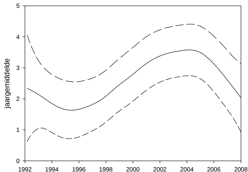
Figuur 3.8.3. Trend en 95% betrouwbaarheidsinterval van de Alk/Zeekoet op het Nederlands Continentaal Plat (NCP) in 1992-2008. Trend with 95% confidence limits of Common Guillemot/Razorbill on the Dutch Continental Shelf in 1992-2008.
