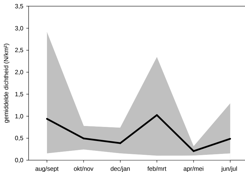
Figuur 3.1.2. Gemiddelde voorspelde dichtheid (lijn) en minimum/maximum voorspelde dichtheid (grijs vlak) in 2003-2008 van de Noordse Stormvogel op het Nederlands Continentaal Plat (NCP). Average predicted density (line) and minimum/maximum predicted density in 2003-2008 of the Fulmar on the Dutch Continental Shelf.
