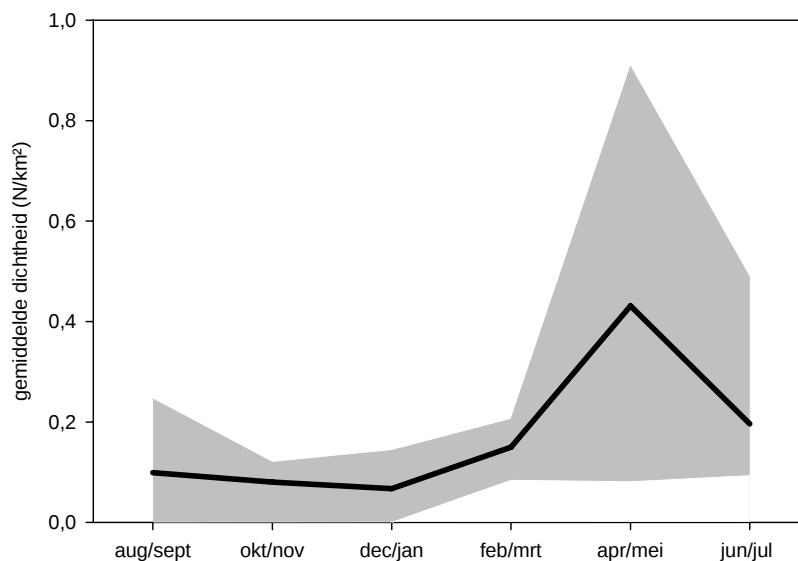
Figuur 3.9.2. Gemiddelde voorspelde dichtheid (lijn) en minimum/maximum voorspelde dichtheid (grijs vlak) in 2003-2008 van de Bruinvis op het Nederlands Continentaal Plat (NCP). Average predicted density (line) and minimum/maximum predicted density in 2003-2008 of the Harbour Porpoise on the Dutch Continental Shelf.
