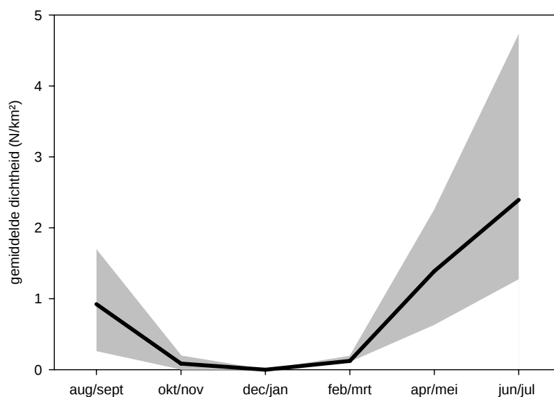
Figuur 3.3.2. Gemiddelde voorspelde dichtheid (lijn) en minimum/maximum voorspelde dichtheid (grijs vlak) in 2003-2008 van de Kleine Mantelmeeuw op het Nederlands Continentaal Plat (NCP). Average predicted density (line) and minimum/maximum predicted density in 2003-2008 of the Lesser Black-backed Gull on the Dutch Continental Shelf.
