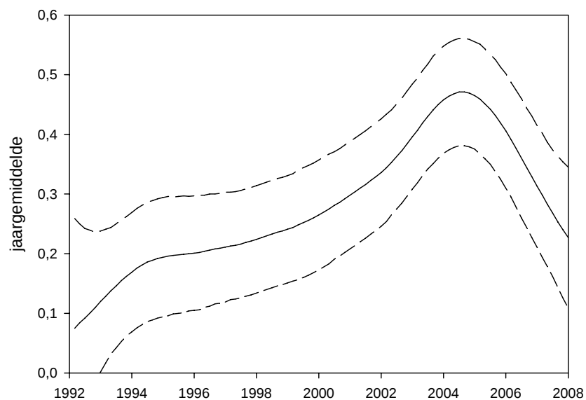
Figuur 3.2.3. Trend en 95% betrouwbaarheidsinterval van de Jan van Gent op het Nederlands Continentaal Plat (NCP) in 1992-2008. Trend with 95% confidence limits of Northern Gannet on the Dutch Continental Shelf in 1992-2008.
