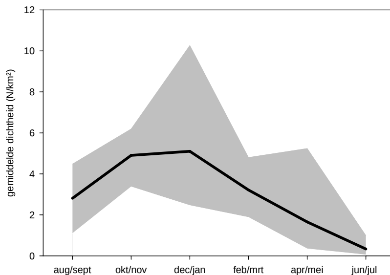
Figuur 3.8.2. Gemiddelde voorspelde dichtheid (lijn) en minimum/maximum voorspelde dichtheid (grijs vlak) in 2003-2008 van de Alk/Zeekoet op het Nederlands Continentaal Plat (NCP). Average predicted density (line) and minimum/maximum predicted density in 2003-2008 of the Common Guillemot/Razorbill on the Dutch Continental Shelf.
