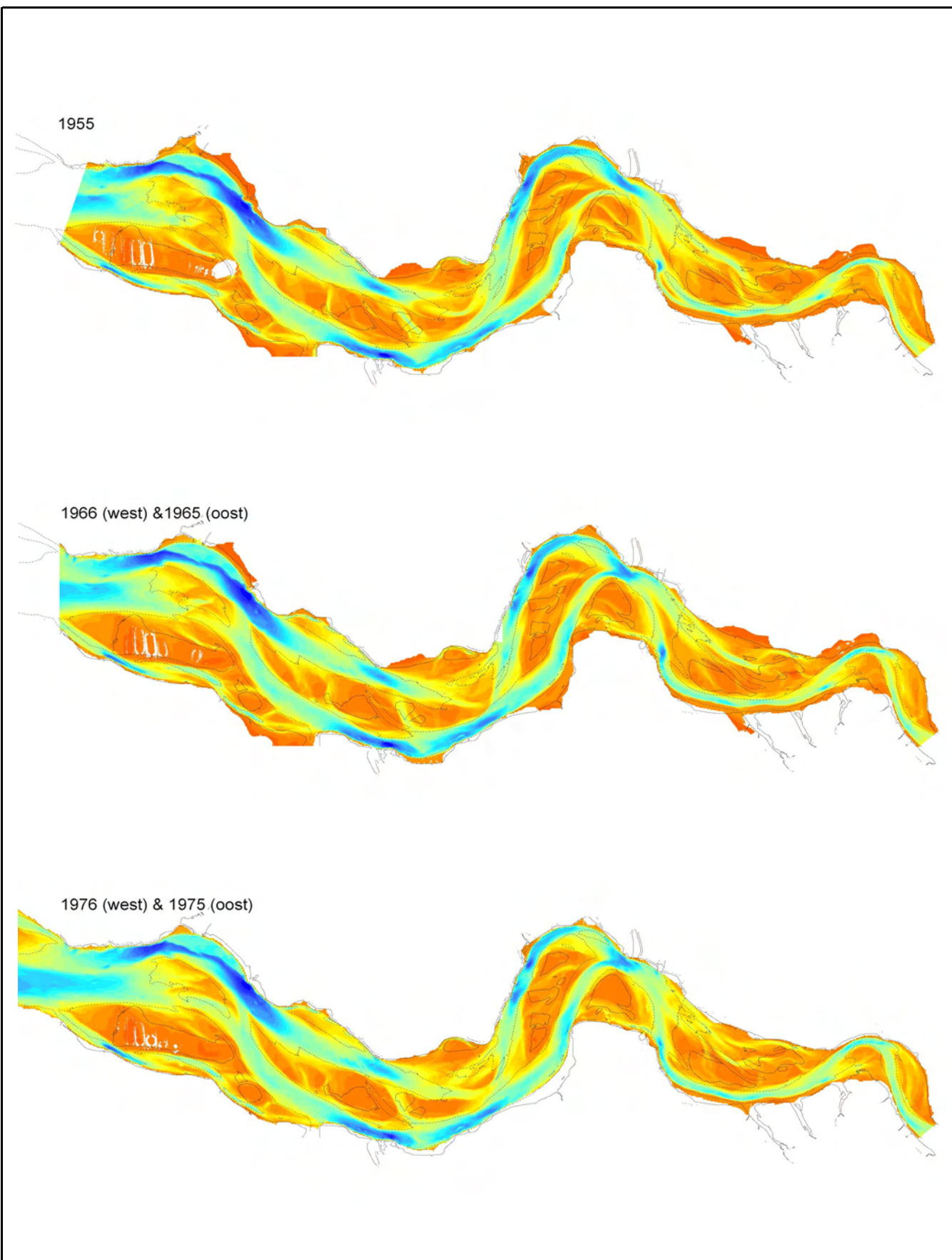
Lange termijn ontwikkeling van de Westerschelde Bodemligging 1955 tot 1976
