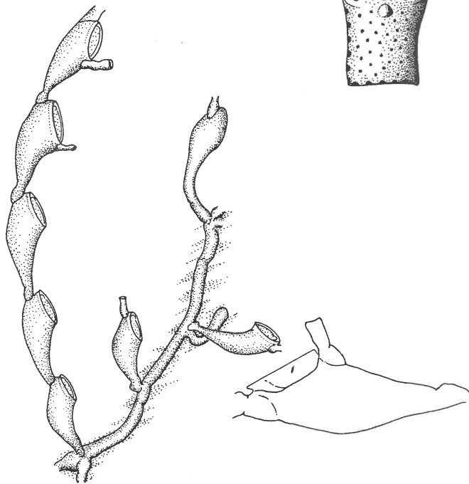
Fig. 10. Scruparia chelata
