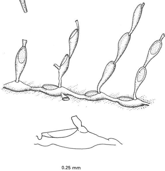
Fig. 7. Scruparia ambigua
