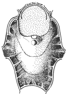
Fig. 8. Umbonula littoralis
