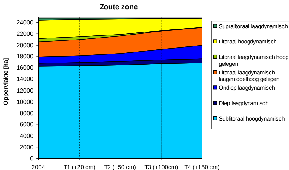
Figuur 5.3 Verschuiving van zoute habitatklassen ten gevolge van een waterstandstijging in de Westerschelde
