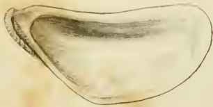
3-5 Dreissena
