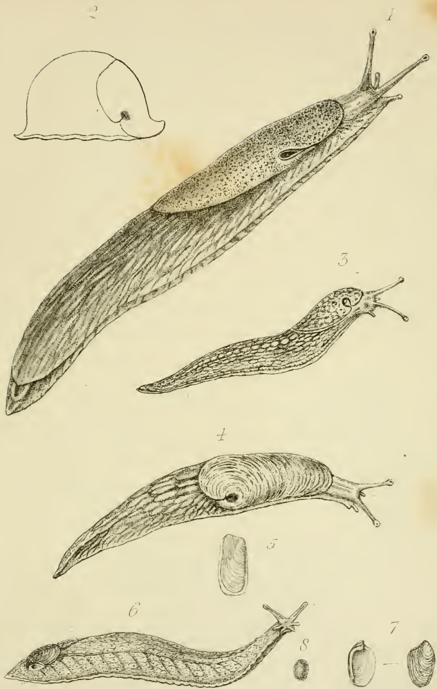
1-2. Arion .
