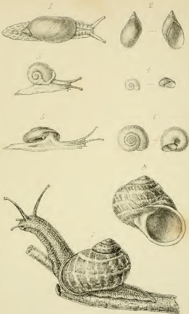
1-2. Succinea
