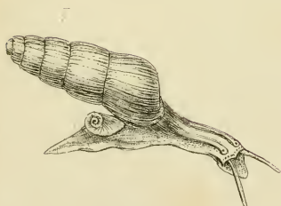
1-3. Carychium .
