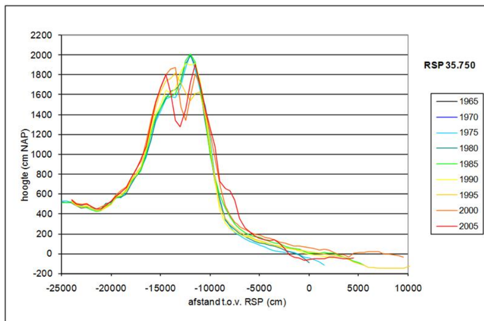
Figuur 6.6. Typend dwarsprofiel voor Bergen-Egmond.
