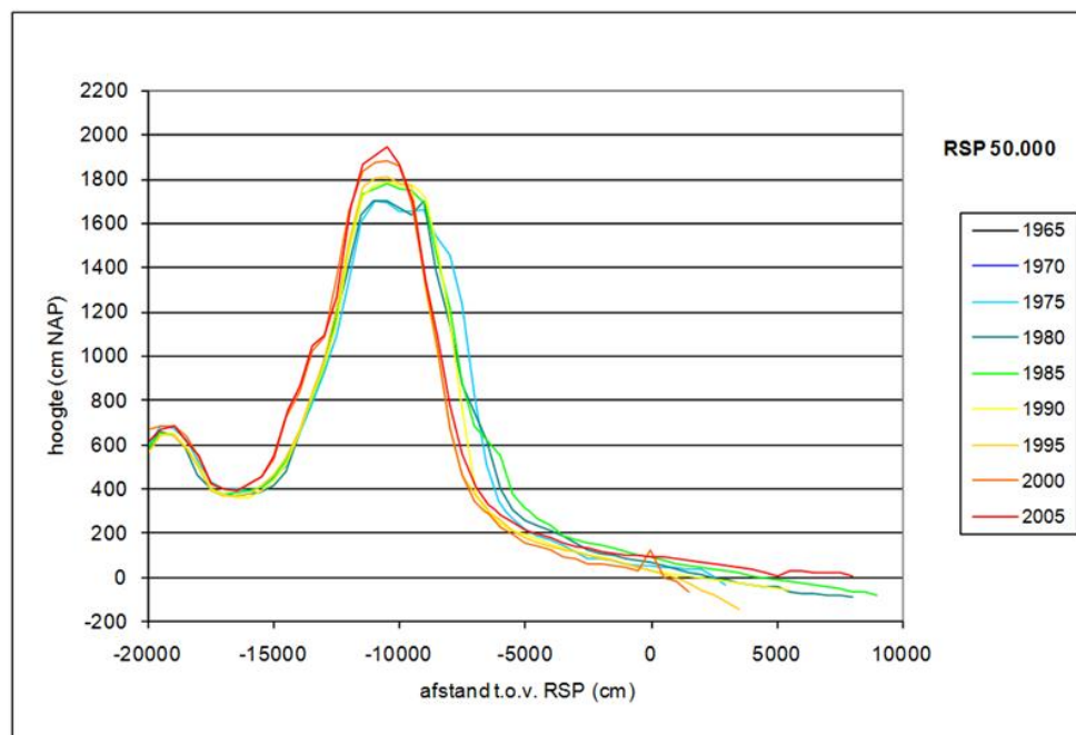
Figuur 6.10. Typend dwarsprofiel voor het gebied rond Heemskerk.
