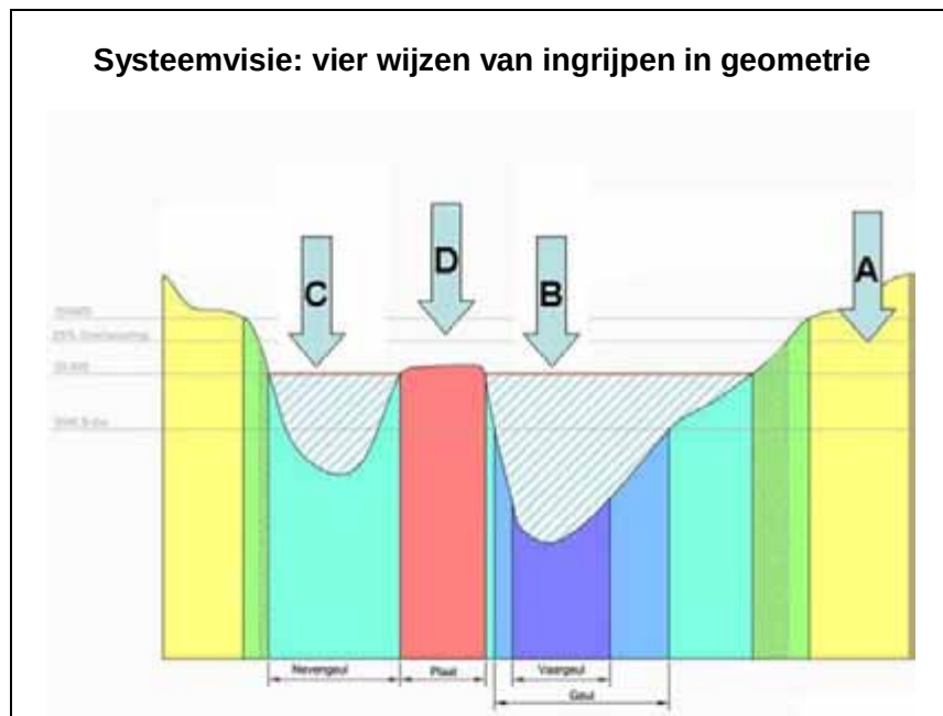
Figuur 3.2 Vier typen ingrepen om via aanpassing geometrie getijslag te beïnvloeden
