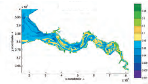
Figuur 5: Berekende slibfractie (-) in de bodem. Hoogdynamische gebieden zoals stroomgeulen bestaan voornamelijk uit zand, laagdynamische gebieden zoals (sommige) platen en havenbekkens hebben een slibrijke bodem.
