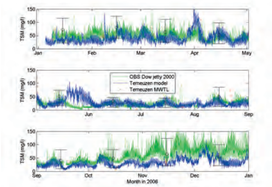
Figuur 4: Berekende (blauw) en gemeten (groen/rood/zwart) slibconcentratie bovenin de waterkolom bij Terneuzen in 2006.
