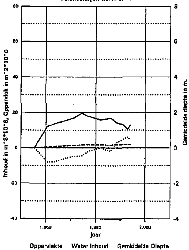
Hoofd Geul, Gat van Ossensisse Geulvak 10, onder NAP -5m Veranderingen t.o.v. 1955
