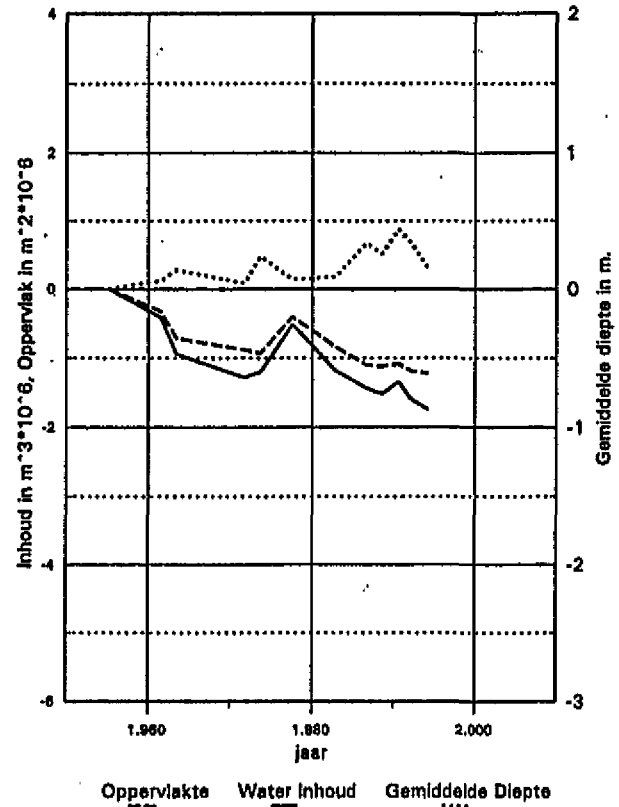
Hoofd Geul, Vaarwater boven Bath Geulvak 1, ondiepwater, tussen NAP-5m en NAP-2m Veranderingen t.o.v. 1955
