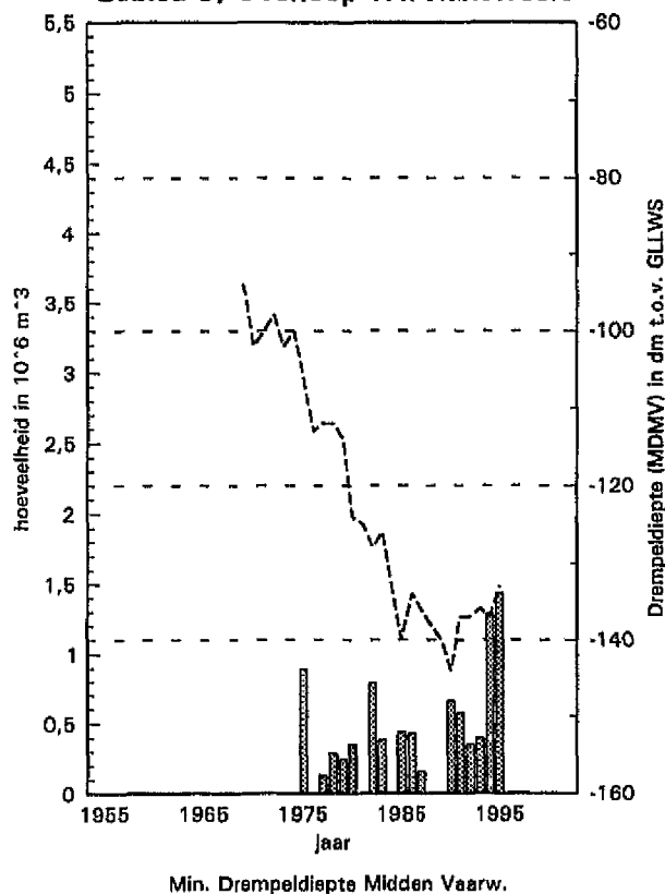
Baggerhoeveelheden en minste Drempeldiepte Gebied 9, Overloop van Hansweert
