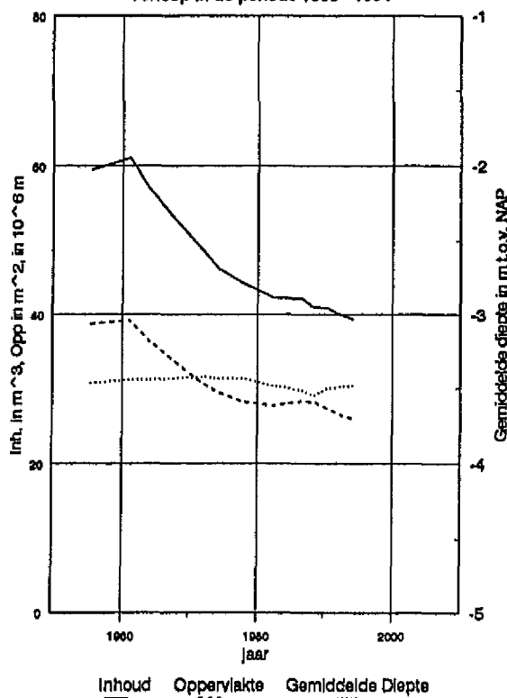
Gehele Westerschelde, Totaal Platen Ondiepwatergebied tussen NAP-5m en NAP-2m Verloop in de periode 1955 - 1994
