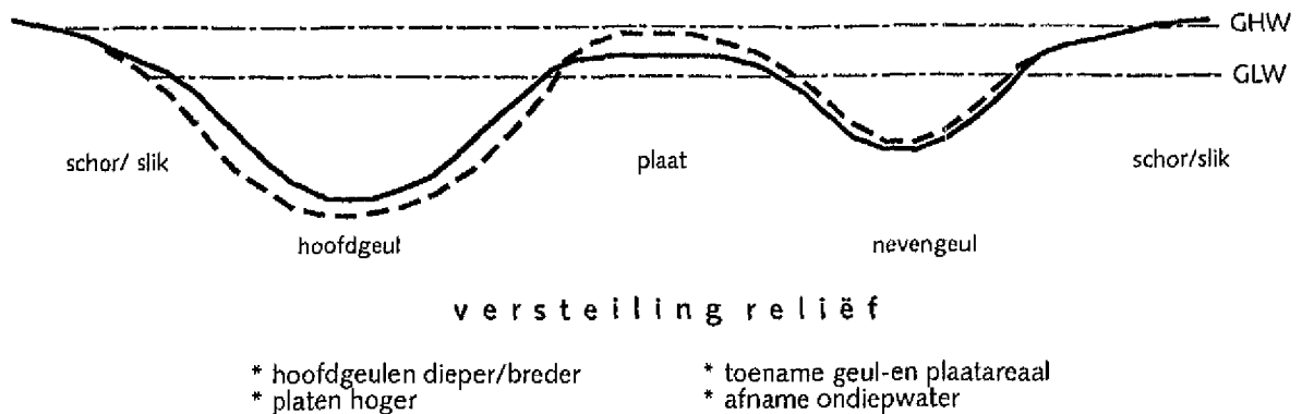
Figuur 2 Veranderingen in het bodemprofiel (doorgetrokken lijn: verleden; onder- broken lijn: huidige situatie)
