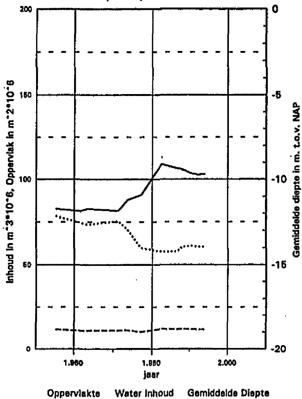
Hoofd Geul, Zuidergat Geulvak 5, onder NAP -5m Verloop in de periode 1955 - 1994
