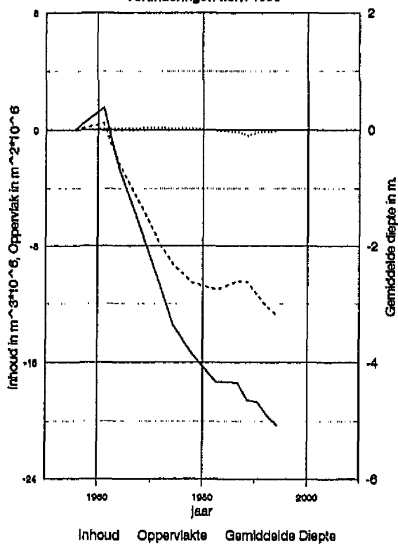
Gehele Westerschelde, Totaal Platen Ondiepwatergebied tussen NAP-5m en NAP-2m Veranderingen t.o.v. 1955
