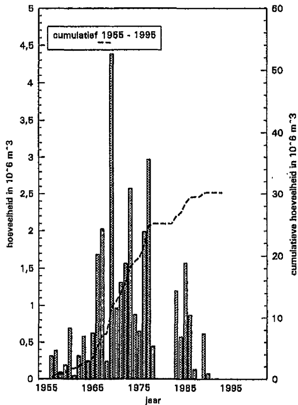
Westelijk deel Westerschelde Zandwinhoeveelheden t.b.v. Nederland
