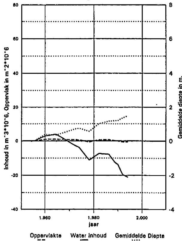
Neven Geul, Vaarwater langs Hoofdplaat Geulvak 14, onder NAP -2m Veranderingen t.o.v. 1955
