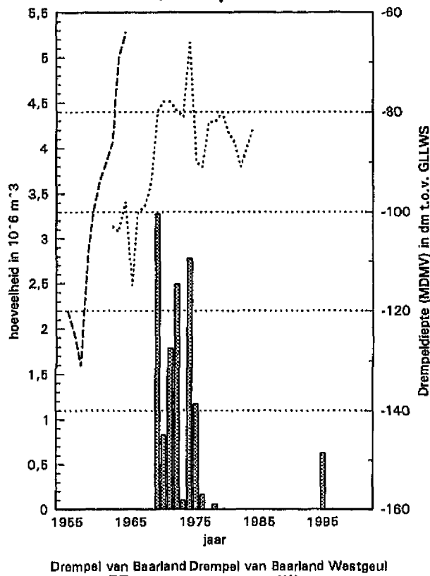
Baggerhoeveelheden en minste Drempeldiepte Gebied 11, Drempel van Baarland
