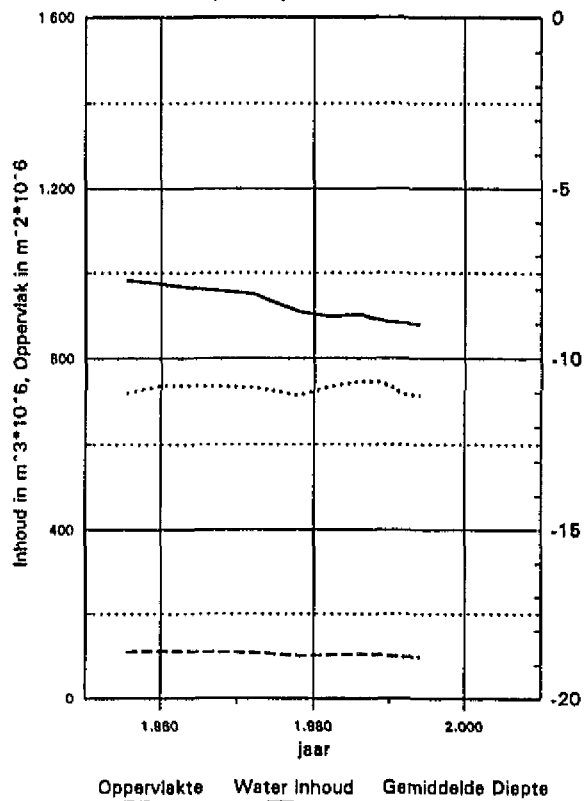
Gehele Westerschelde Neven Geulen, onder NAP -2m Verloop in de periode 1955 - 1994
