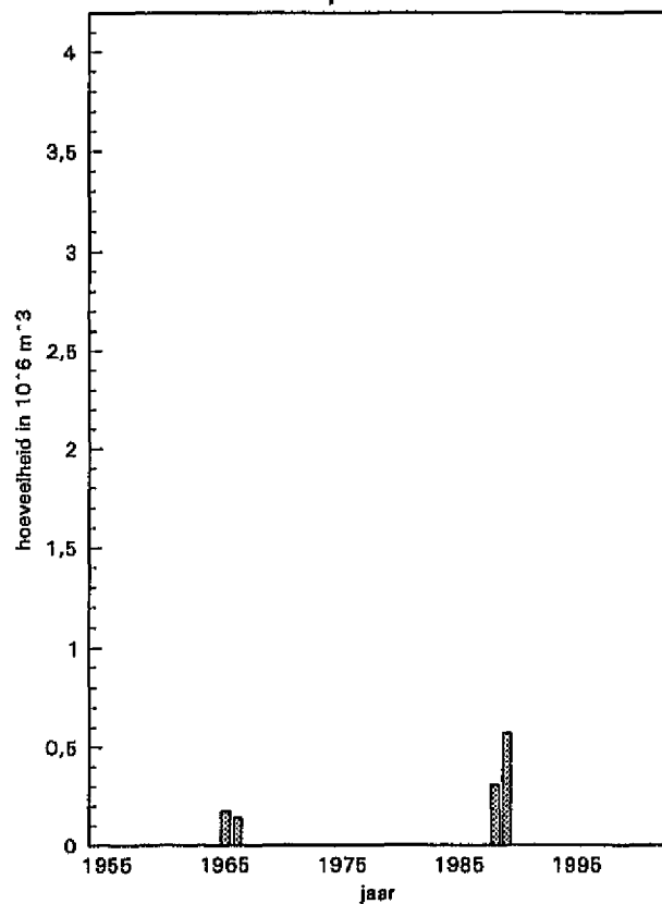
Stortheoevelheden Gebied 13 Perkpolder
