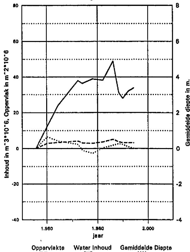
Neven Geul, Everingen Geulvak 13, onder NAP -2m Veranderingen t.o.v. 1955
