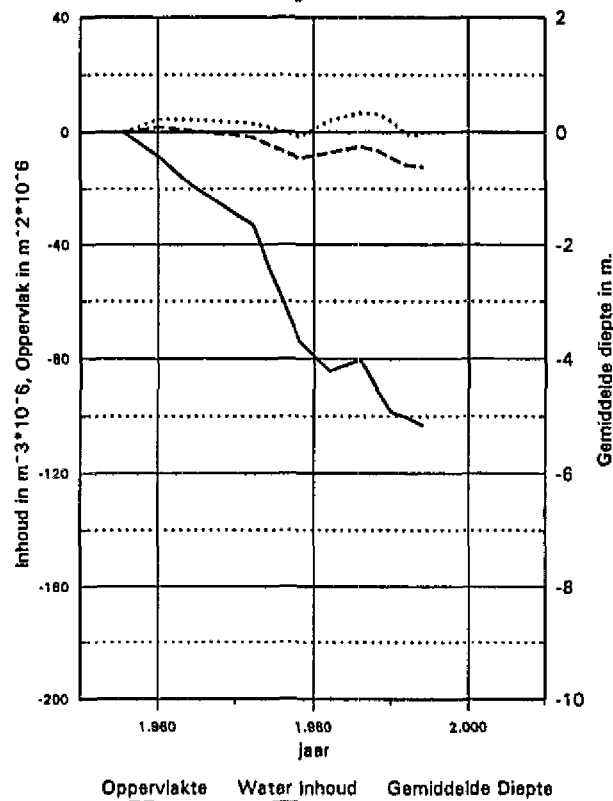
Gehele Westerschelde Neven Geulen, onder NAP -2m Veranderingen t.o.v. 1955
