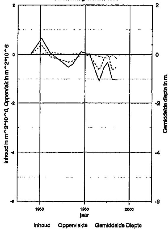
Plaat van Baarland, plaatvak 150 Ondiepwatergebied tussen NAP-5m en NAP-2m Veranderingen t.o.v. 1955
