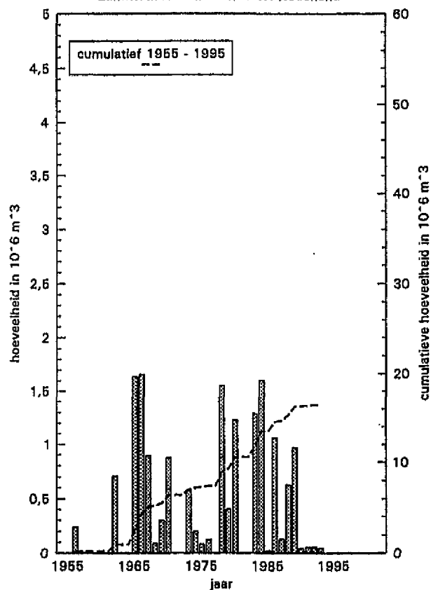
Oostelijk deel Westerschelde Zandwinhoeveelheden t.b.v. Nederland
