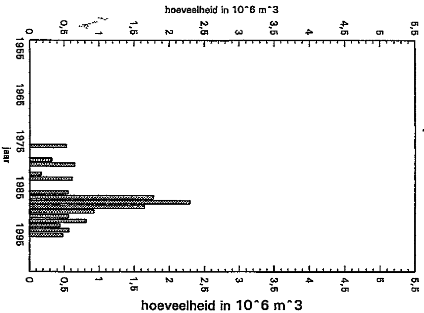
Baggerhoeveelheden Gebied 5 Overloop van Valkenisse
