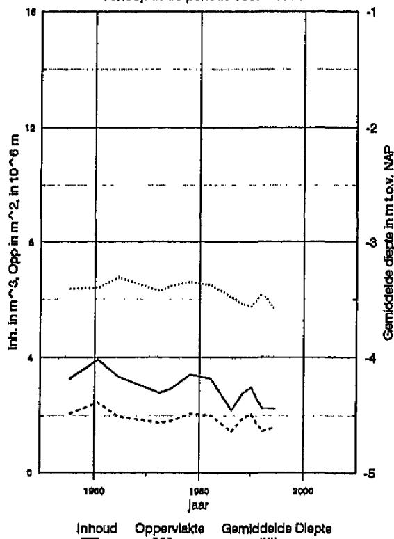
Plaat van Baarland, plaatvak 150 Ondiepwatergebied tussen NAP-5m en NAP-2m Verloop in de periode 1955 - 1994
