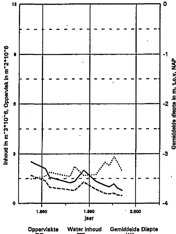
Hoofd Geul, Vaarwater boven Bath Geulvak 1, ondiepwater, tussen NAP-5m en NAP-2m Verloop in de periode 1955 - 1994
