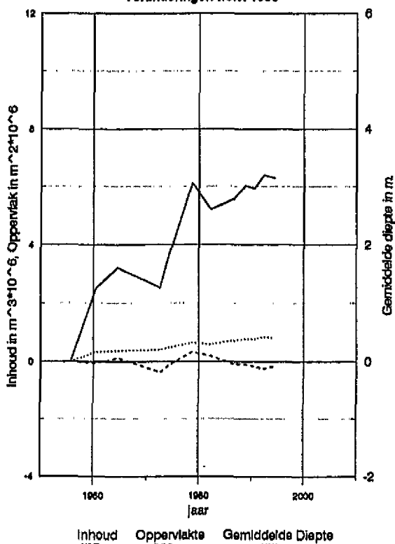
Hoge Platen Plaatvak 170, boven NAP -2m Veranderingen t.o.v. 1955
