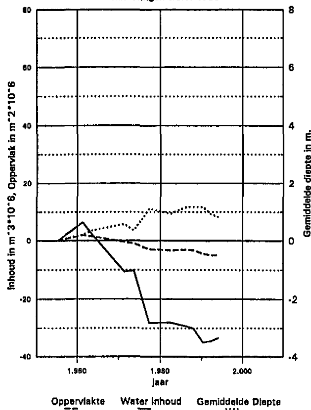
Nevengeul, Schaar van Valkenisse Geulvak 6, onder NAP -2m Veranderingen t.o.v. 1955
