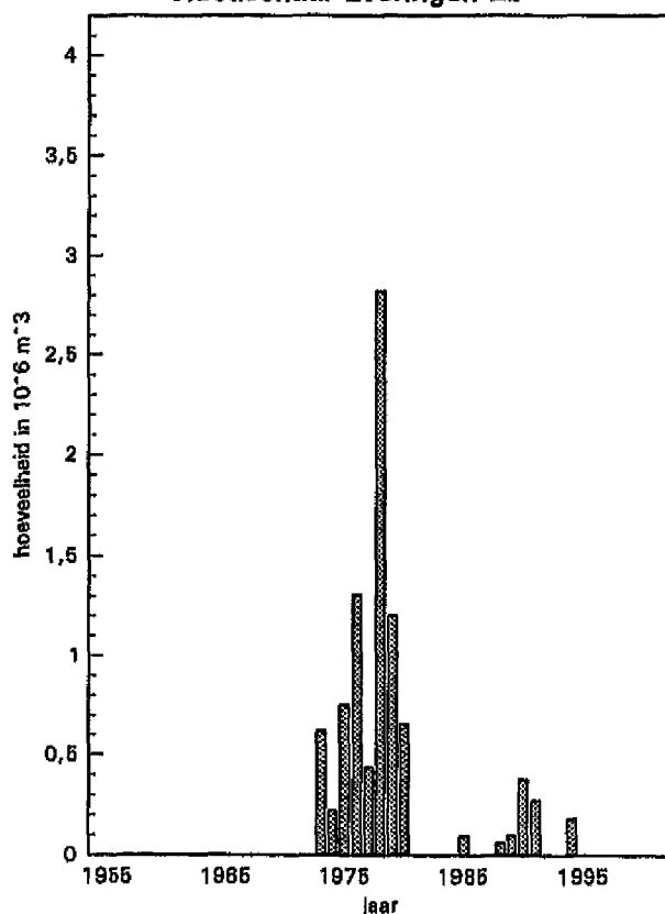
Stortheoevelheden Gebied 20 Vloedschaar Everingen Eb
