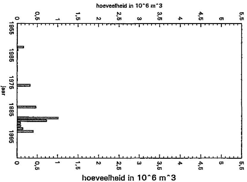
Baggerhoeveelheden Gebied 6 Platen van Valkenisse
