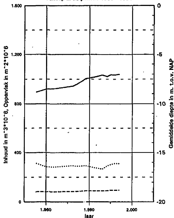
Gehele Westerschelde Hoofd Geulen, onder NAP -5m Verloop in de periode 1955 - 1994
