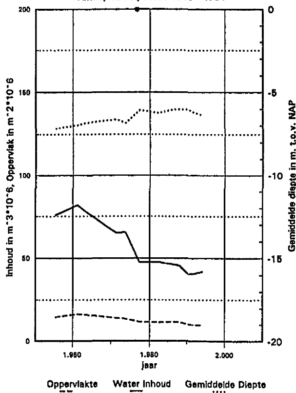
Neven Geul, Schaar van Valkenisse Geulvak 6, onder NAP -2m Verloop in de periode 1955 - 1994
