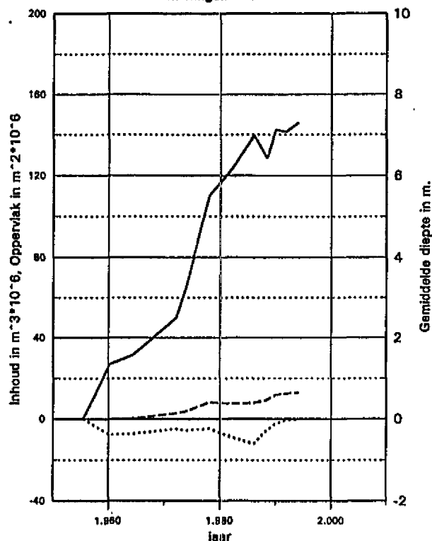
Gehele Westerschelde Hoofd Geulen, onder NAP -5m Veranderingen t.o.v. 1955
