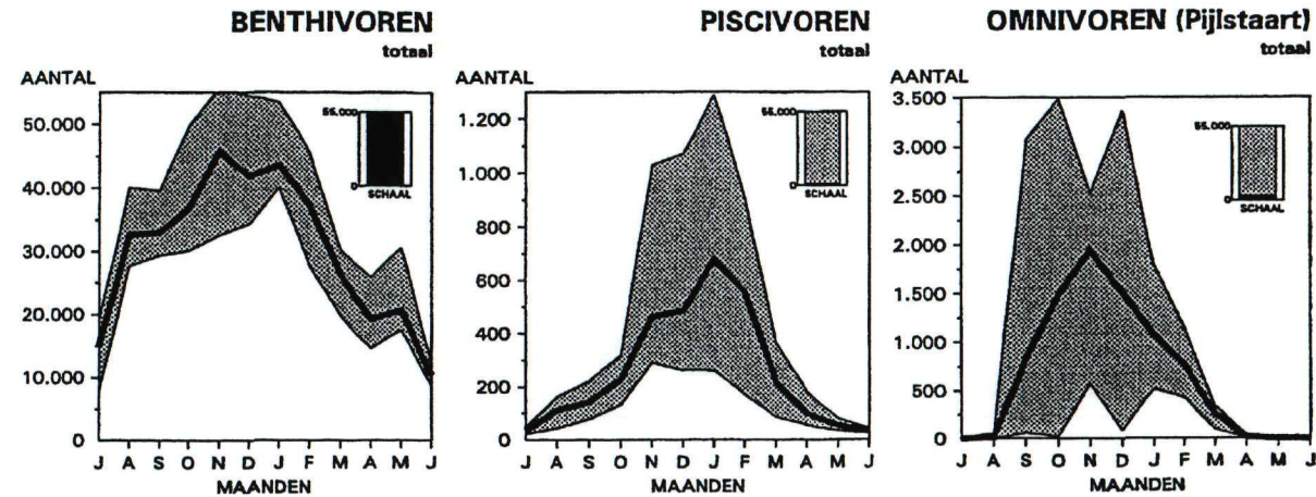
Figuur 3 Aantallen watervogels in de Westerschelde, op basis van de voedselgroepen (1979-1995) (grijs: extremen; dikke lijn: gemiddelde)
