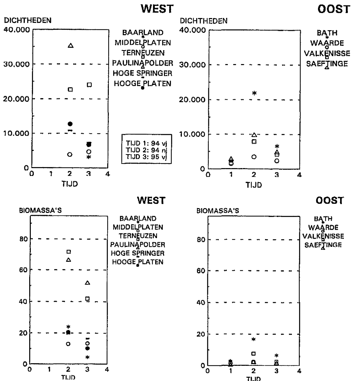
DICHTHEDEN (a) en BIOMASSA'S (b) PER DEELGEBIED (RAAIEN) NB: raai HULST vertegenwoordigt deelgebied MIDDEN
