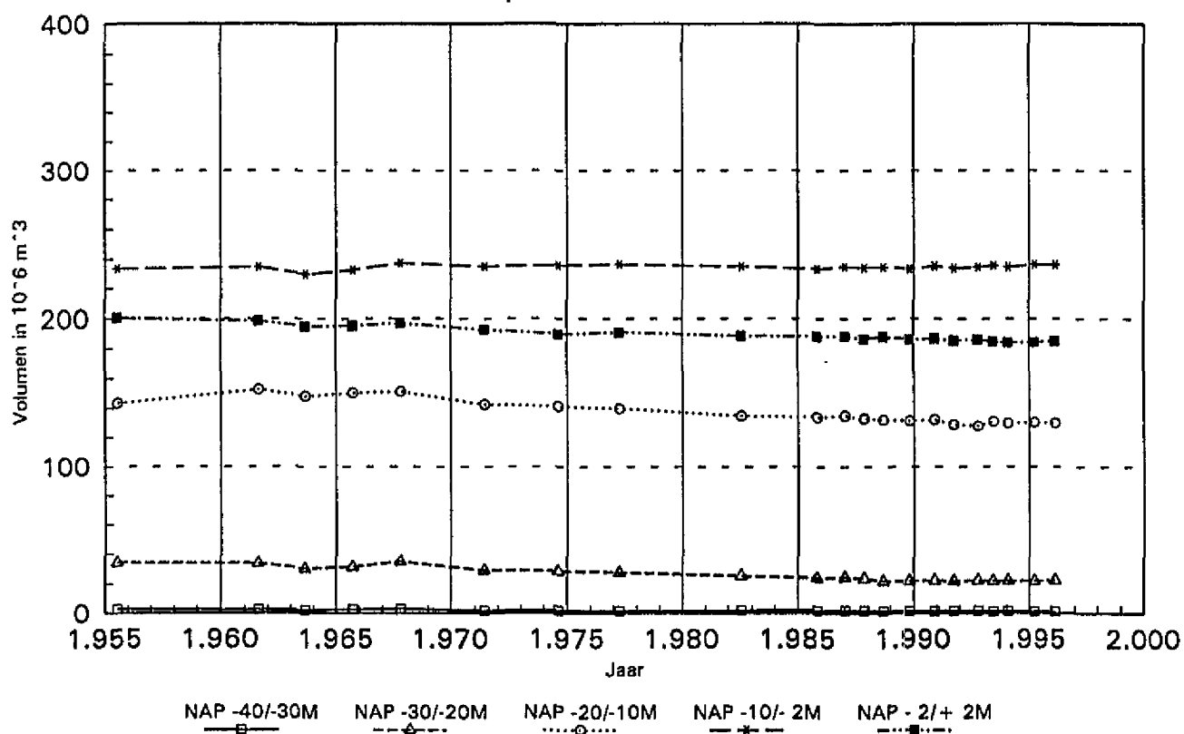
Volumeverloop tussen diverse niveau's
