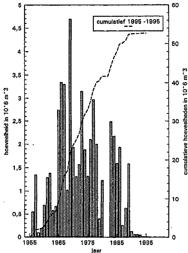
Gehele Westerschelde Zandwin hoeveelheden t.b.v. Nederland
