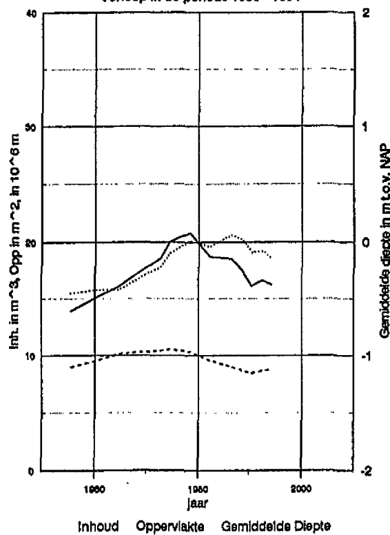
Middelplaten complex Plaatvak 160, boven NAP -2m Verloop in de periode 1955 - 1994
