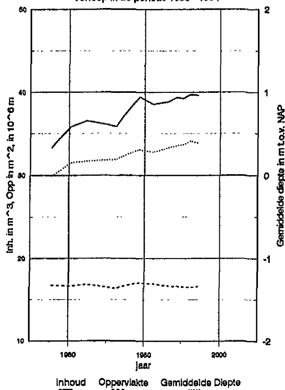
Hoge platen Plaatvak 170, boven NAP -2m Verloop in de periode 1955 - 1994
