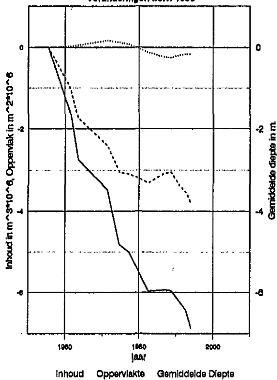
Rug van Baarland, plaatvak 140 Ondiepwatergebied tussen NAP-5m en NAP-2m Veranderingen t.o.v. 1955
