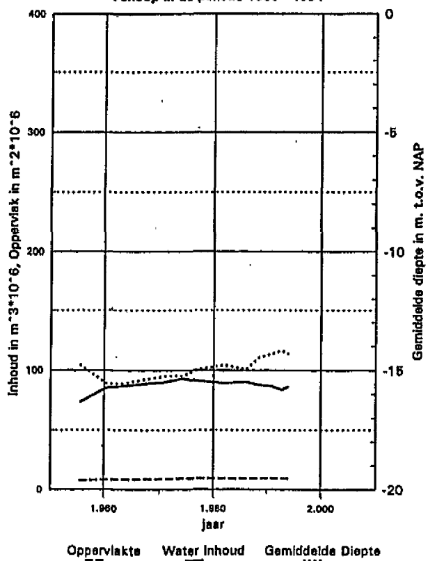
Hoofd Geul, Gat van Ossensisse Geulvak 10, onder NAP -5m Verloop in de periode 1955 - 1994
