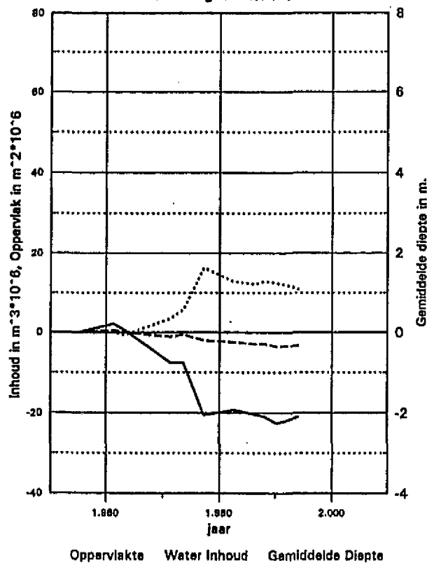
Nevengeul, Schaar van Valkenisse Geulvak 6, onder NAP -5m Veranderingen t.o.v. 1955
