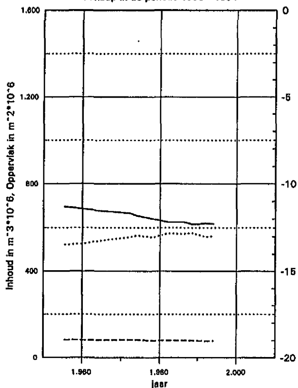
Gehele Westerschelde Neven Geulen, onder NAP -5m Verloop in de periode 1955 - 1994
