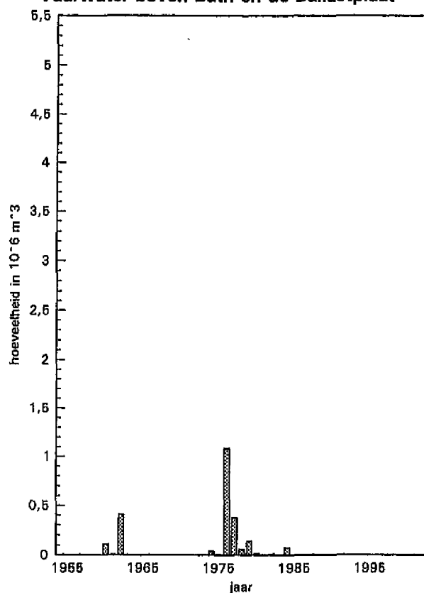
Baggerhoeveelheden Gebied 2 Vaarwater boven Bath en de Ballastplaat
