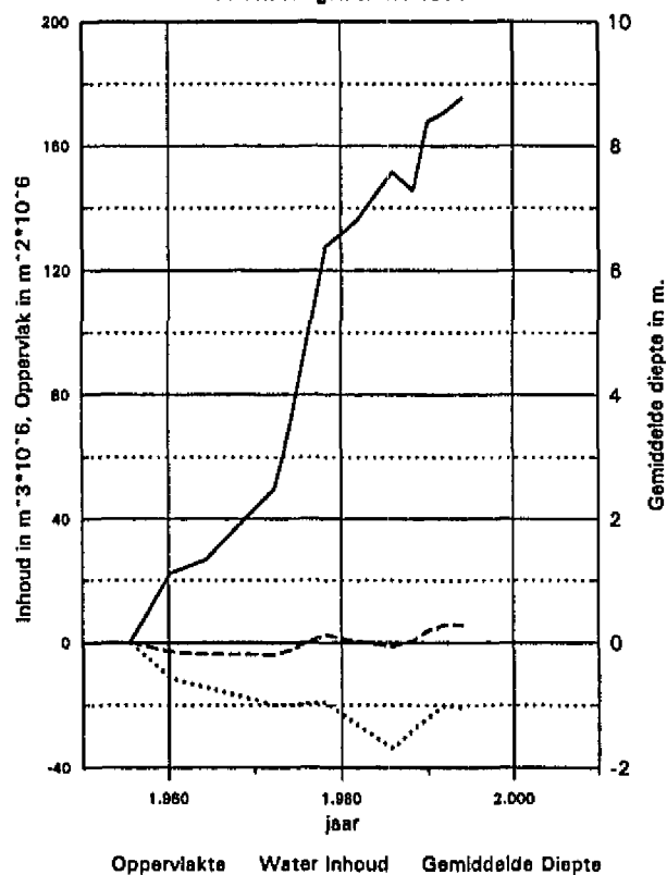
Gehele Westerschelde Hoofd Geulen, onder NAP -2m Veranderingen t.o.v. 1955
