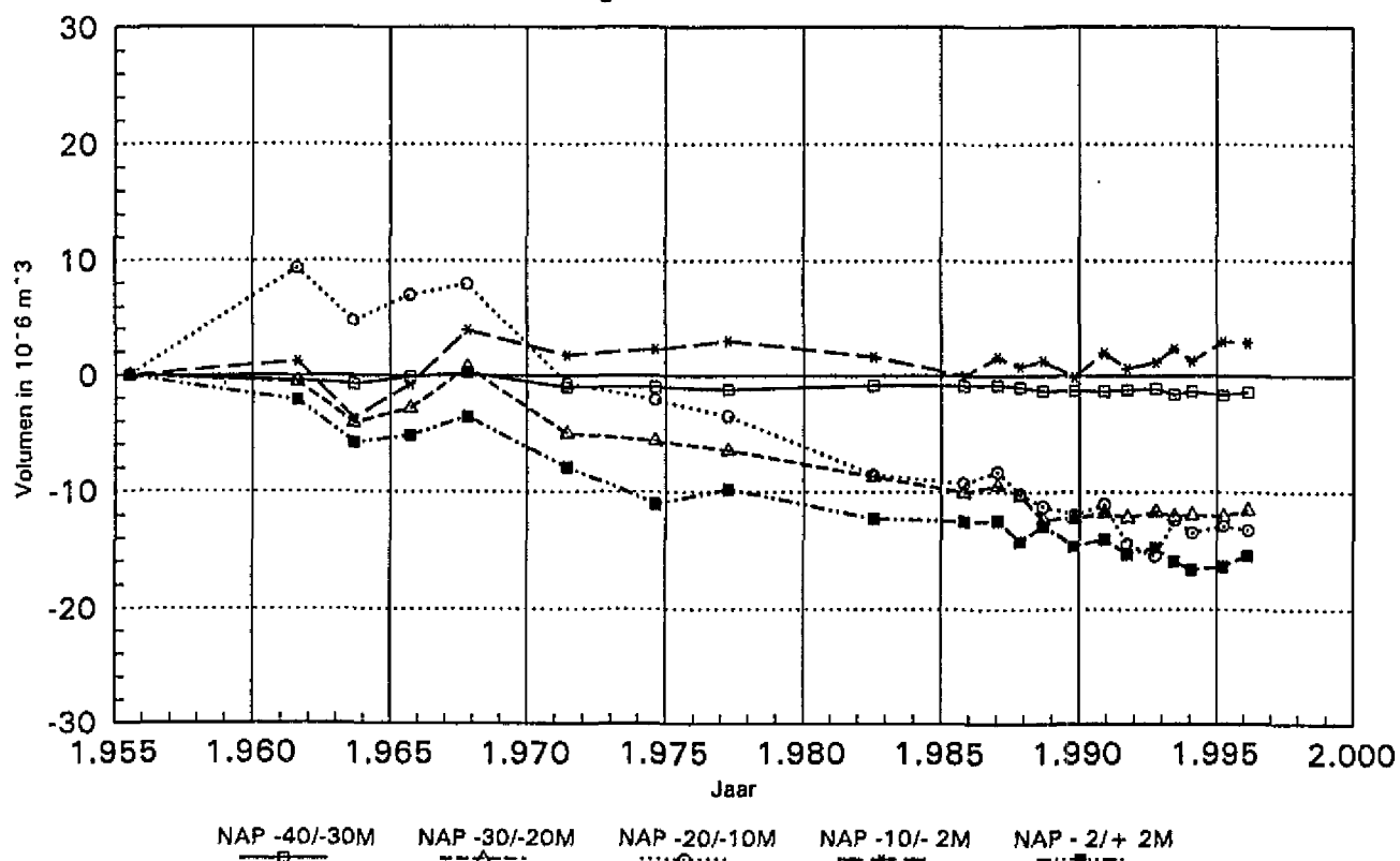
Volumeverandering tussen niveau's t.o.v. 1955
