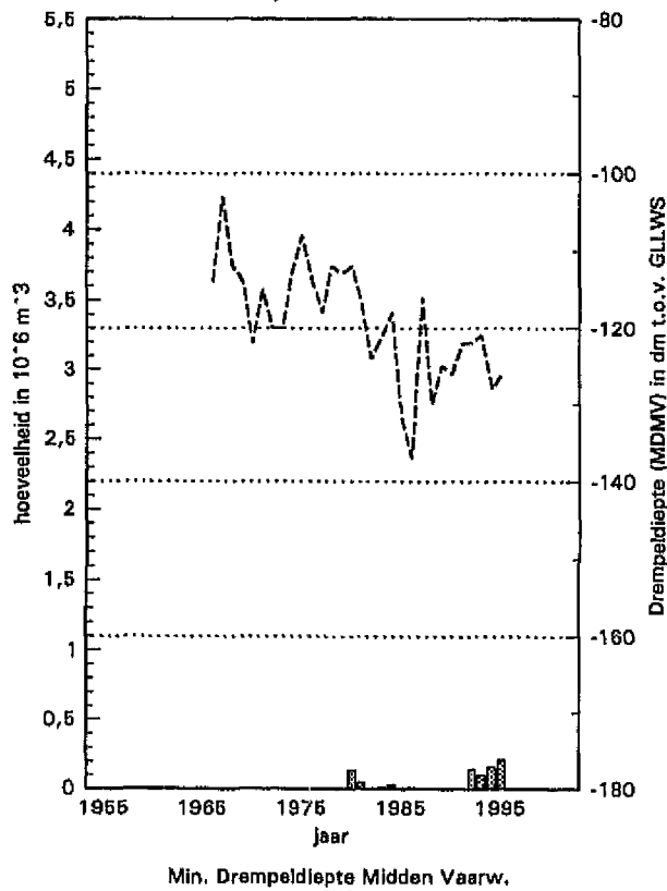
Baggerhoeveelheden en minste Drempeldiepte Gebied 12, Put van Terneuzen
