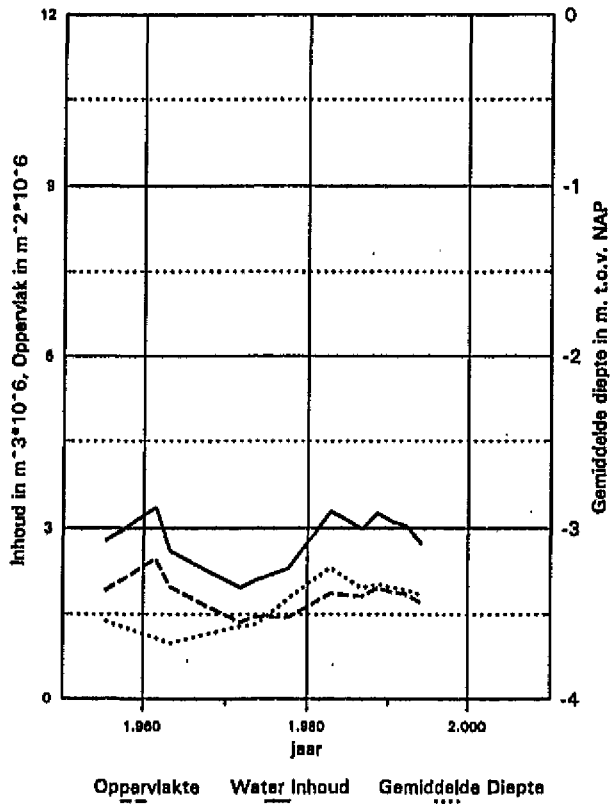
Neven Geul, Appelzak Geulvak 2, ondiepwater, tussen NAP-5m en NAP-2m Verloop in de periode 1955 - 1994
