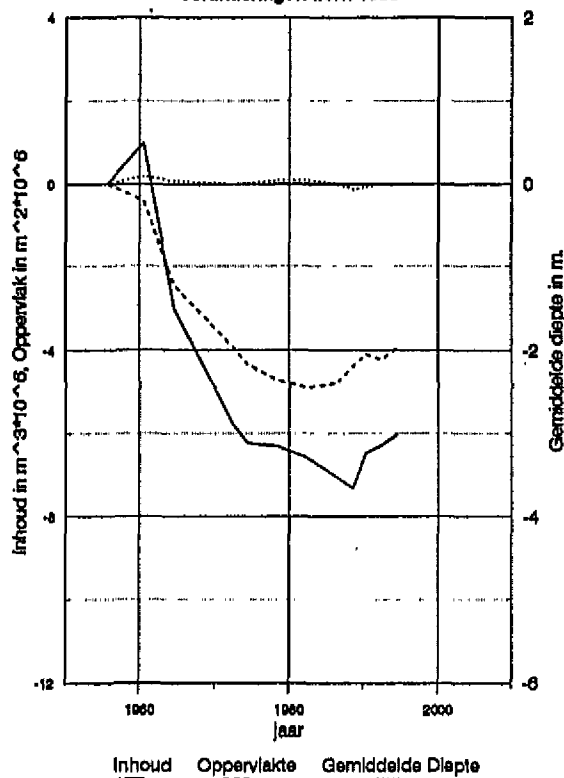
Westelijk deel Westerschelde, Totaal platen Ondiepwatergebied tussen NAP-5m en NAP-2m Veranderingen t.o.v. 1955
