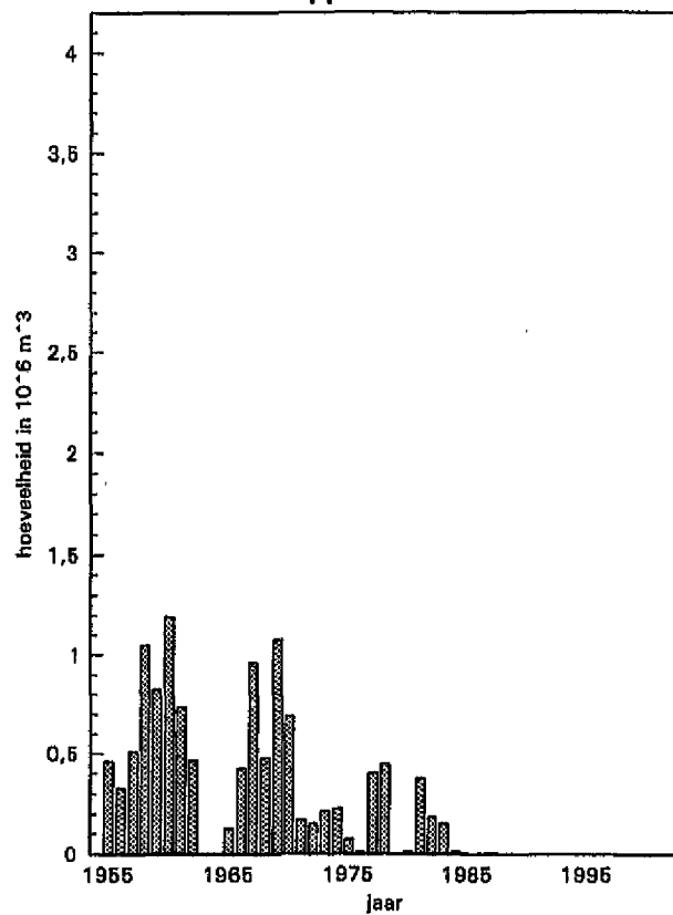
Stortheveelheden Gebied 3 Appelzak
