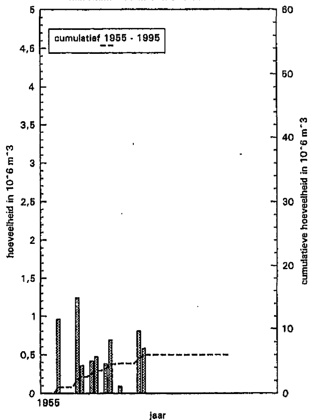
Midden deel Westerschelde Zandwinhoeveelheden t.b.v. Nederland
