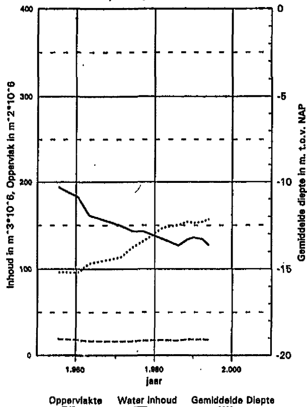
Neven Geul, Middelgat Geulvak 9, onder NAP -5m Verloop in de periode 1955 - 1994
