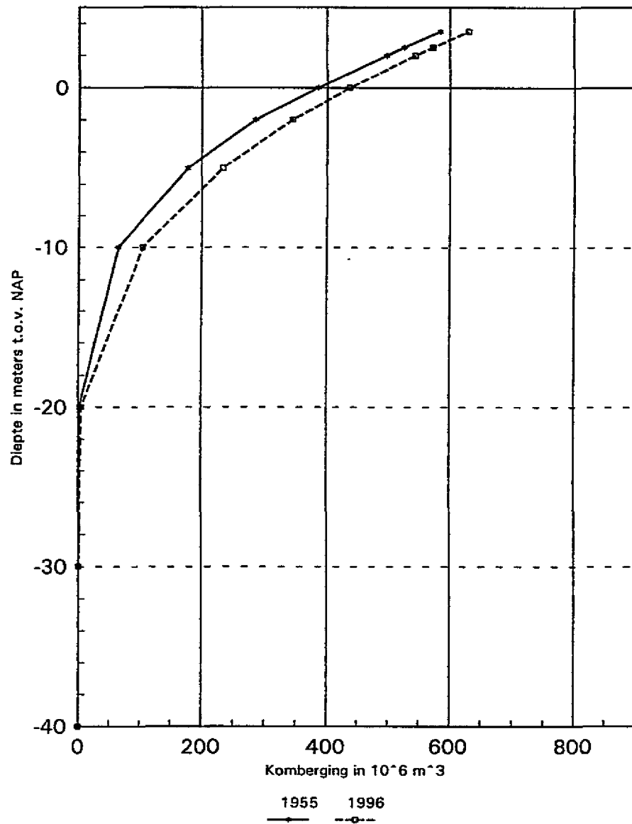
Oostelijk deel Westerschelde Kombergingsgrafieken 1955 en 1996
