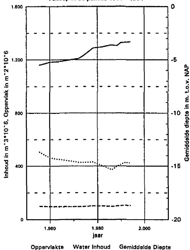
Gehele Westerschelde Hoofd Geulen, onder NAP -2m Verloop in de periode 1955 - 1994
