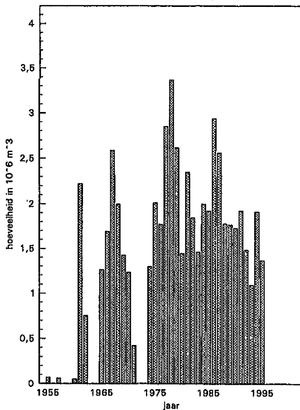
Storthoeveelheden Gebied 8 Baalhoek + Boei 63
