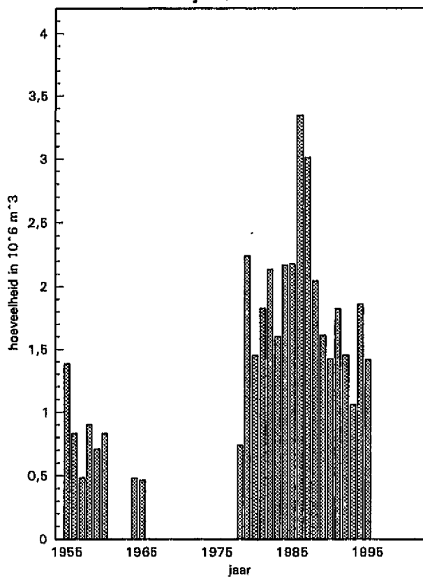
Storthoeveelheden Gebied 7 Konijnenschor
