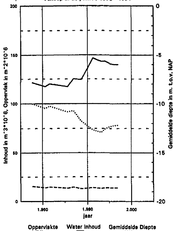
Hoofd Geul, Zuidergat Geulvak 5, onder NAP -2m Verloop in de periode 1955 - 1994
