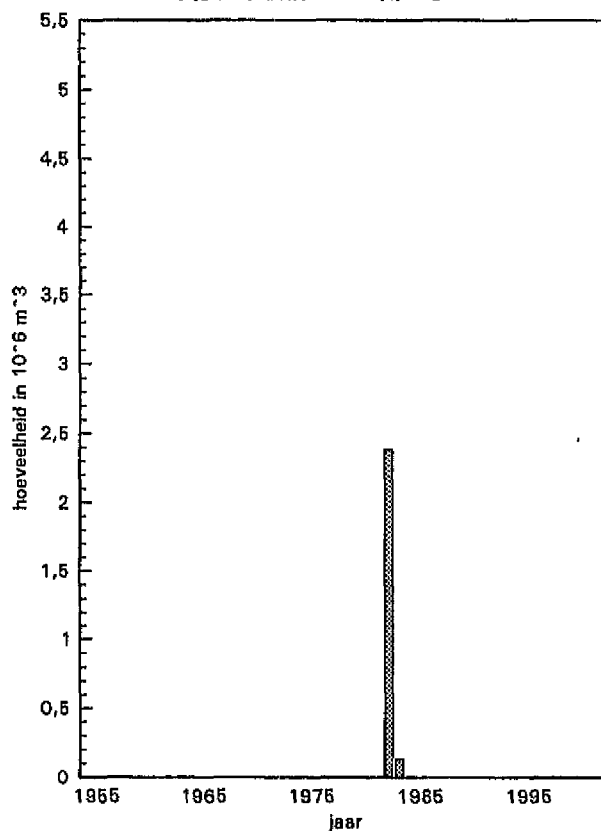
Baggerhoeveelheden Gebied 10 Platen van Ossenisse
