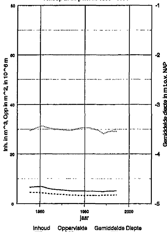
Westelijk deel Westerschelde, Totaal Platen Ondiepwatergebied tussen NAP-5m en NAP-2m Verloop in de periode 1955 - 1994
