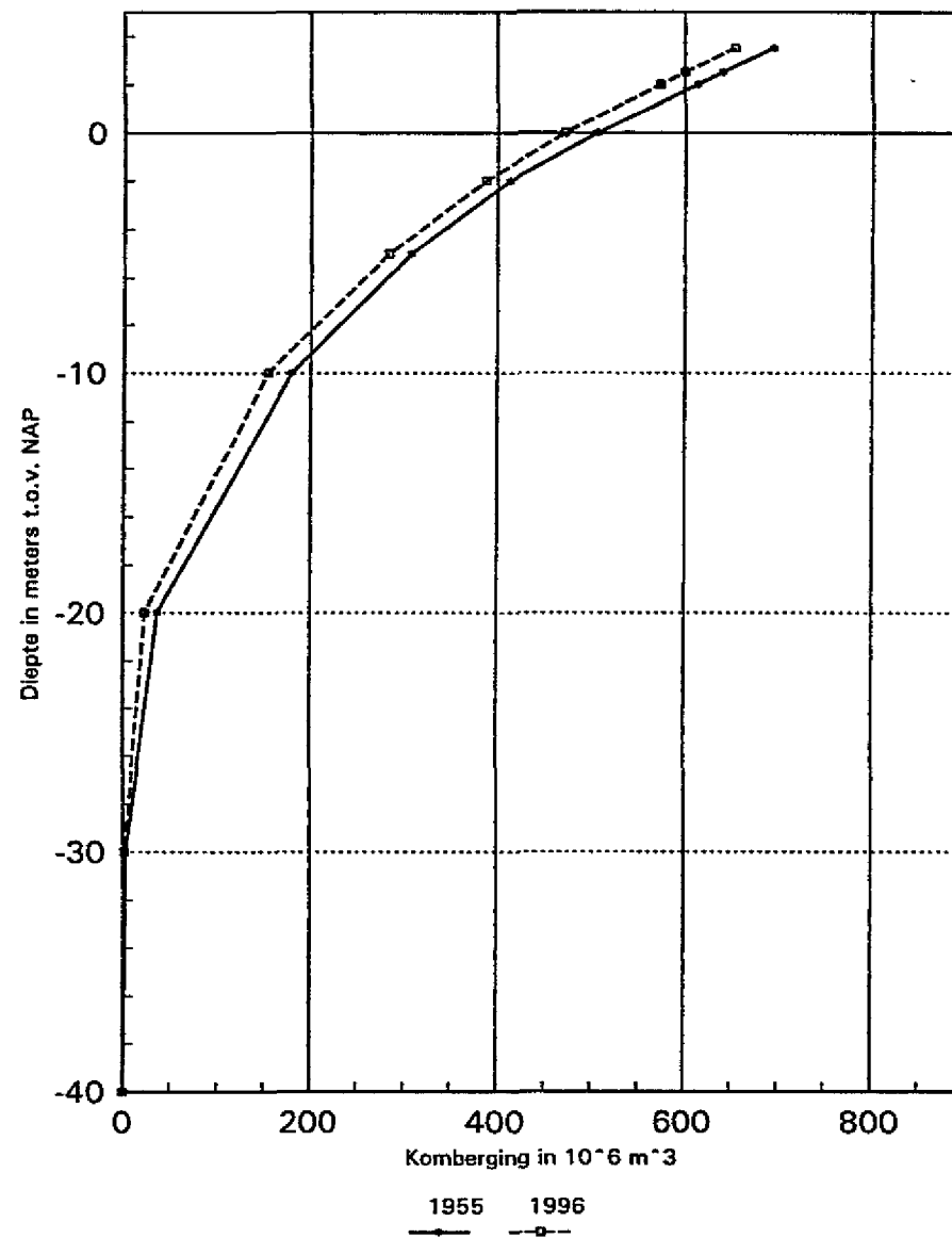
Midden deel Westerschelde Kombergingsgrafieken 1955 en 1996
