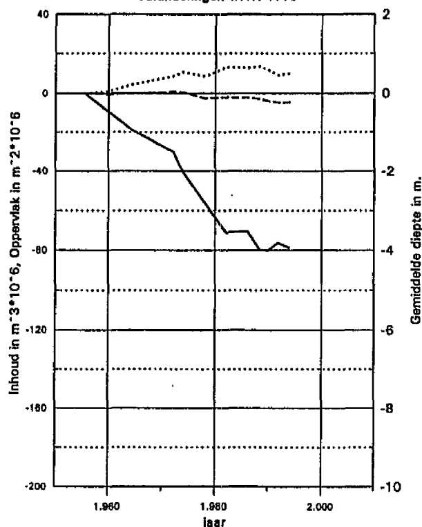
Gehele Westerschelde Neven Geulen, onder NAP -5m Veranderingen t.o.v. 1955
