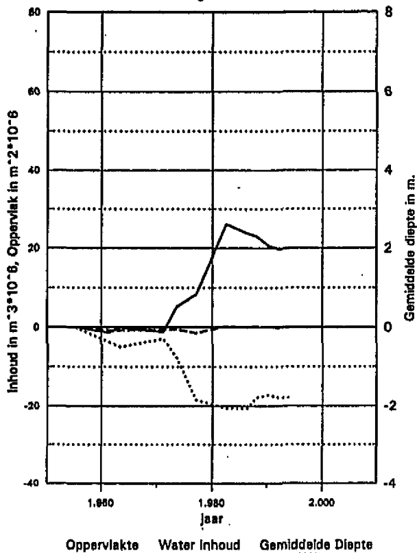
Hoofdgeul, Zuidergat Geulvak 5, onder NAP -5m Veranderingen t.o.v. 1955
