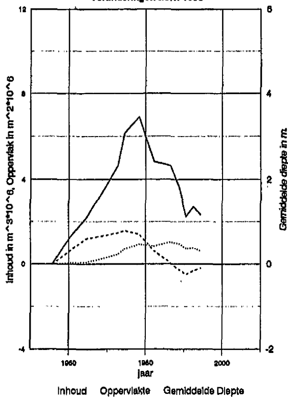
Middelplaten complex Plaatvak 160, boven NAP -2m Veranderingen t.o.v. 1955
