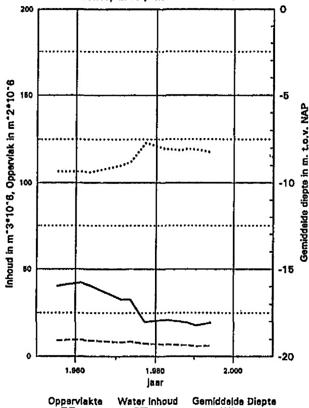
Neven Geul, Schaar van Valkenisse Geulvak 6, onder NAP -5m Verloop in de periode 1955 - 1994
