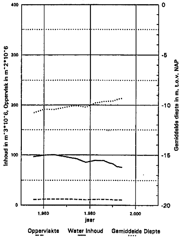
Neven Geul, Vaarwater langs Hoofdplaat Geulvak 14, onder NAP -2m Verloop in de periode 1955 - 1994
