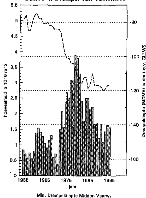
Baggerhoeveelheden en minste Drempeldiepte Gebied 4, Drempel van Valkenisse
