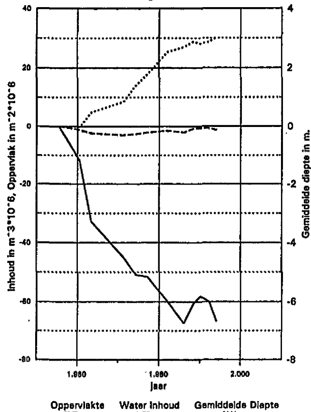
Neven Geul, Middelgat Geulvak 9, onder NAP -5m Veranderingen t.o.v. 1955
