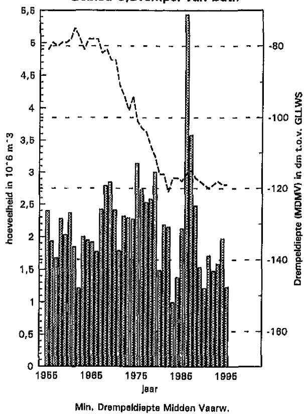
Baggerhoeveelheden en minste Drempeldiepte Gebied 3, Drempel van Bath
