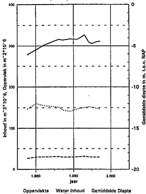
Neven Geul, Everingen Geulvak 13, onder NAP -2m Verloop in de periode 1955 - 1994
