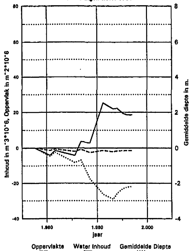
Hoofdgeul, Zuidergat Geulvak 5, onder NAP -2m Veranderingen t.o.v. 1955
