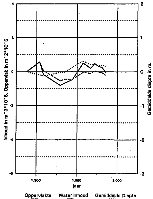
Neven Geul, Appelzak Geulvak 2, ondiepwater, tussen NAP-5m en NAP-2m Veranderingen t.o.v. 1955
