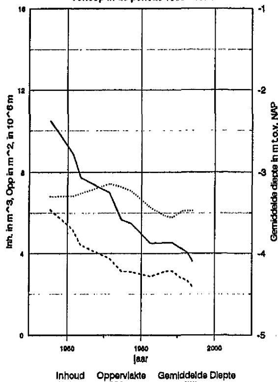
Rug van Baarland, plaatvak 140 Ondiepwatergebied tussen NAP-5m en NAP-2m Verloop in de periode 1955 - 1994
