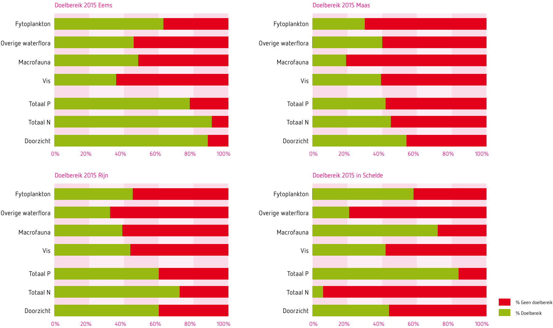
Figuur 8 Percentage waterlichamen per stroomgebied dat in 2015 de doelen haalt voor de biologische parameters
