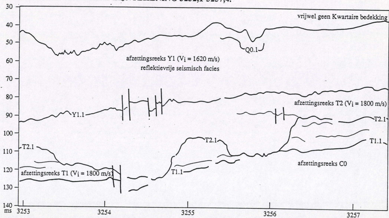
Figuur 37. Seismisch profiel in het noorden van het studiegebied, dat de geulopvullingsstructuren weergeeft in de T2-afzettingenreeks.
