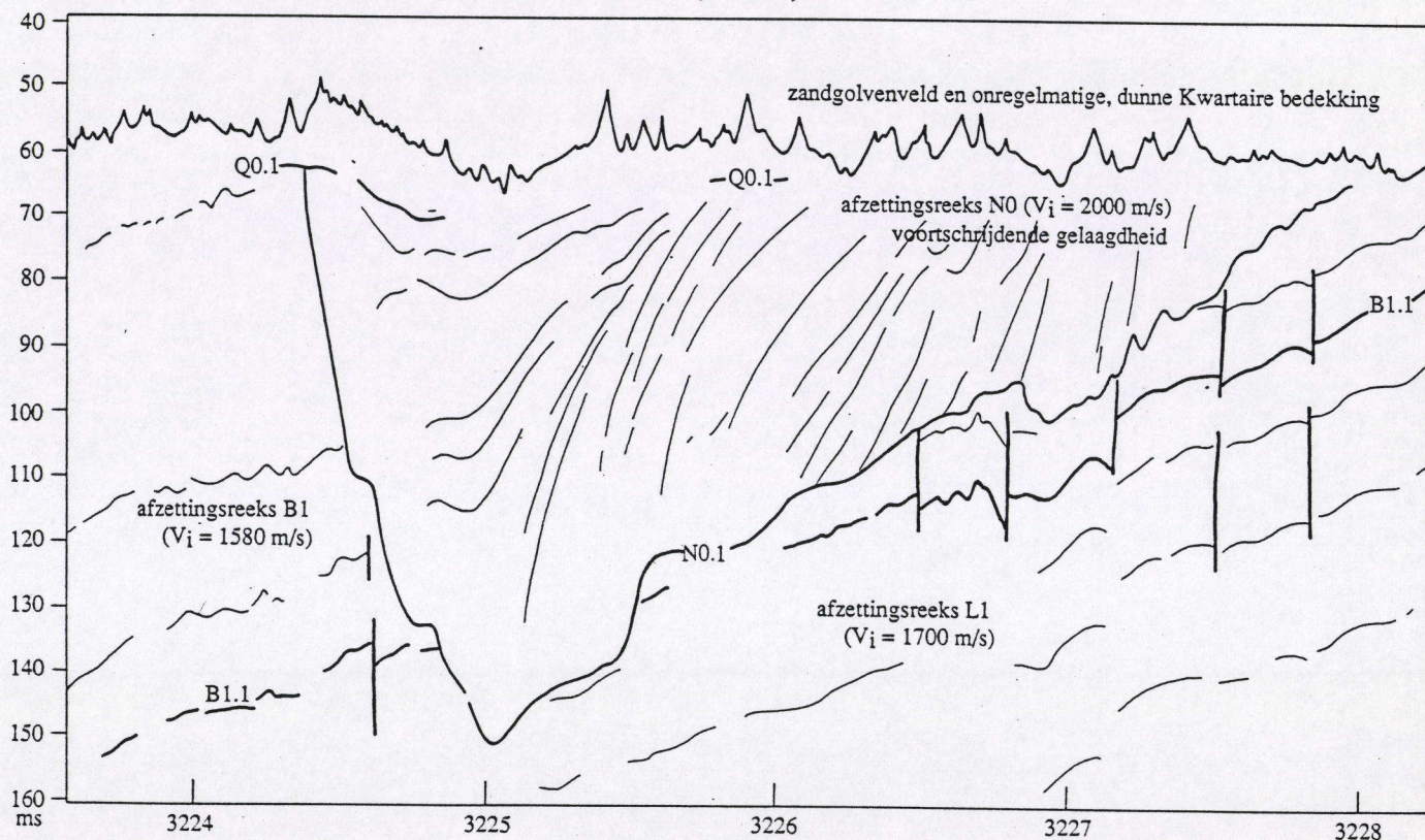
Figuur 92. Seismisch profiel in het noorden van het studiegebied, dat de met de N0-afzettingenreeks opgevulde Murray Pit weergeeft.
