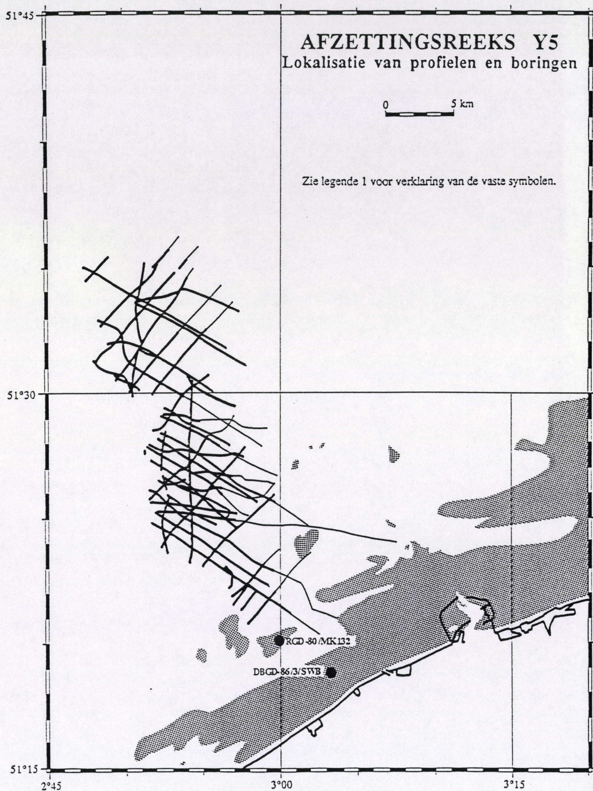
Figuur 58. - Seismostratigrafische interpretatiekaart. Afzettingsreeks Y5 : lokalisatie van bij de interpretatie gebruikte profielen en boringen (zie ook Legende 1). Mercatorprojectie op 51°20'.
