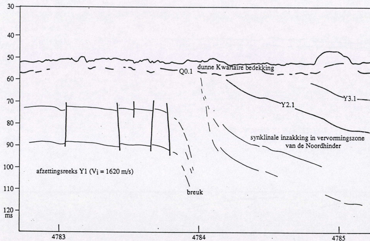
Figuur 132. Seismisch profiel doorheen de vervormingszone van de Noordhinder, dat een door een breuk geflankeerde synklinale inzakking in de Y1-afzettingenreeks weergeeft.
