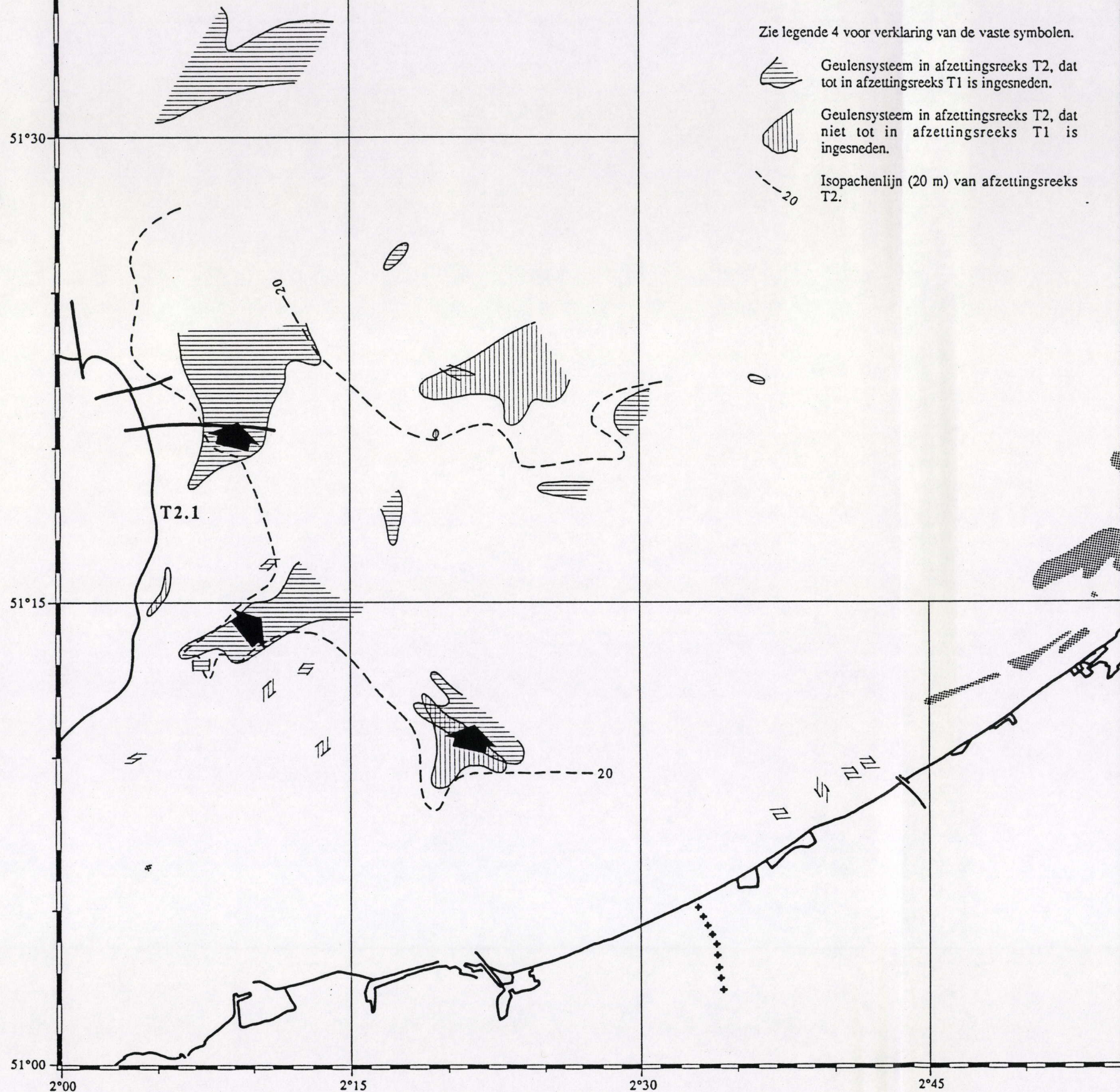
Figuur 36. Seismostratigrafische interpretatiekaart. Afzettingenreeks T2 : kenmerken van het seismisch facies (zie ook Legende 4). Mercatorprojectie op 51° 20'.
