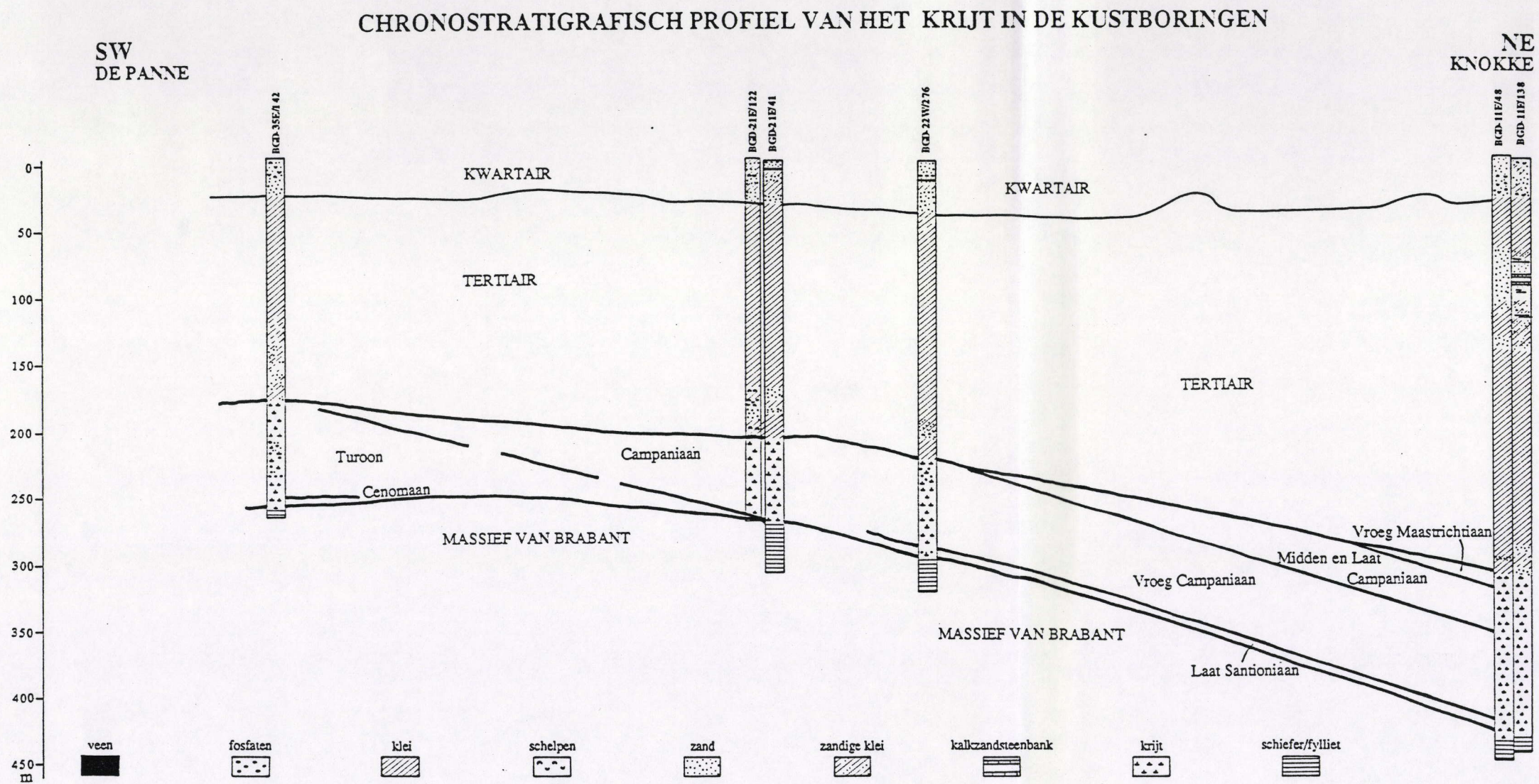
Figuur 100. Chronostratigrafisch profiel van de Krijt-afzettingen doorheen de kustboringen (naar : LAGA & VANDENBERGHE, 1989).
