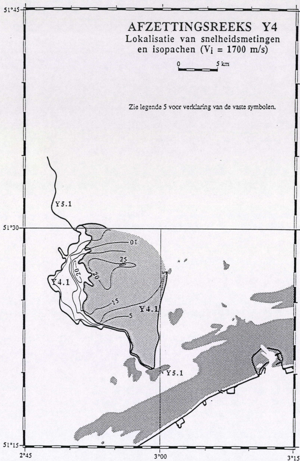
Figuur 56. Seismostratigrafische interpretatiekaart. Afzettingenreeks Y4 : lokalisatie van snelheidsmetingen en diktekaart (zie ook Legende 5). Diktes werden berekend met een seismische intervalsnelheid van 1700 m/s. Mercatorprojectie op 51°20'.
