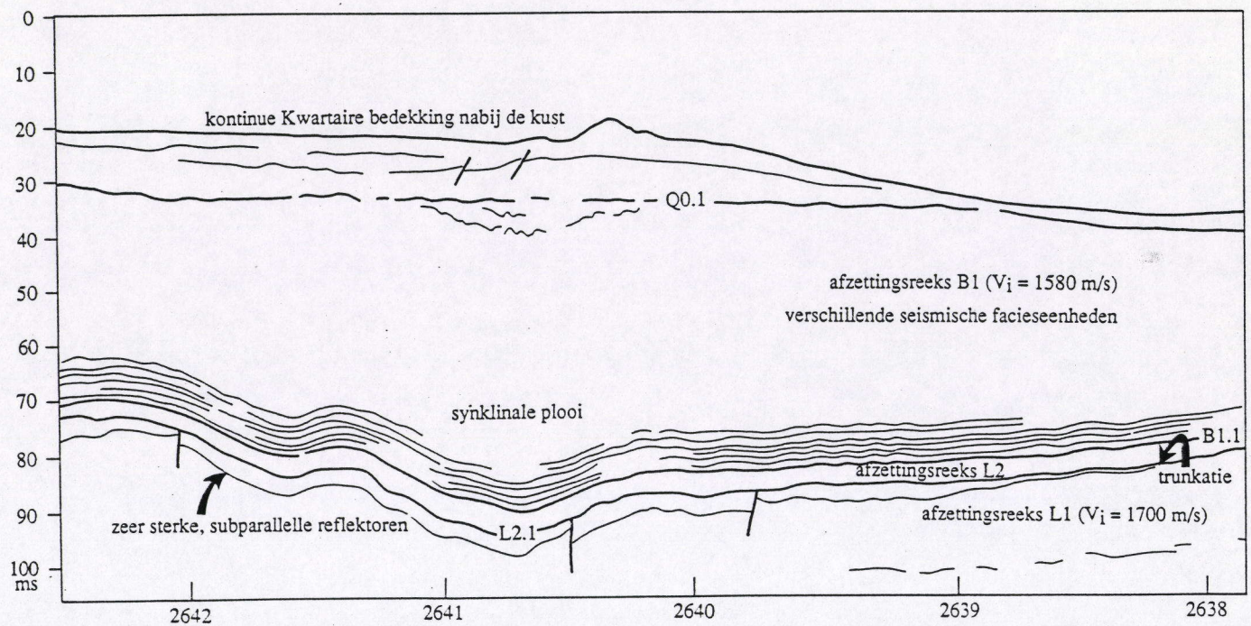
Figuur 66. Seismisch profiel vóór de Belgische oostkust, dat de erosieve trunkatie aan de top van de L1-afzettingsreeks, de slechts plaatselijk identificeerbare L2-afzettingsreeks en verschillende seismische facieseenheden in de B1-afzettingsreeks weergeeft.
