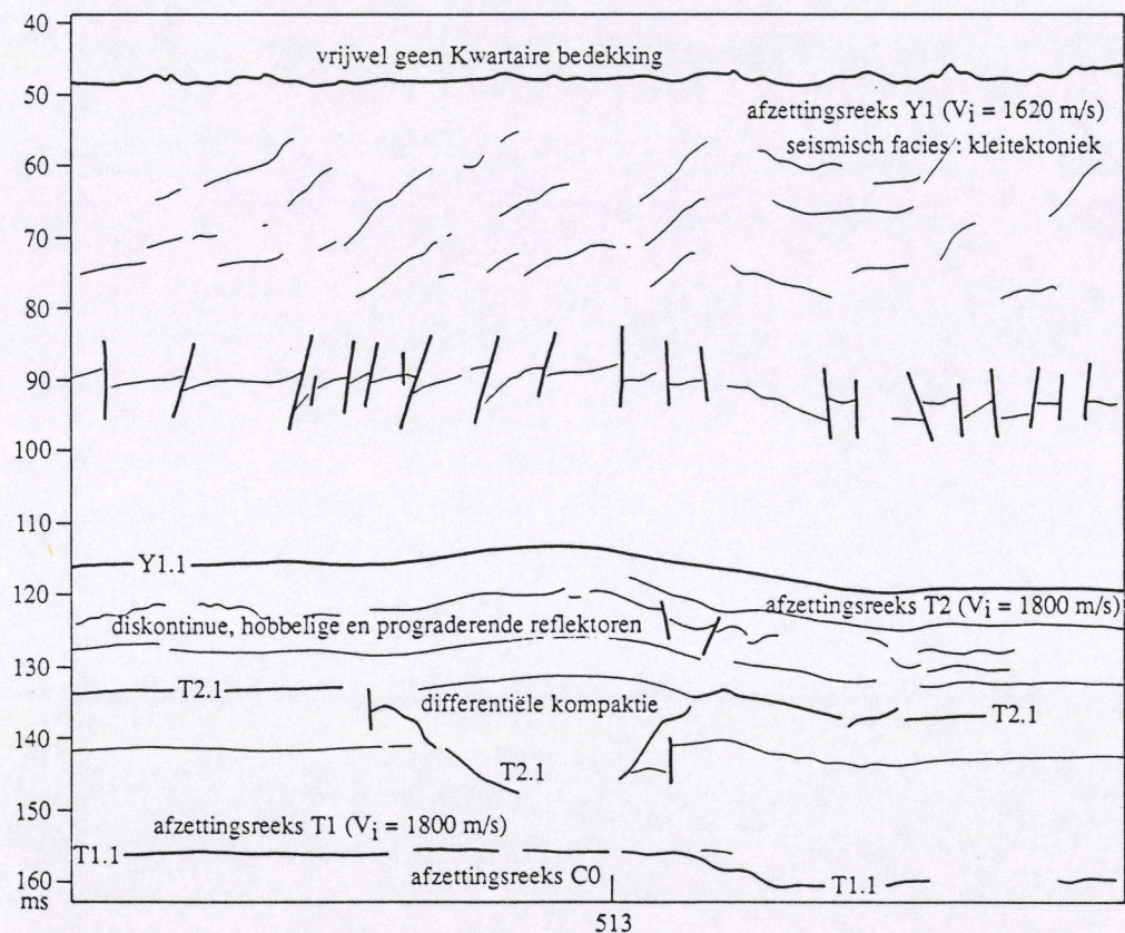
Figuur 98. Seismisch profiel in het centrale deel van het studiegebied, dat differentieel gekompakteerde geulopvullingsstructuren in de T2-afzettingsreeks weergeeft.
