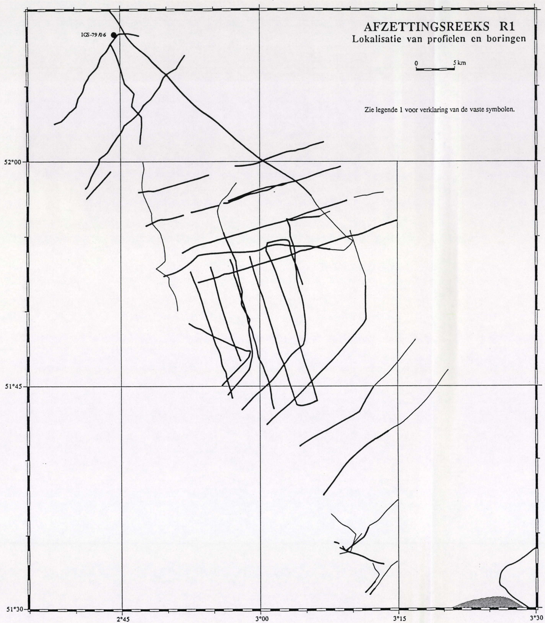
Figuur 79. Seismostratigrafische interpretatiekaart. Afzettingsreeks R1 : lokalisatie van bij de interpretatie gebruikte profielen en boringen (zie ook Legende 1). Mercatorprojectie op 51°20'.
