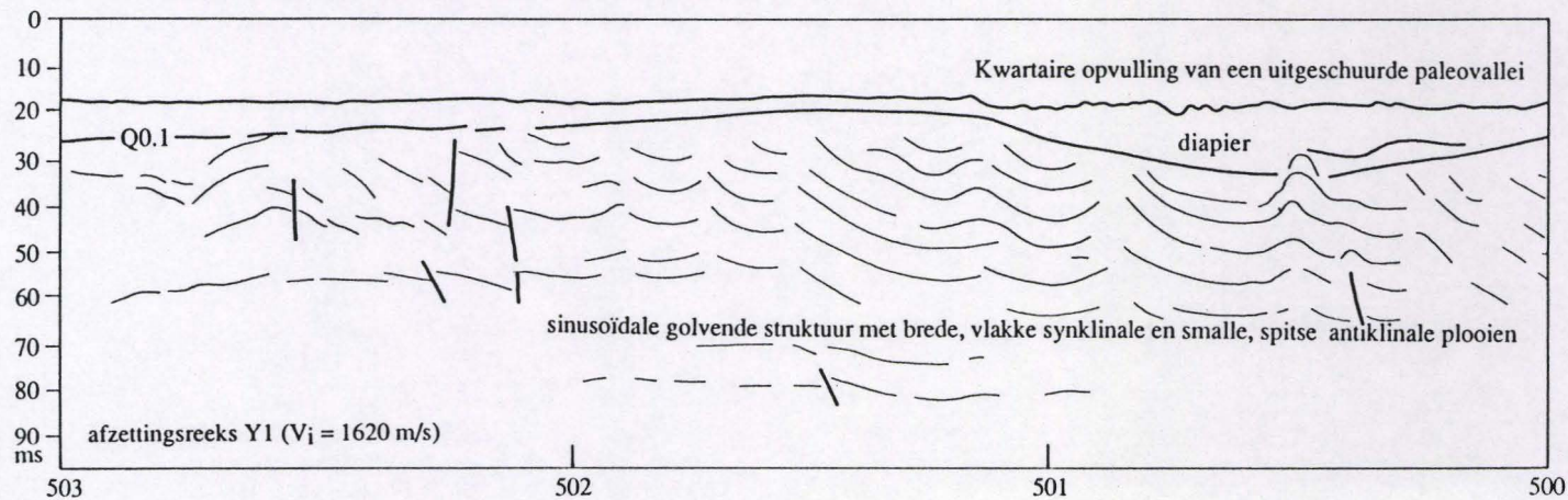
Figuur 111. Seismisch profiel in het centrale deel van het studiegebied, dat een sinusoidale, golvende vervorming en diapierachtige structuren in het middenste interval van de Y1-afzettingenreeks weergeeft.
