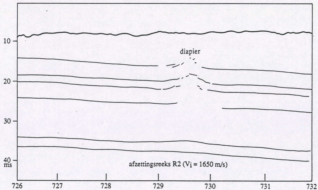
Figuur 129. Seismisch profiel op de Schelde in de buurt van Antwerpen, dat kleidiapierisme in de R2- afzettingenreeks weergeeft.
