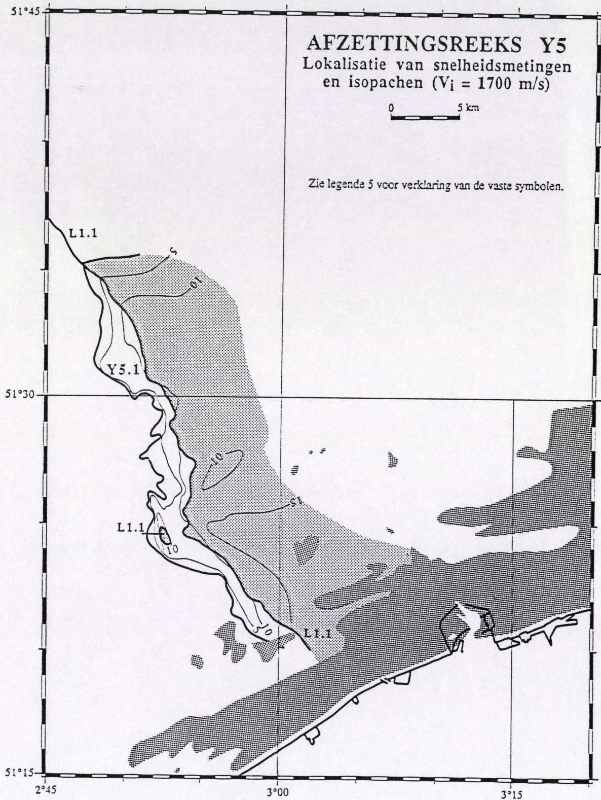
Figuur 62. Seismostratigrafische interpretatiekaart. Afzettingsreeks Y5 : lokalisatie van snelheidsmetingen en diktekaart (zie ook Legende 5). Diktes werden berekend met een seismische intervalsnelheid van 1700 m/s. Mercatorprojectie op 51°20'.
