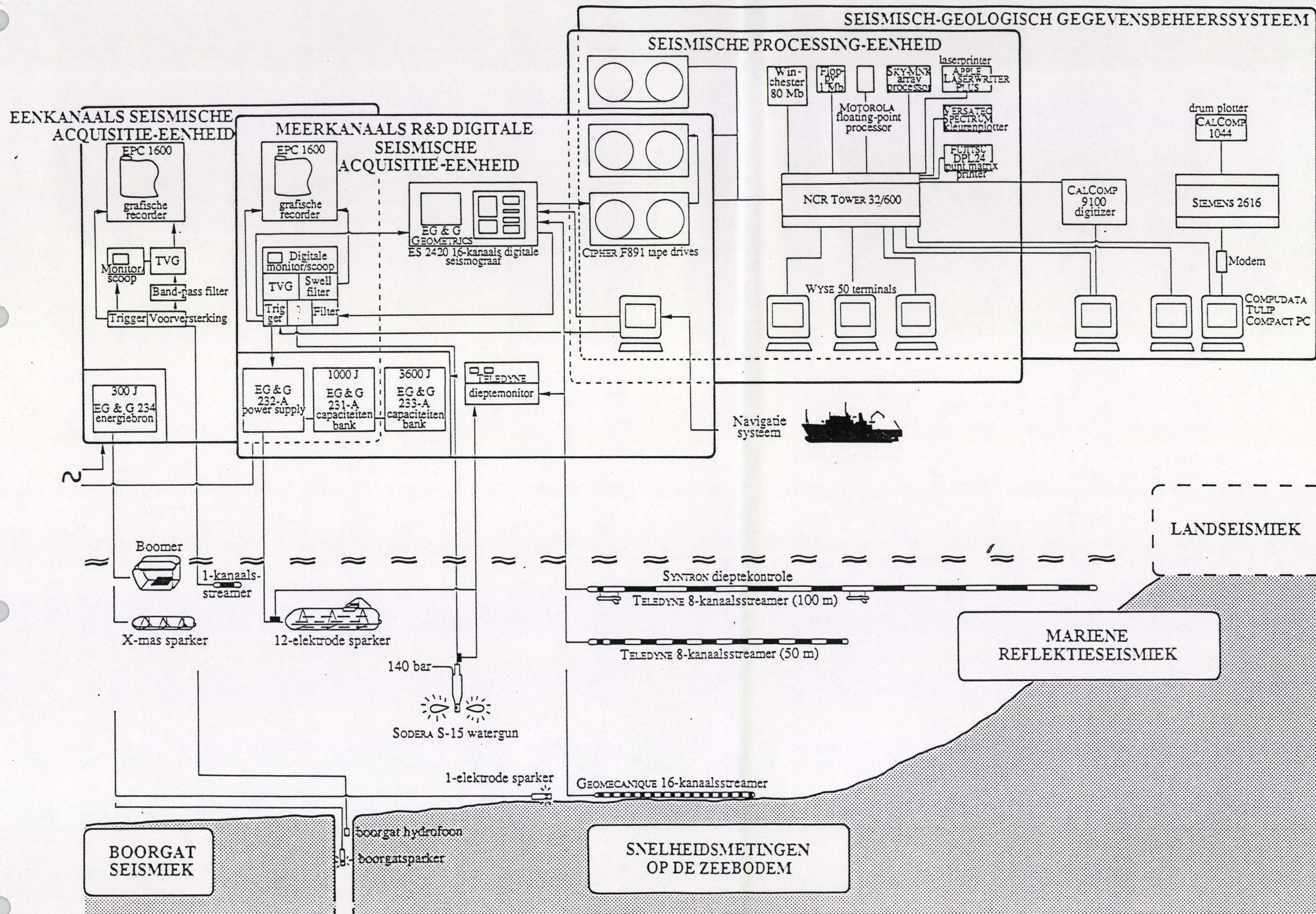
Figuur 4. Schematisch overzicht van het seismisch systeem van het RCMG.
