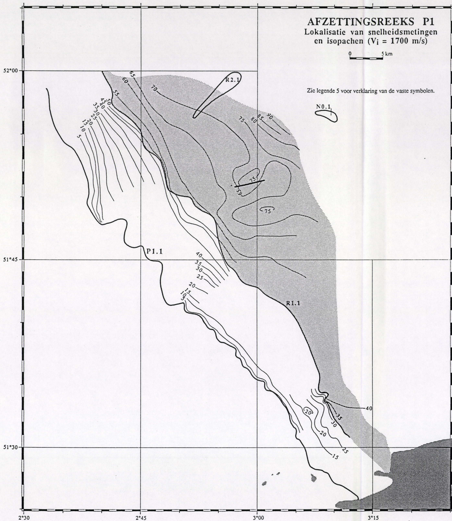
Figuur 78. Seismostratigrafische interpretatiekaart. Afzettingsreeks P1 : lokalisatie van snelheidsmetingen en diktekaart (zie ook legende 5). Diktes werden berekend met een seismische intervalsnelheid van 1700 m/s. Mercatorprojectie op 51°20'.
