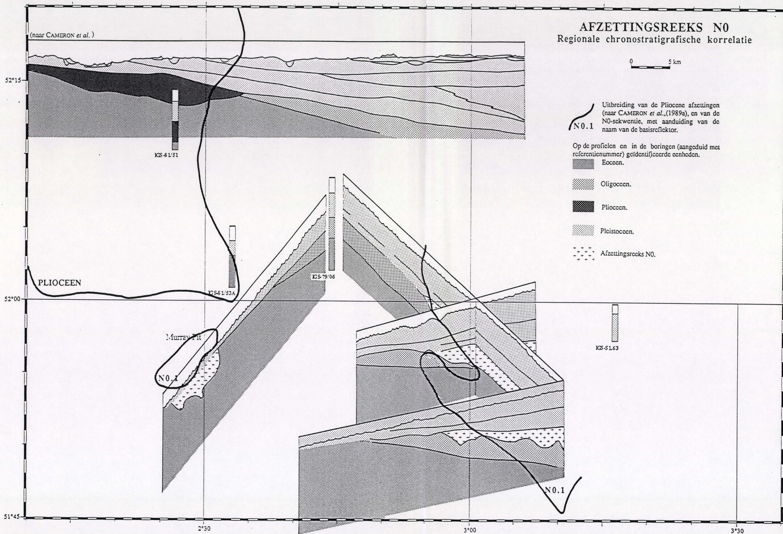
Figuur 93. Regionale chronostratigrafische korrelatie van de N0-afzettingsreeks. Mercatorprojectie op 51°20'. Door vergelijking met naburige geologische informatie uit boringen, geïnterpreteerde profielen (CAMERON et al. , 1989a) en geologische kaarten (CAMERON et al. , 1989a) kan afgeleid worden dat de N0-afzettingsreeks vermoedelijk van Pliocene ouderdom is.
