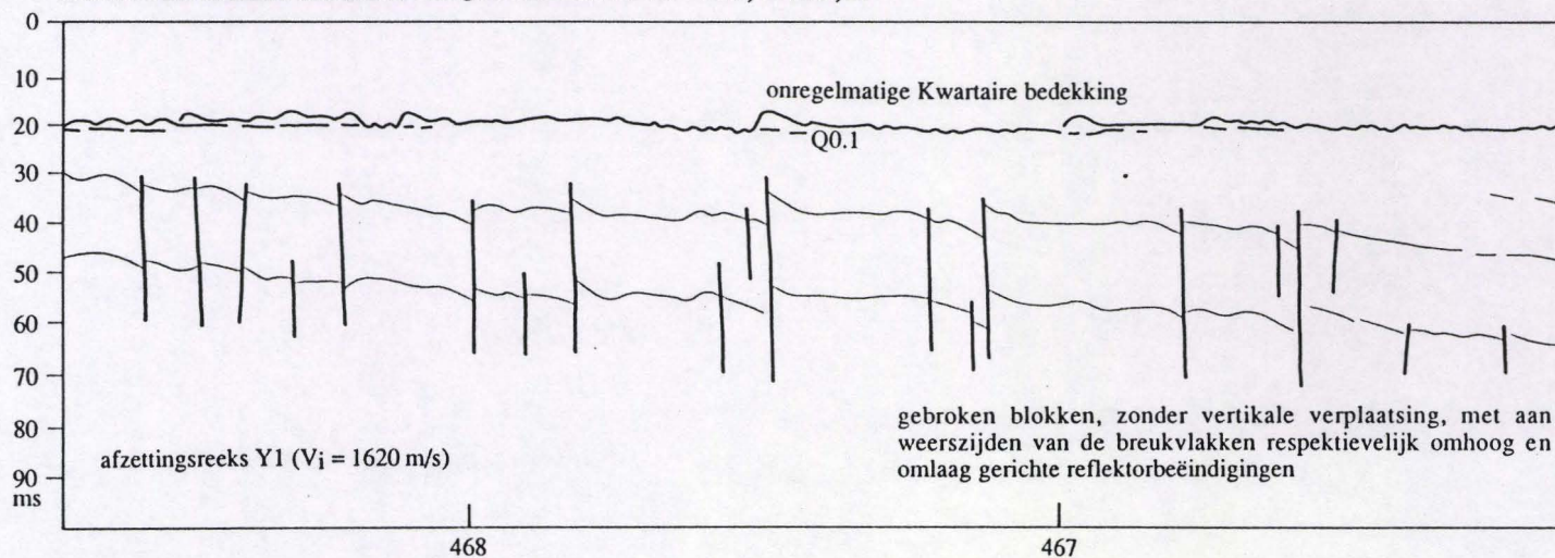
Figuur 114. Seismisch profiel in het centrale deel van het studiegebied, dat de kenmerkende sedimenttektonische vervormingsstijl helemaal bovenaan in de Y1-afzettingsreeks weergeeft.
