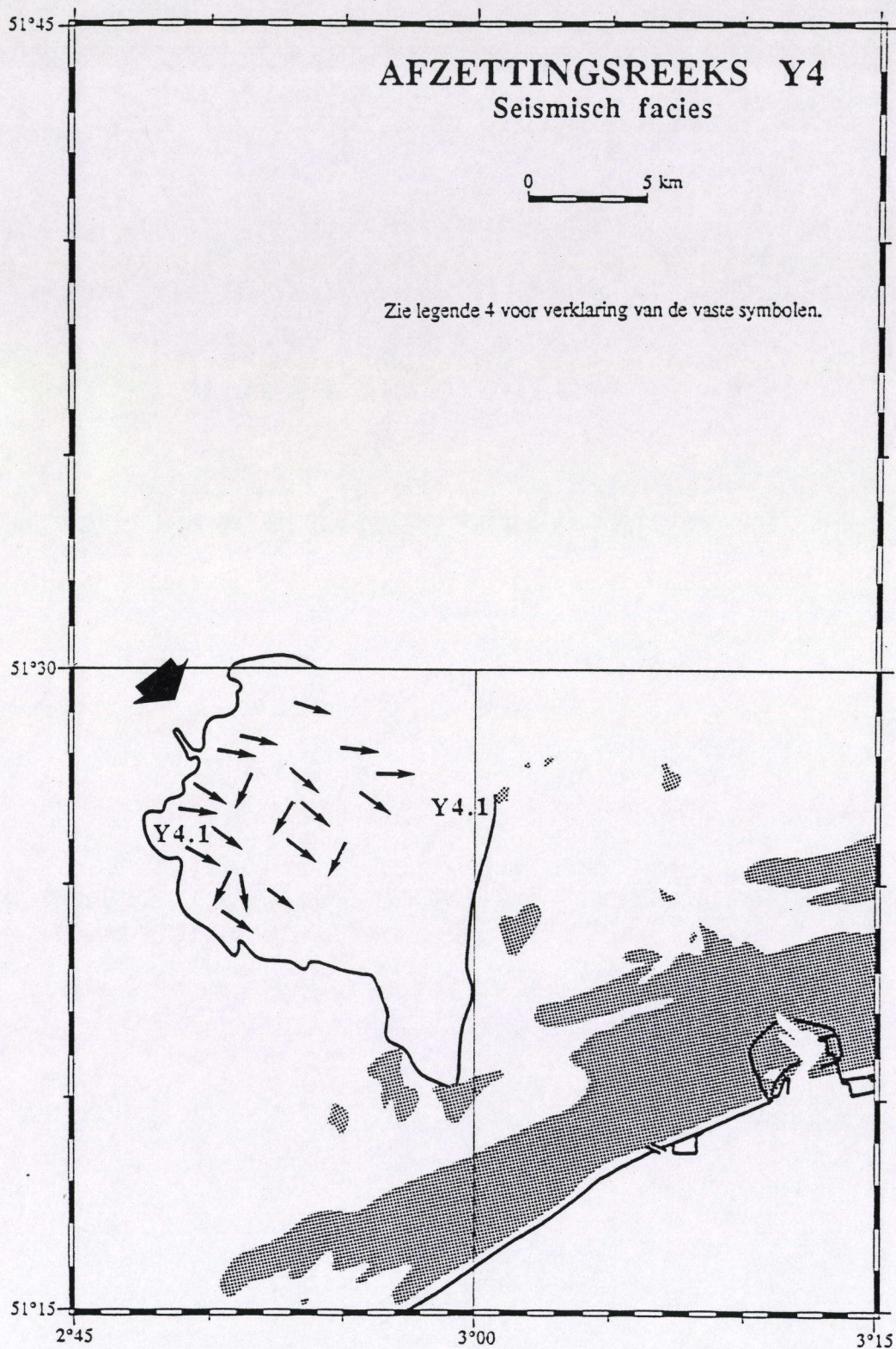
Figuur 55. Seismostratigrafische interpretatiekaart. Afzettingsreeks Y4 : kenmerken van het seismisch facies (zie ook Legende 4). Mercatorprojectie op 51°20'.
