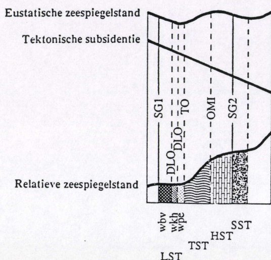
Figuur 14. Relatie tussen eustatische zeespiegelschommelingen, subsidentiesnelheid, sedimentaanvoer en de opeenvolging van verschillende systems tracts en oppervlakken binnen een afzettingsreeks (naar : VAIL, 1987 ; VAIL et al., 1987).
