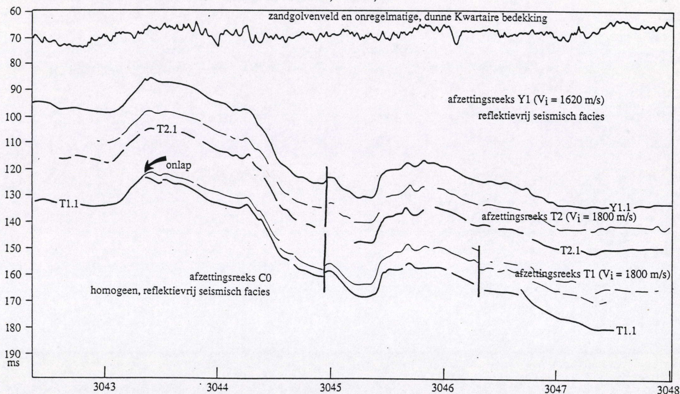
Figuur 28. Seismisch profiel in het noordwesten van het studiegebied, dat de onlap-configuratie weergeeft van de T1-afzettingenreeks tegen het post-Mesozoische erosieoppervlak.
