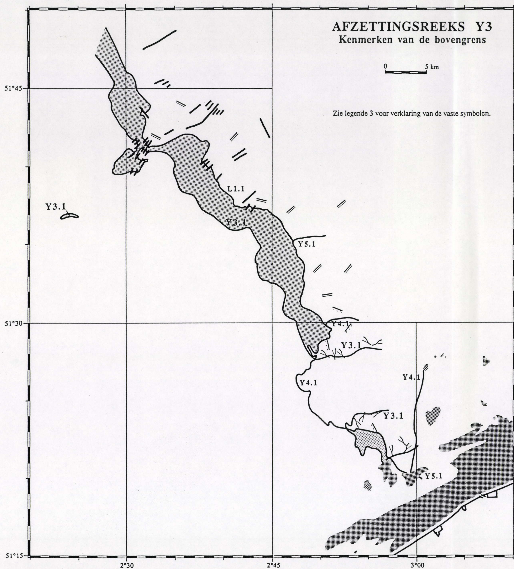
Figuur 49. Seismostratigrafische interpretatiekaart. Afzettingsreeks Y3 : Reflektorkonfiguraties ten opzichte van de bovengrens (zie ook Legende 3). Mercatorprojectie op 51°20'.
