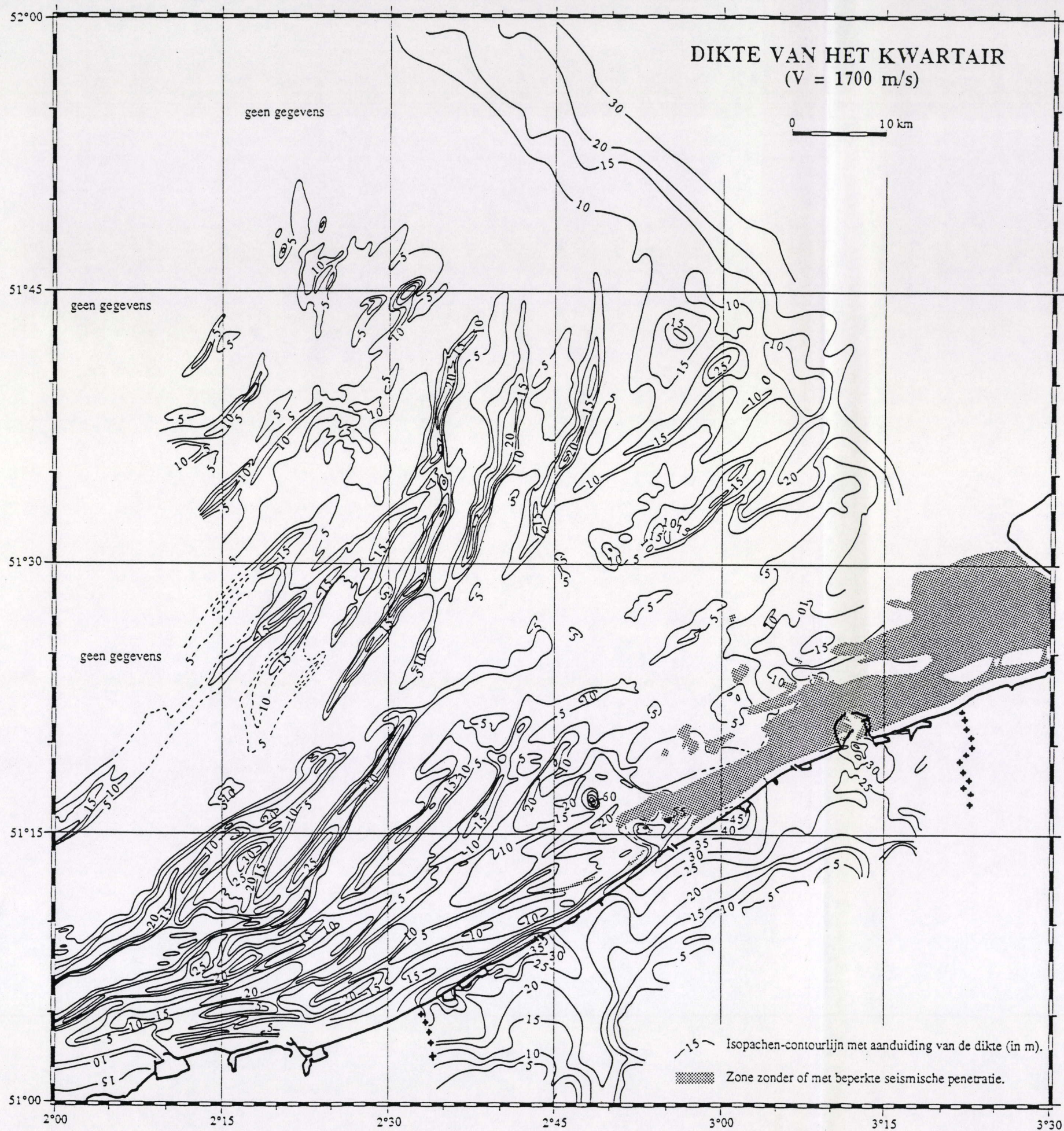
Figuur 97. Diktekaart van de Kwartaire afzettingen. Mercatorprojectie op 51° 20'. Diktes werden berekend aan de hand van een gemiddelde seismische snelheid van 1700 m/s. Landgedeelte gecompileerd naar : BAETEMAN (1981), DE BREUCK & DE MOOR (1974), DEPRET (1983), DEVOS (1984), MOSTAERT (1985) en SOMME (1979).
