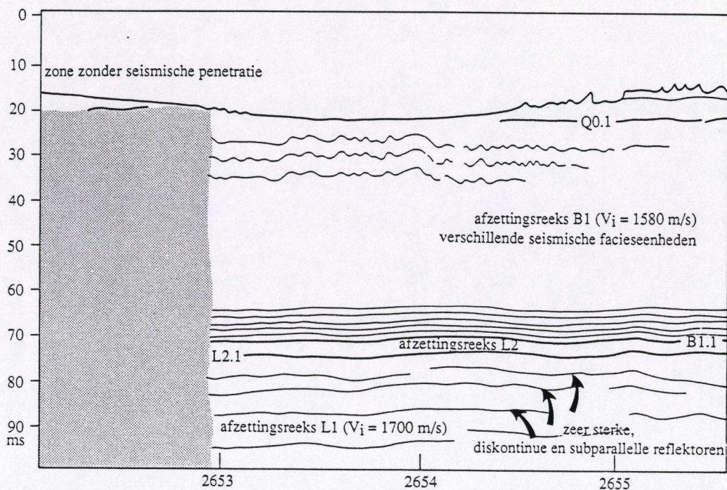
Figuur 67. Seismisch profiel vóór de Belgische oostkust, dat de slechts plaatselijk identificeerbare L2-afzettingenreeks, verschillende seismische facieseenheden in de B1-afzettingenreeks en een zone zonder seismische penetratie weergeeft.
