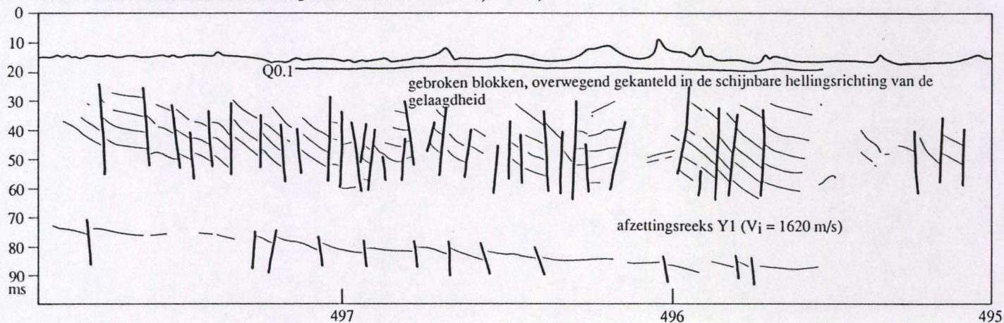
Figuur 112. Seismisch profiel in het centrale deel van het studiegebied, dat gebroken en preferentieel in de hellingsrichting gekantelde blokken in het bovenste interval van de Y1-afzettingenreeks weergeeft.
