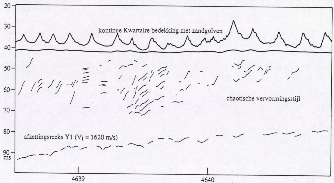
Figuur 108. Seismisch profiel in het centrale deel van het studiegebied, dat een chaotische sedimenttektonische vervormingsstijl in de Y1-afzettingenreeks weergeeft.
