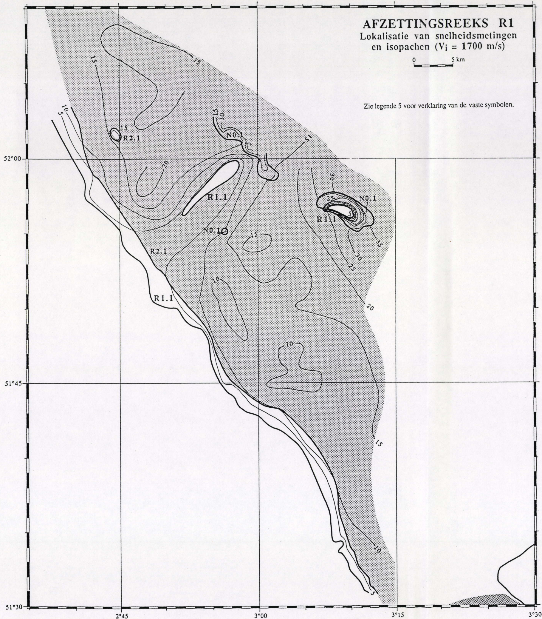
Figuur 83. Seismostratigrafische interpretatiekaart. Afzettingsreeks R1 : lokalisatie van snelheidsmetingen en diktekaart (zie ook legende 5). Diktes werden berekend met een seismische interval snelheid van 1700 m/s. Mercatorprojectie op 51°20'.
