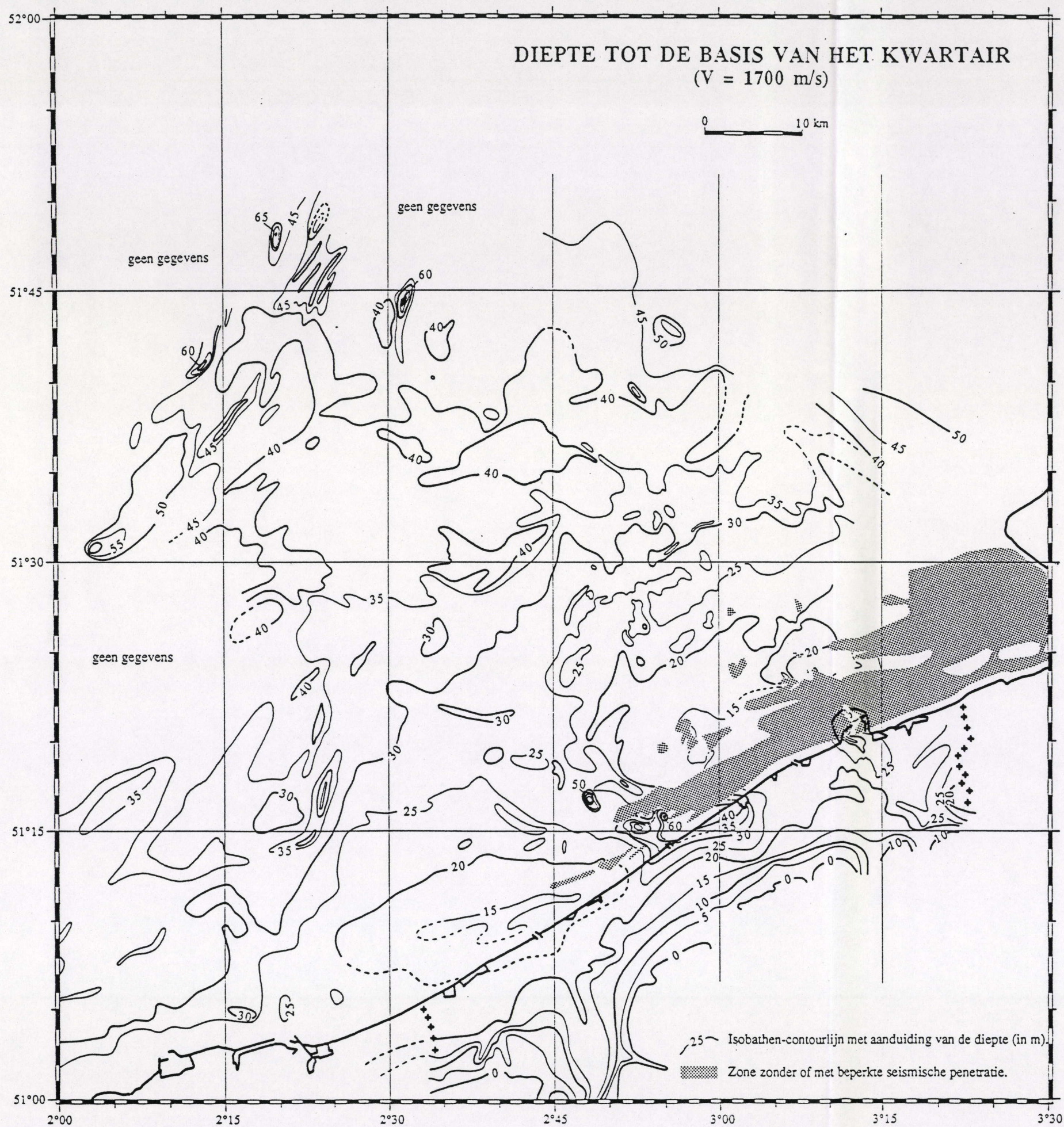
Figuur 20. Dieptekaart tot de basis van de Kwartaire afzettingen. Mercatorprojectie op 51°20'. Referentieniveau : MLLWS. Diepten werden berekend aan de hand van een gemiddelde seismische snelheid van 1700 m/s. Landgedeelte gekompileerd naar : BAETEMAN (1981), DE BREUCK & DE MOOR (1974), DEPRET (1983), DEVOS (1984), MOSTAERT (1985) en SOMME (1979).
