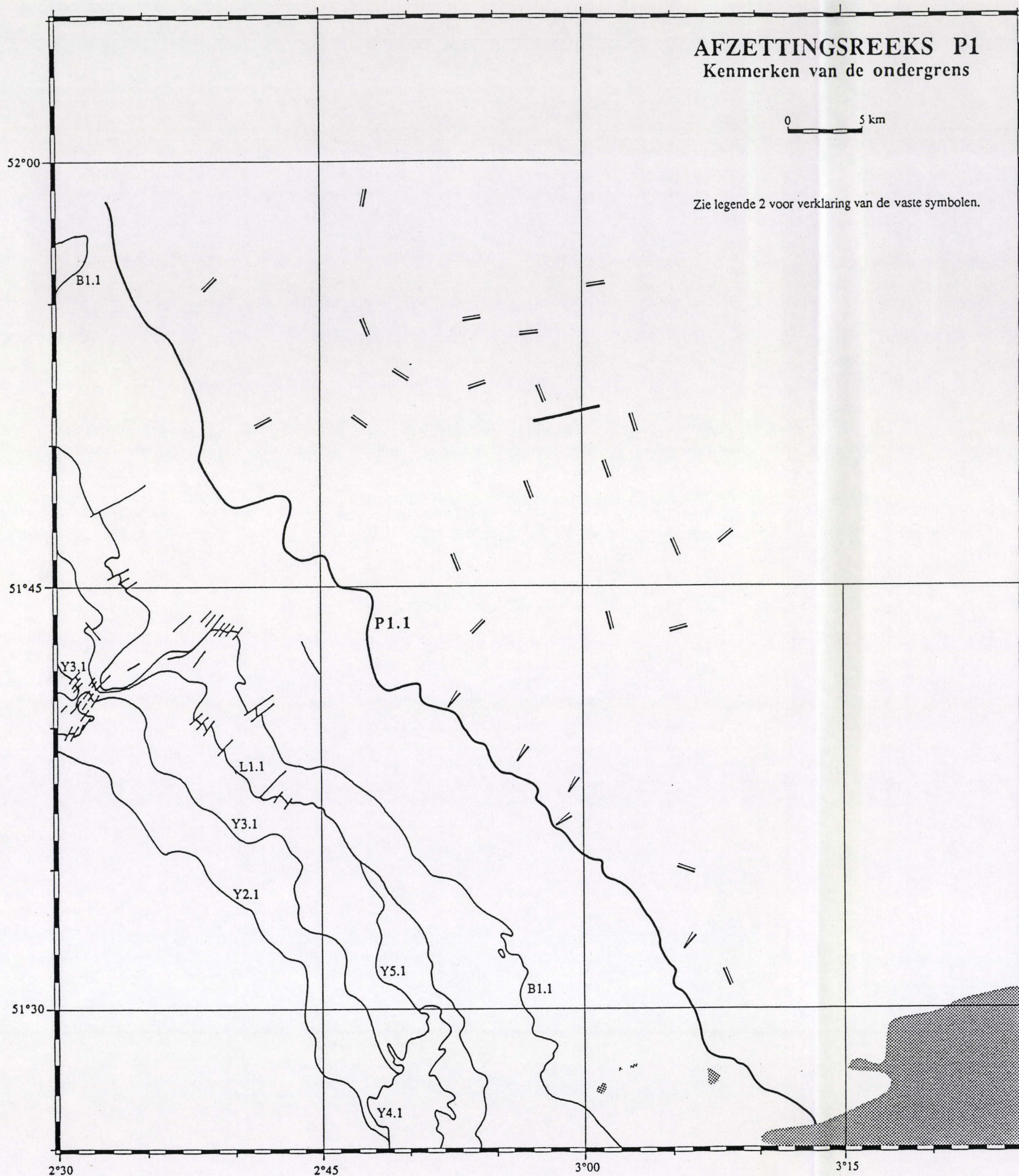
Figuur 76. Seismostratigrafische interpretatiekaart. Afzettingsreeks P1 : Reflektorkonfiguraties ten opzichte van de ondergrens (zie ook legende 2). Mercatorprojectie op 51°20'.
