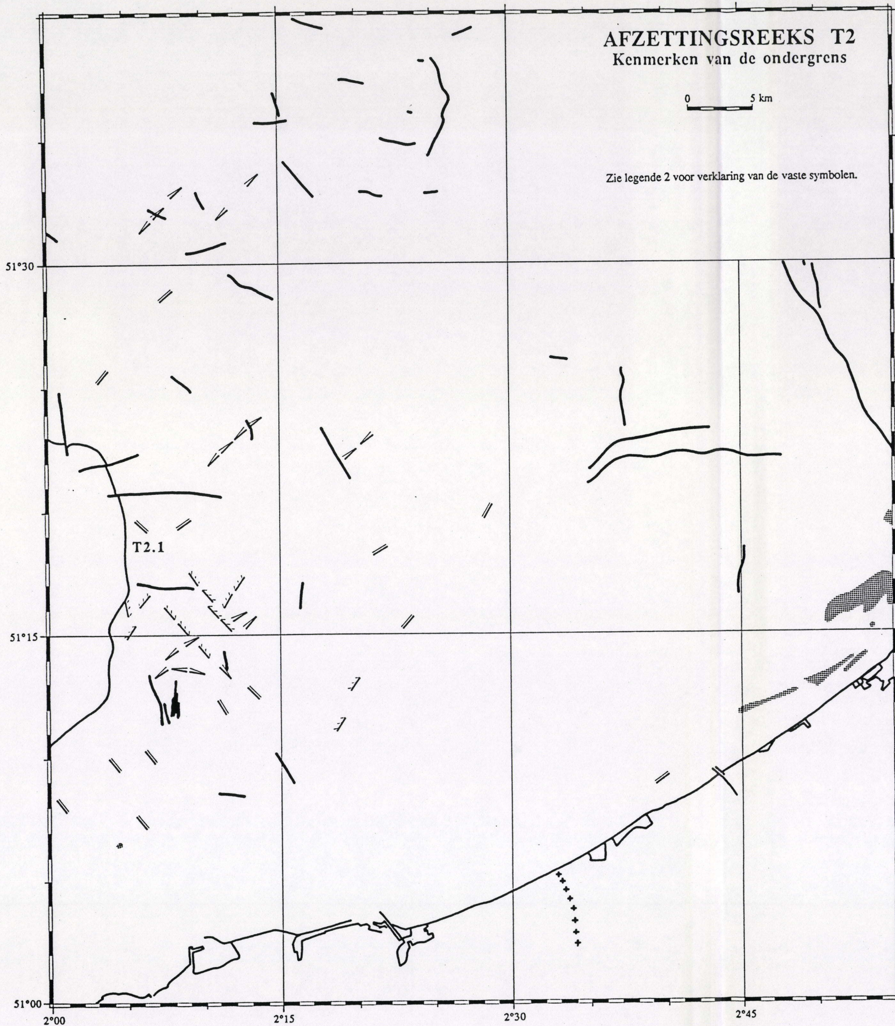
Figuur 34. Seismostratigrafische interpretatiekaart. Afzettingsreeks T2 : Reflektorkonfiguraties ten opzichte van de ondergrens (zie ook Legende 2). Mercatorprojectie op 51°20'.
