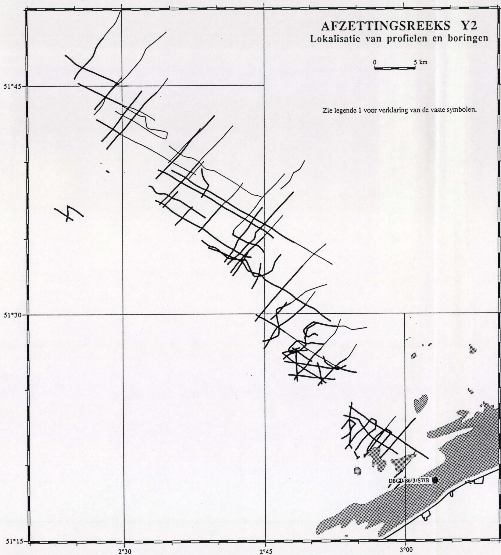
Figuur 42. Seismostratigrafische interpretatiekaart. Afzettingsreeks Y2 : lokalisatie van bij de interpretatie gebruikte profielen en boringen (zie ook Legende 1). Mercatorprojectie op 51°20'.
