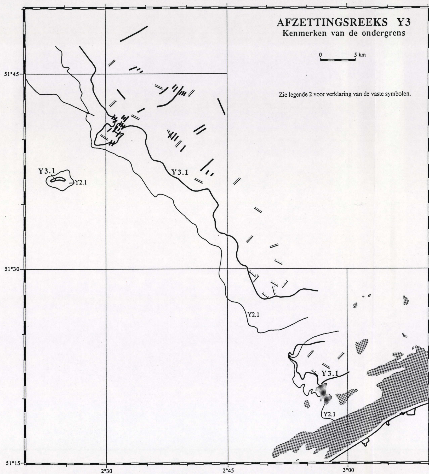
Figuur 48. Seismostratigrafische interpretatiekaart. Afzettingenreeks Y3 : Reflektorkonfiguraties ten opzichte van de ondergrens (zie ook Legende 2). Mercatorprojectie op 51°20'.
