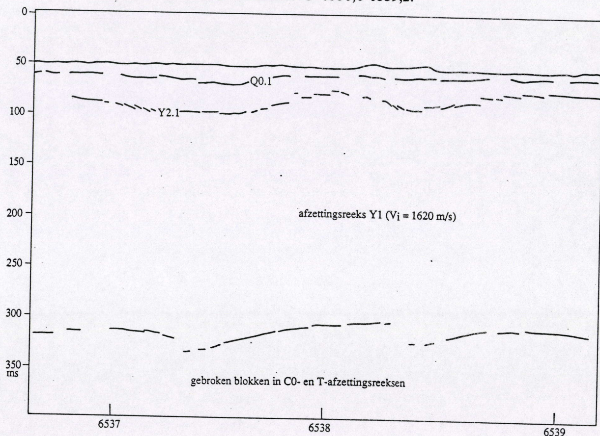
Figuur 133. Seismisch profiel doorheen de vervormingszone van de Noordhinder, dat de relatie weergeeft tussen synklinale plooien in de Y1-afzettingsreeks en een structuur van gekantelde blokken in de onderliggende sekwenties.
