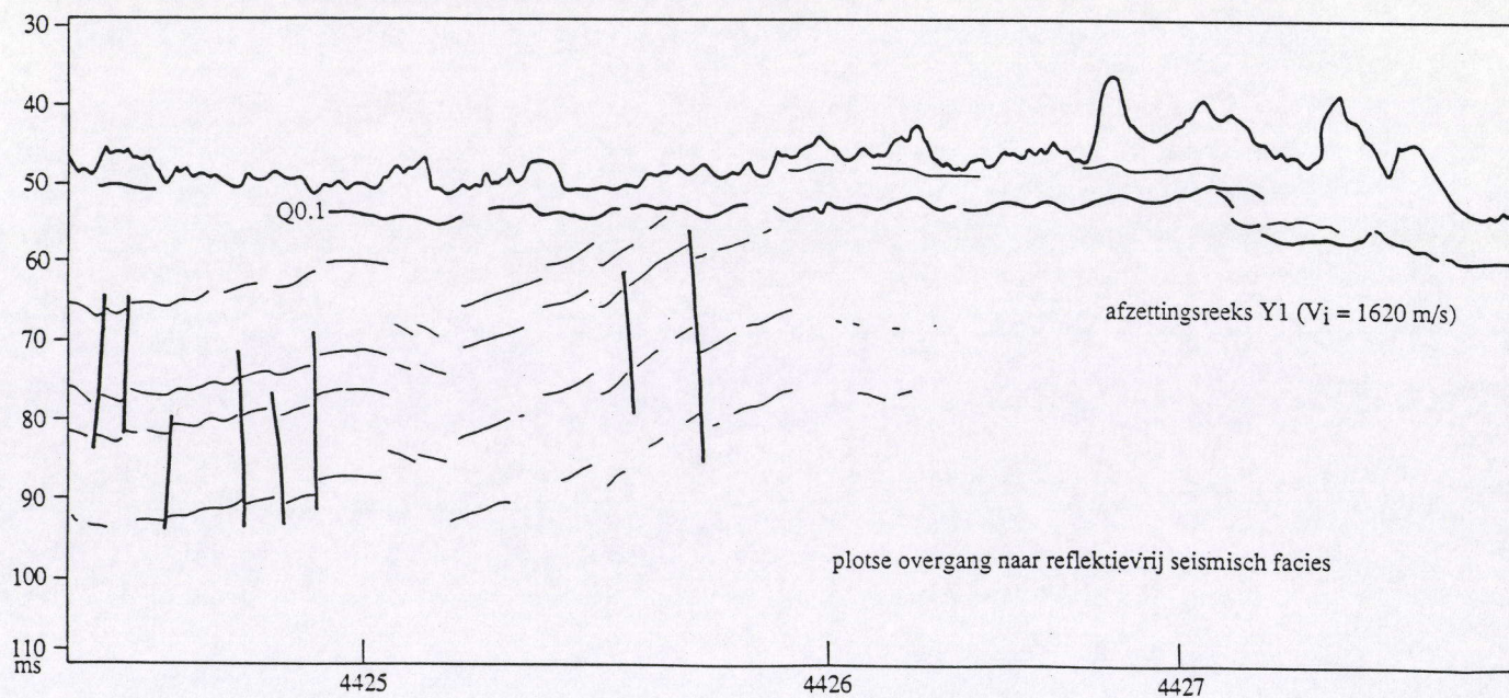
Figuur 107. Seismisch profiel in het centrale deel van het studiegebied, nabij de vervormingszone van de Noordhinder, dat de plotse overgang naar een reflektievrij seismisch facies in de Y1-afzettingenreeks weergeeft.
