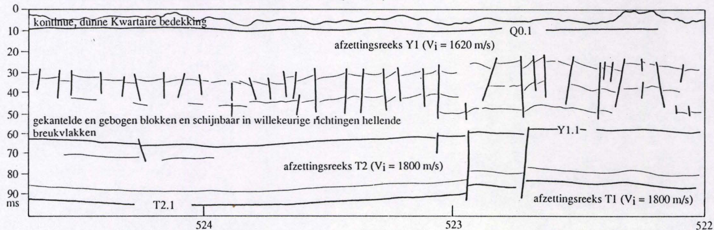
Figuur 110. Seismisch profiel in het centrale deel van het studiegebied, dat de sedimenttektonische vervormingen in het onderste interval van de Y1-afzettingenreeks weergeeft.
