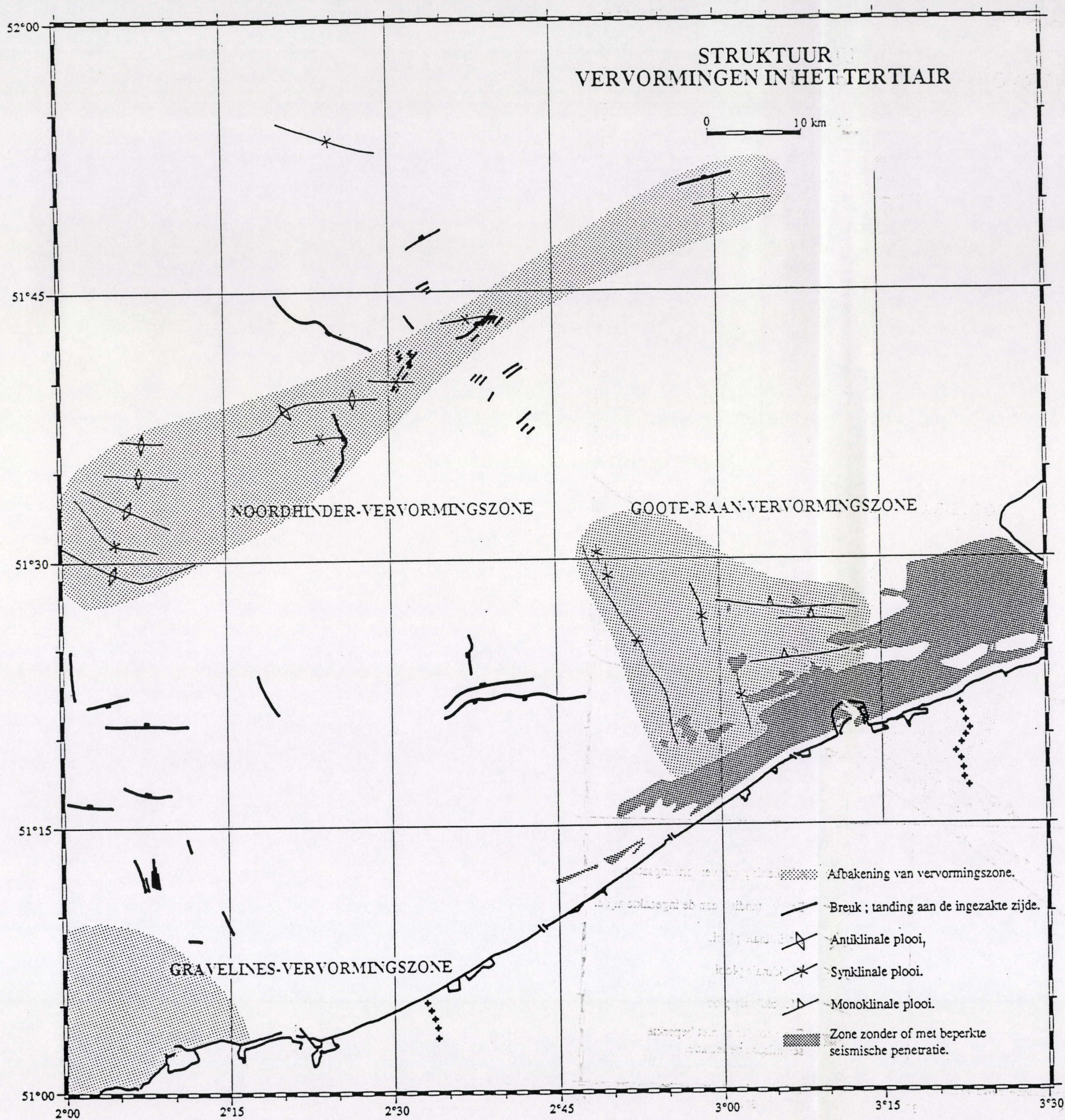
Figuur 130. Overzichtskaart van de structuren, waargenomen in de Tertiaire afzettingen, en lokalisatie van de drie vervormingszones. Mercatorprojectie op 51°20'.
