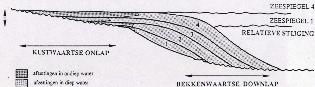
Figuur 7. Relatie tussen kustwaartse onlap met bekkenwaartse downlap en relatieve zeespiegelstijging (naar : VAIL et al., 1977a).
