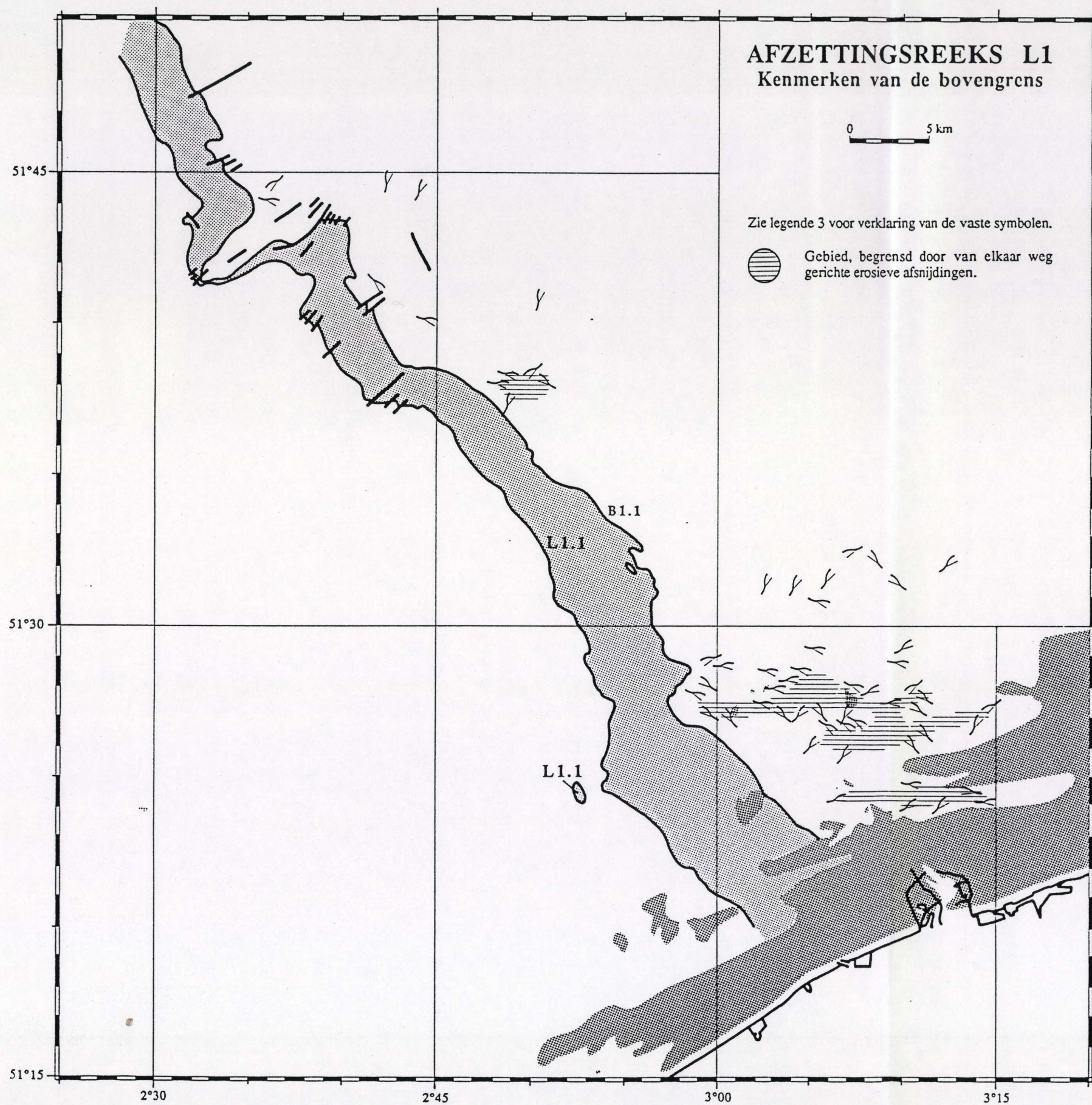
Figuur 65. Seismostratigrafische interpretatiekaart. Afzettingsreeks L1 : Reflektorkonfiguraties ten opzichte van de bovengrens (zie ook Legende 3). Mercatorprojectie op 51°20'.
