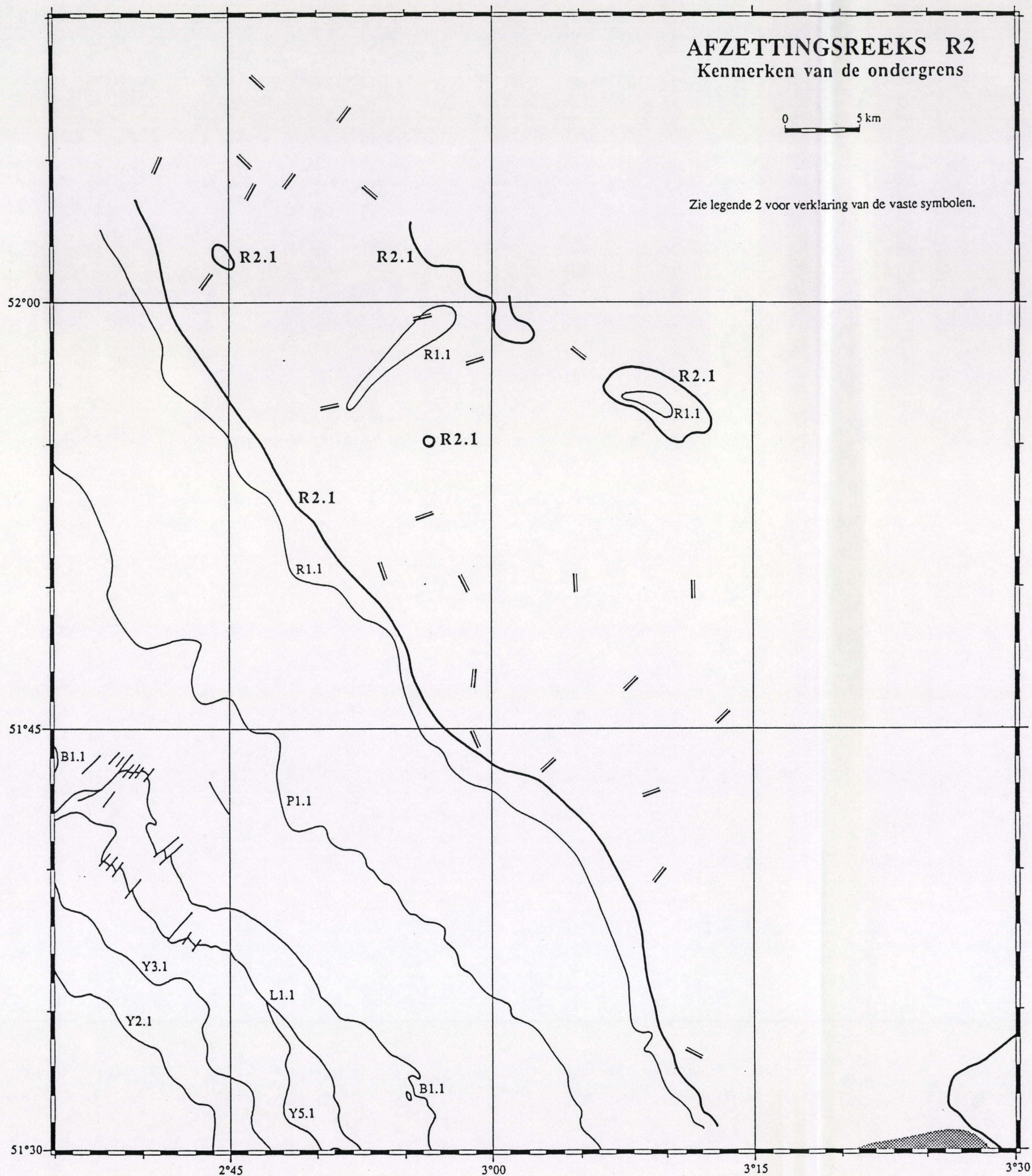
Figuur 85. Seismostratigrafische interpretatiekaart. Afzettingssreeks R2 : Reflektorkonfiguraties ten opzichte van de ondergrens (zie ook legende 2). Mercatorprojectie op 51°20'.
