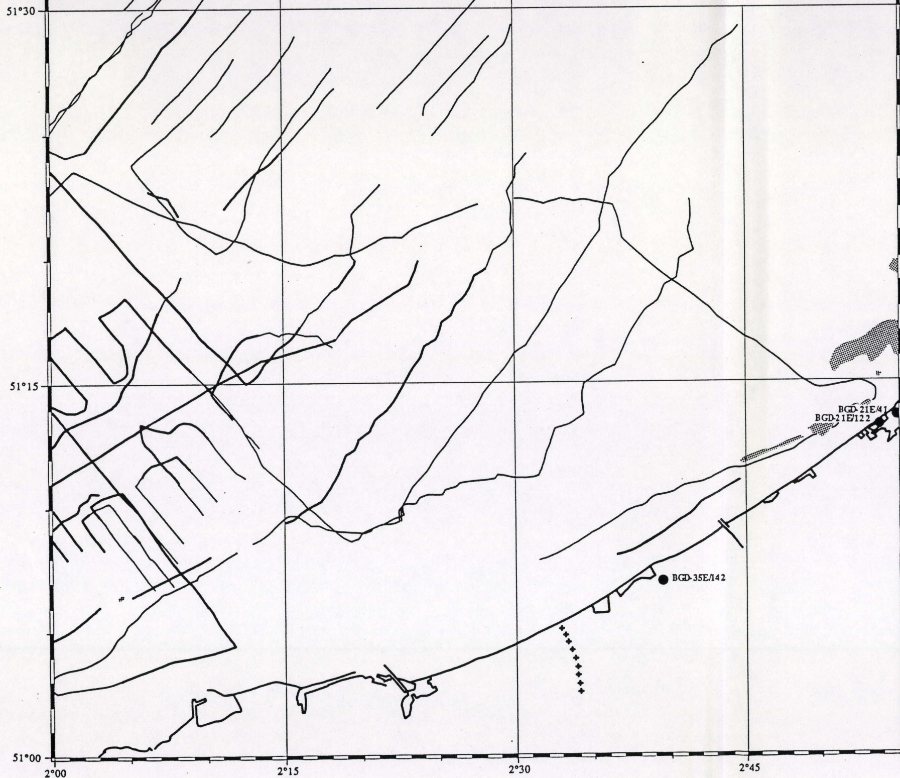
Figuur 31. Seismostratigrafische interpretatiekaart. Afzettingsreeks T1 : lokalisatie van bij de interpretatie gebruikte profielen en boringen (zie ook Legende 1). Mercatorprojectie op 51°20'.
