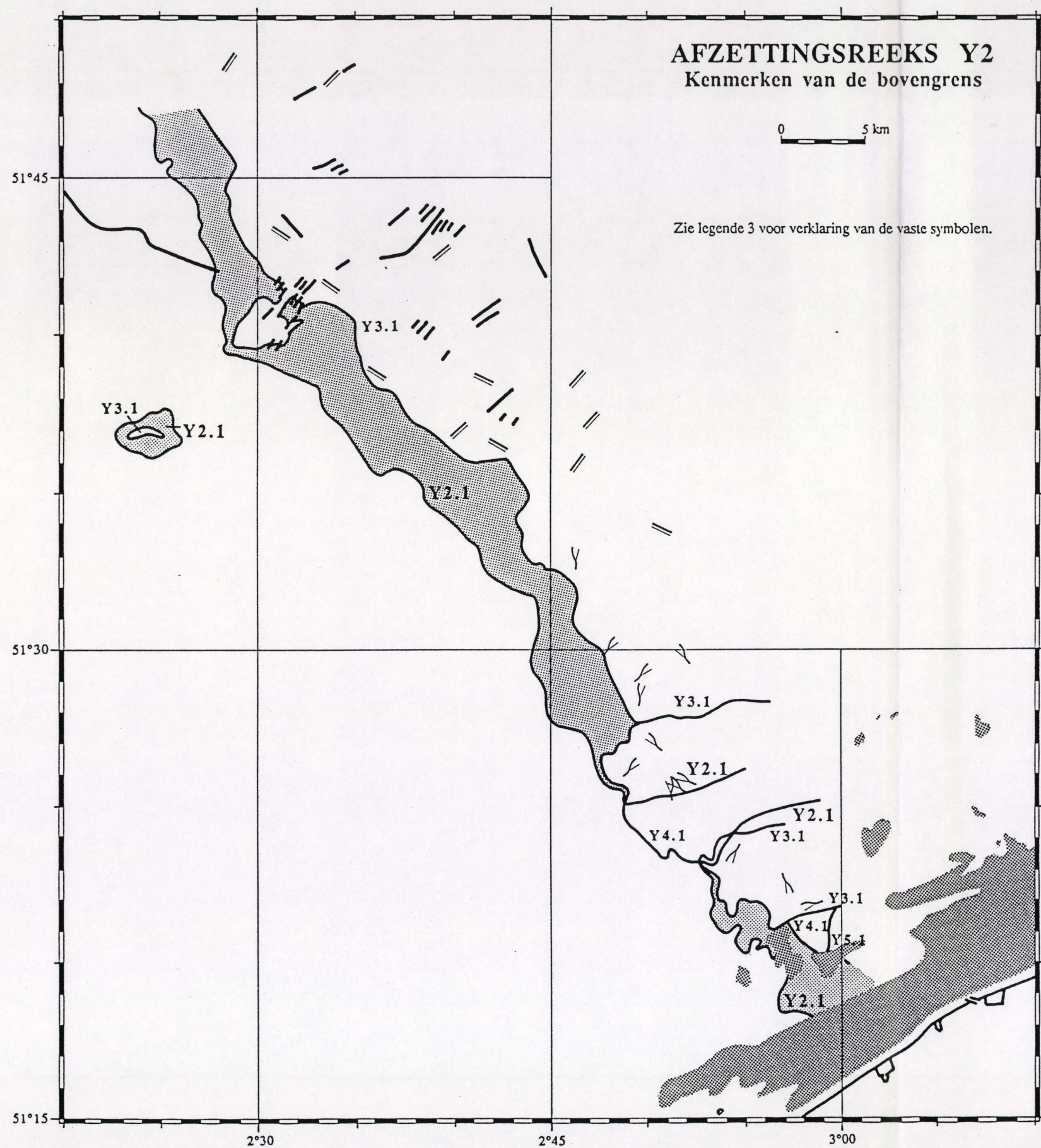
Figuur 45. Seismostratigrafische interpretatiekaart. Afzettingsreeks Y2 : Reflektorkonfiguraties ten opzichte van de bovengrens (zie ook Legende 3). Mercatorprojectie op 51°20'.
