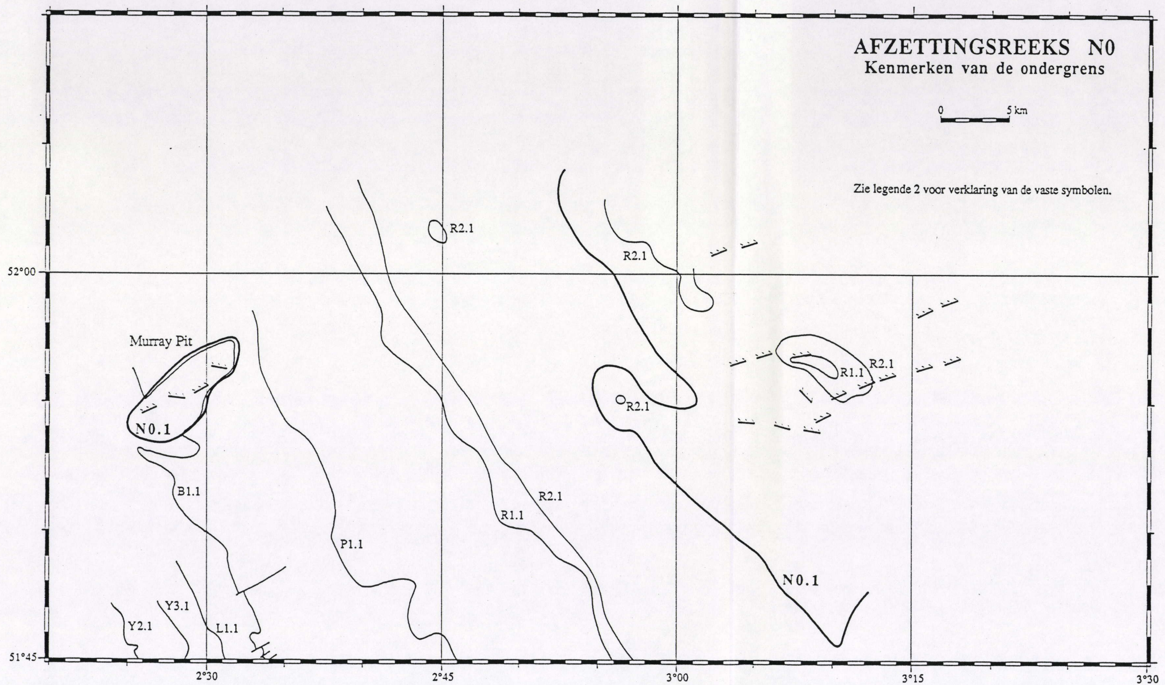
Figuur 94. Seismostratigrafische interpretatiekaart. Afzettingenreeks N0 : Reflektorkonfiguraties ten opzichte van de ondergrens (zie ook legende 2). Mercatorprojectie op 51°20'.
