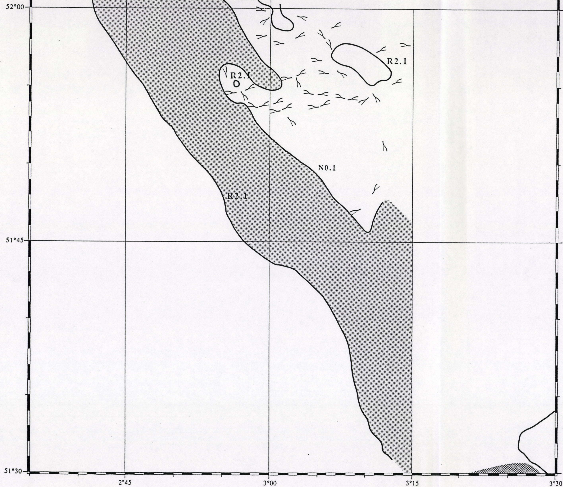
Figuur 86. Seismostratigrafische interpretatiekaart. Afzettingen R2 : Reflektorkonfiguraties ten opzichte van de bovengrens (zie ook legende 3). Mercatorprojectie op 51°20'.
