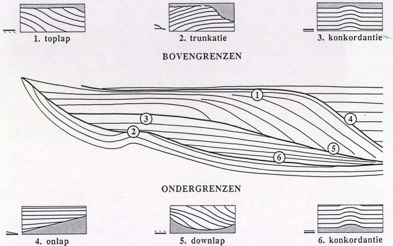
Figuur 6. Verschillende types van reflektorkonfiguraties ten opzichte van de begrenzing van een afzettingsreeks. Nummers verwijzen naar beschrijvingen in de tekst ; bijgevoegde symbolen worden gebruikt op de seismostratigrafische interpretatiekaarten (zie Legendes 2 en 3).
