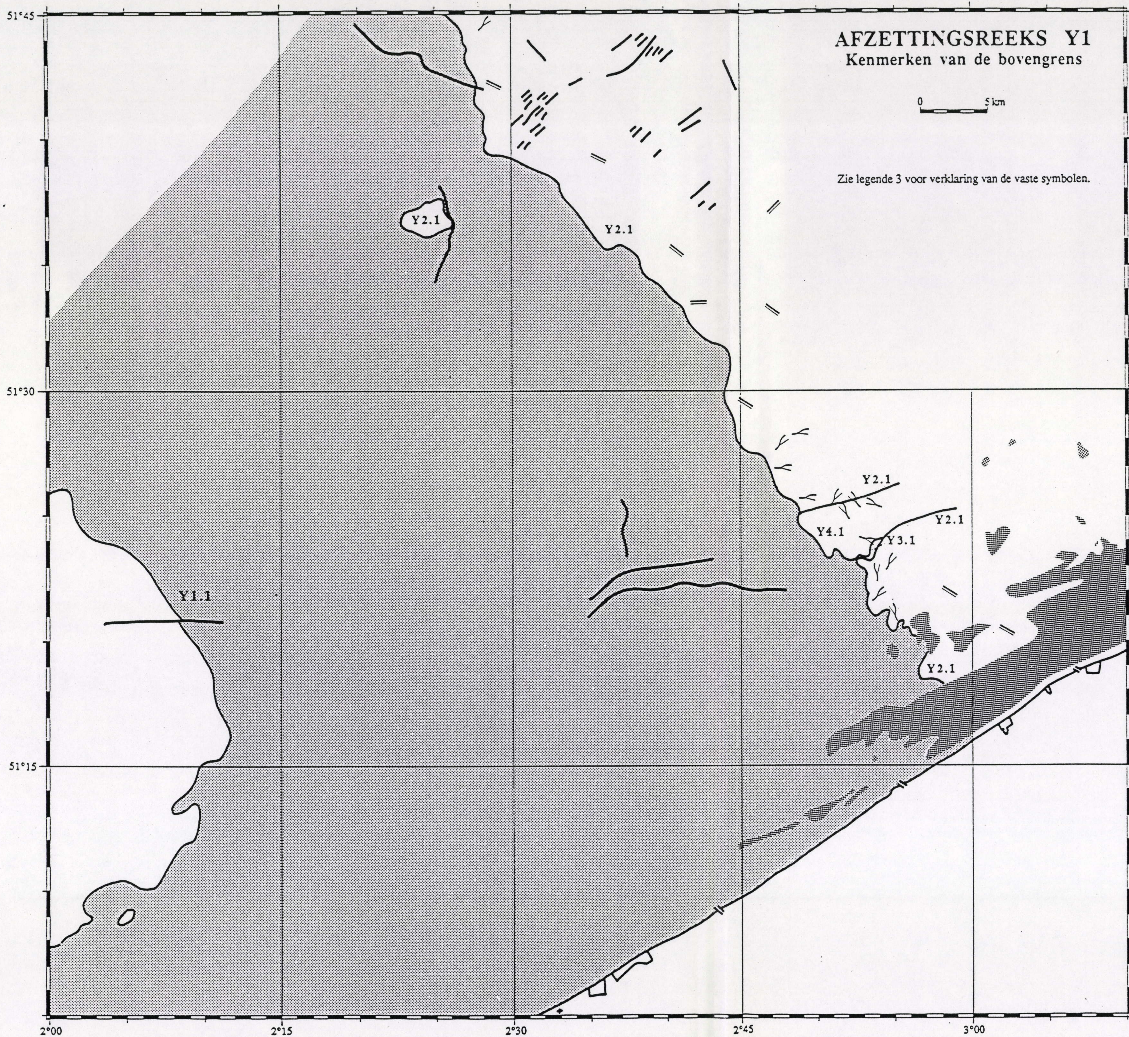
Figuur 41. Seismostratigrafische interpretatiekaart. Afzettingsreeks Y1 : Reflektorkonfiguraties ten opzichte van de bovengrens (zie ook Legende 3). Mercatorprojectie op 51°20'.
