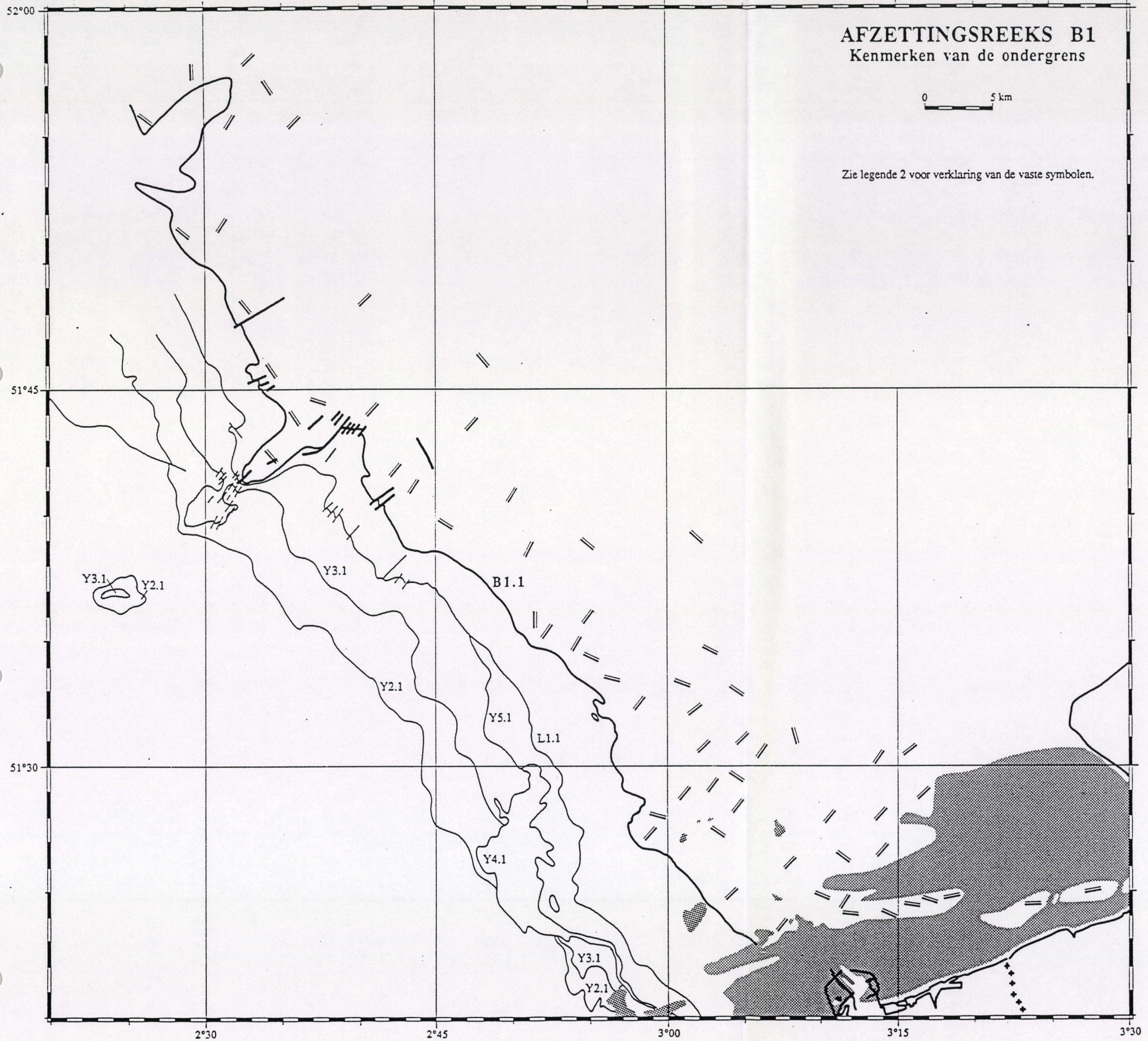
Figuur 69. Seismostratigrafische interpretatiekaart. Afzettingsreeks B1 : Reflektorkonfiguraties ten opzichte van de ondergrens (zie ook Legende 2). Mercatorprojectie op 51°20'.
