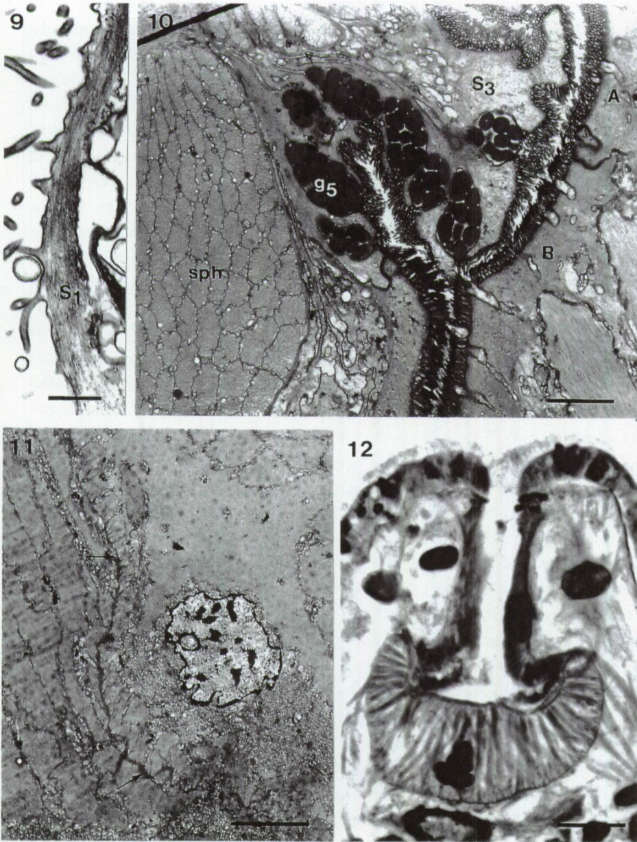
Figs.9-11. Tenerrhynchus magnus .
