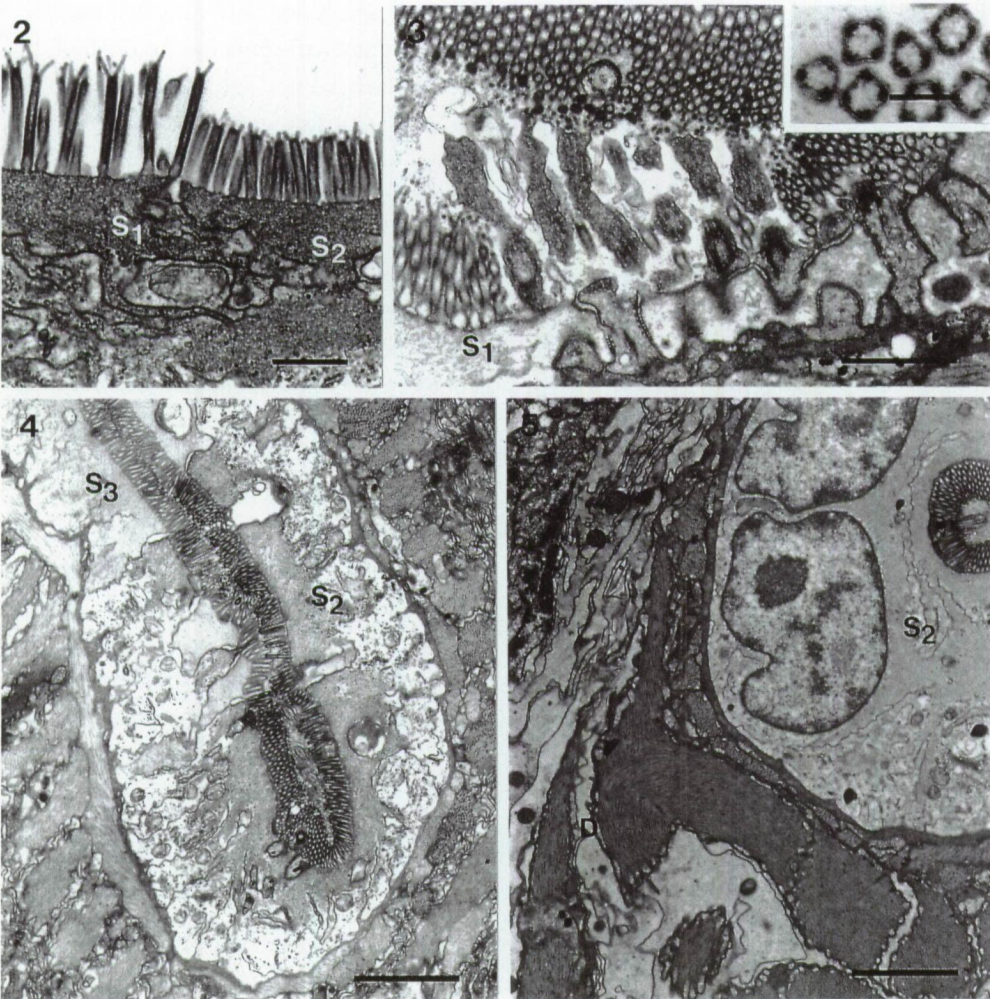
Figs. 2-5. Itaipusa karlingi .
