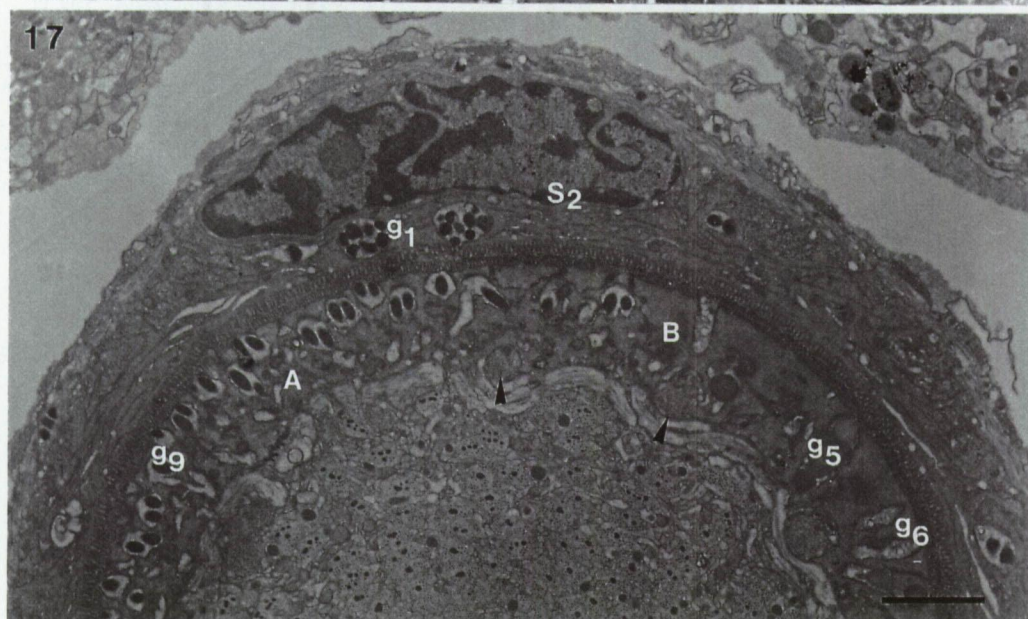
Figs 16-17. Typhlopolycystis rubra .
