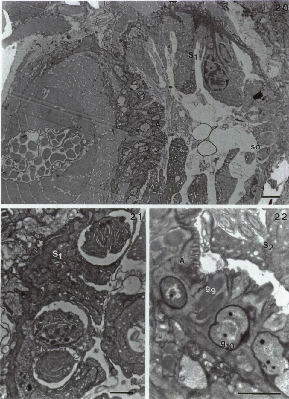
Figs 20-22. Gnathorhynchus conocaudatus .
