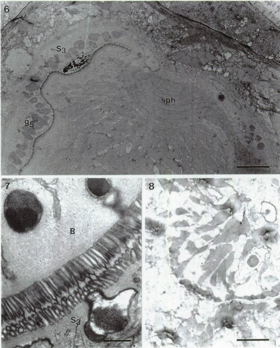
Figs 6-8. Itaipusa karlingi .
