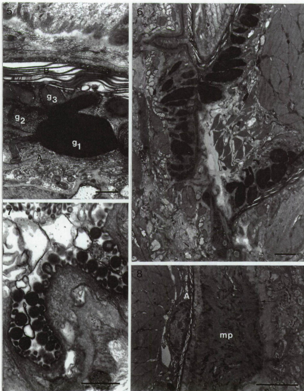
Figs 5-8. Placorhynchus octaculeatus .
