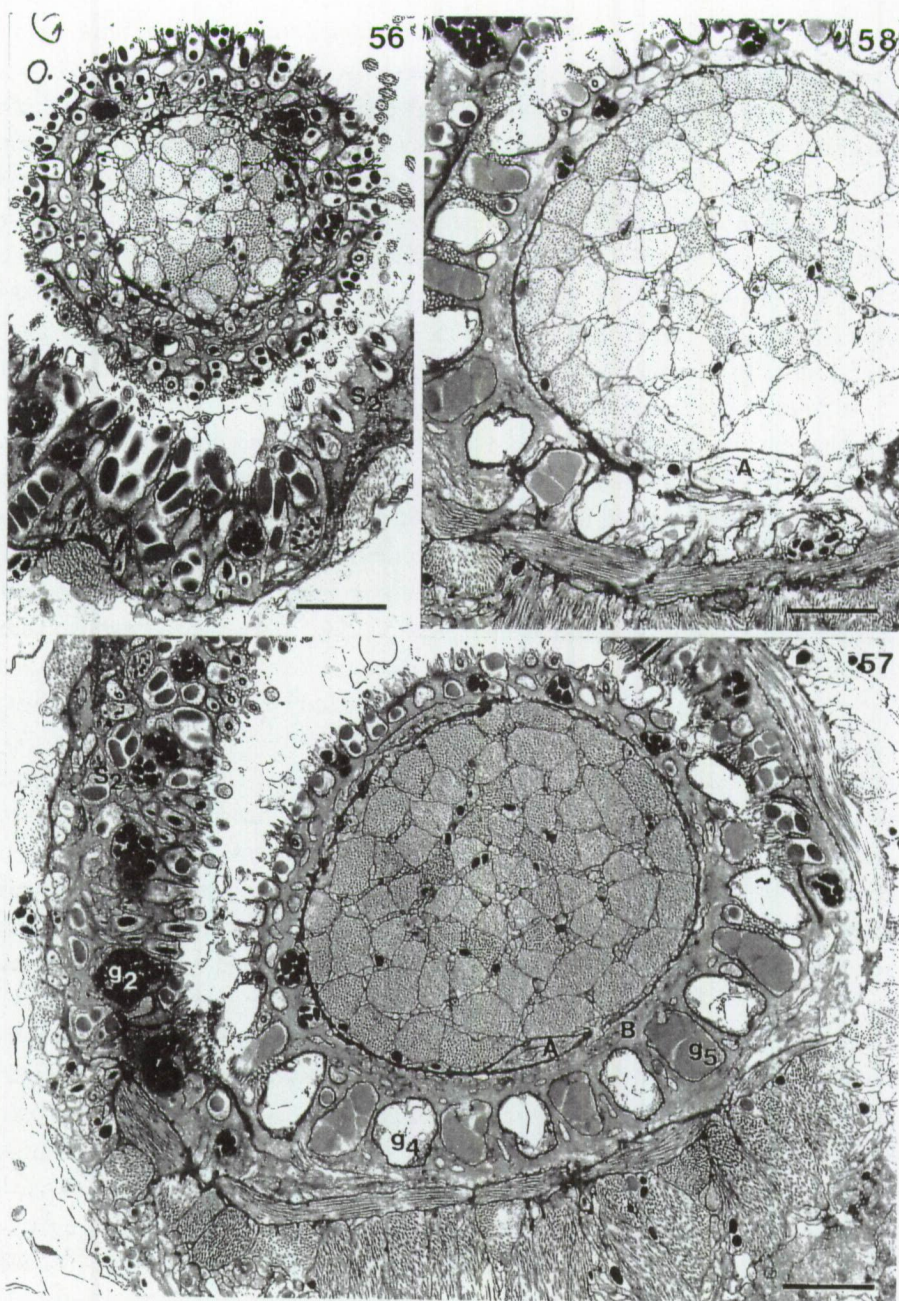
Figs 56-58. Ptyalorhynchus coecus .
