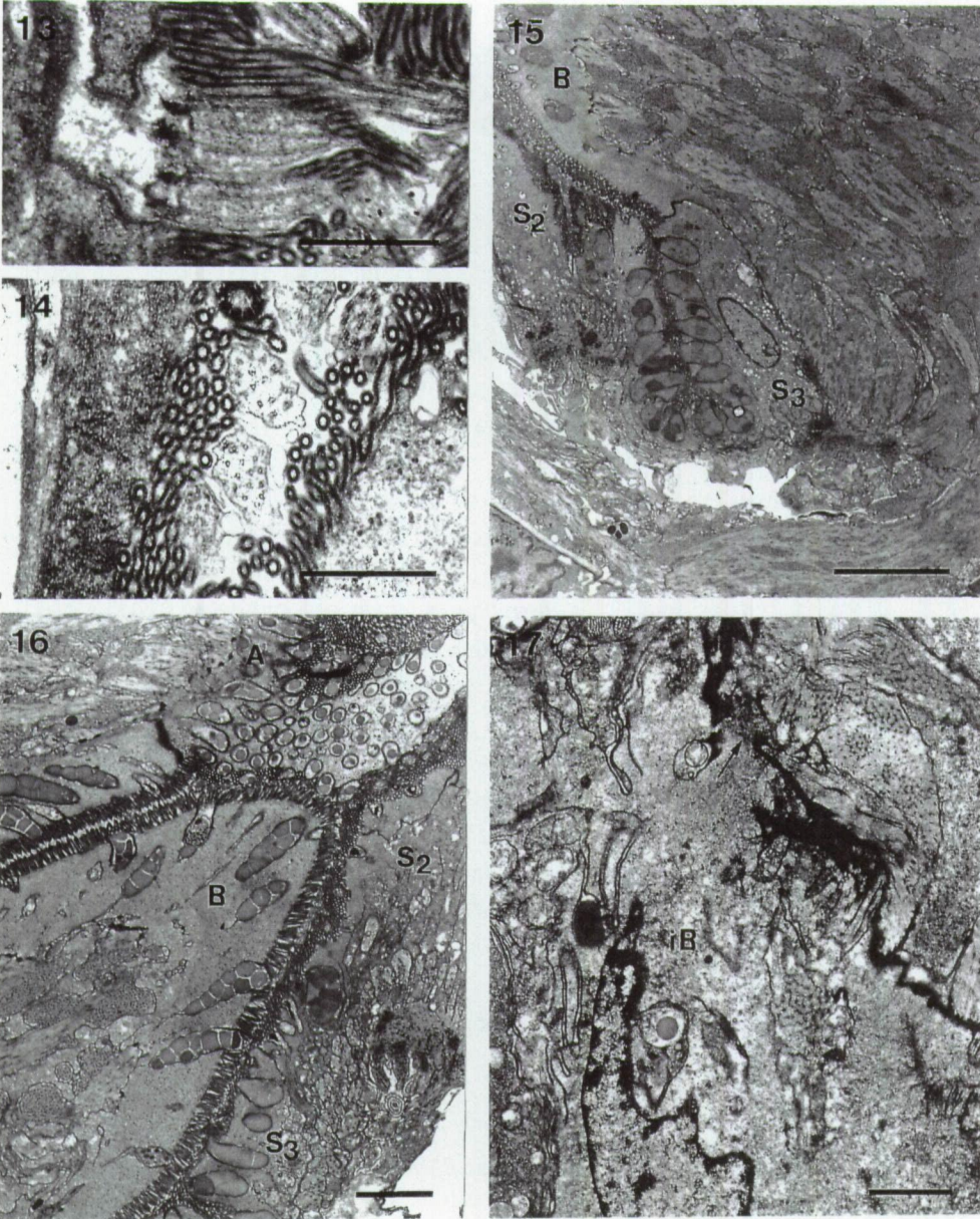
Figs 13-17. Parautelga bilioi .
