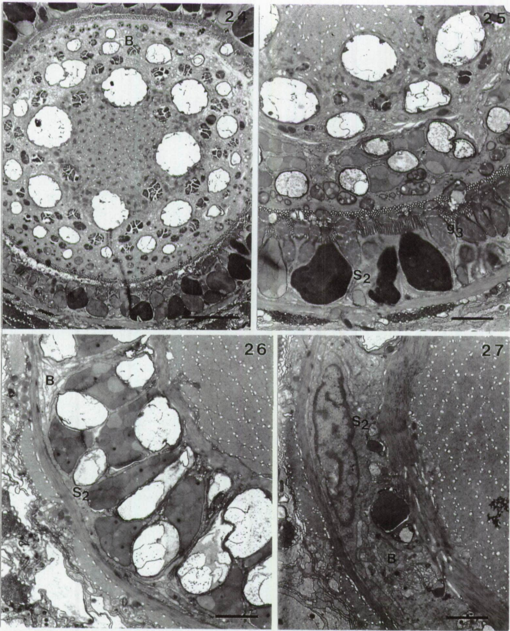
Figs 24-27. Zonorhynchus sp.
