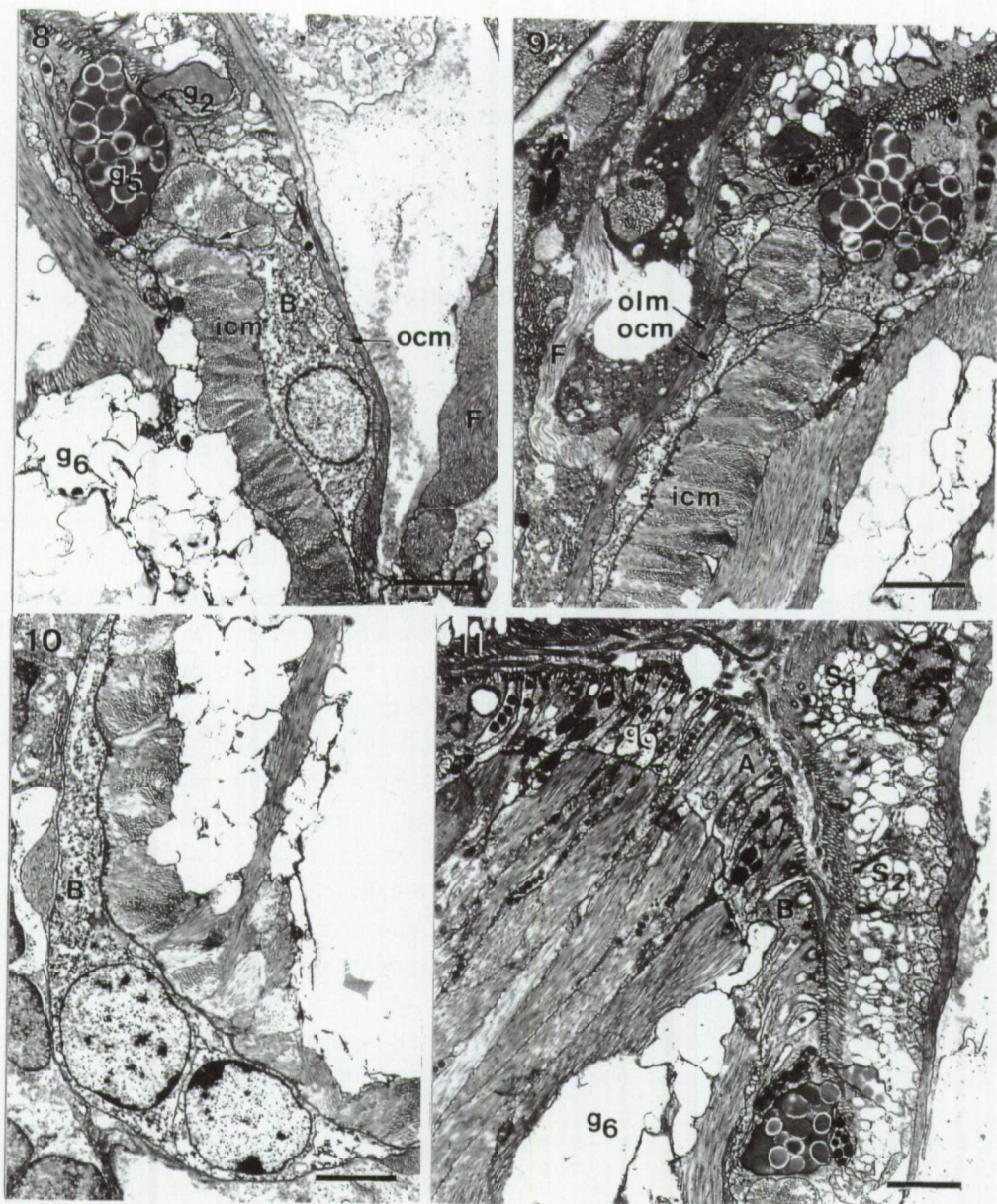
Figs 8-11. Toia calceformis .
