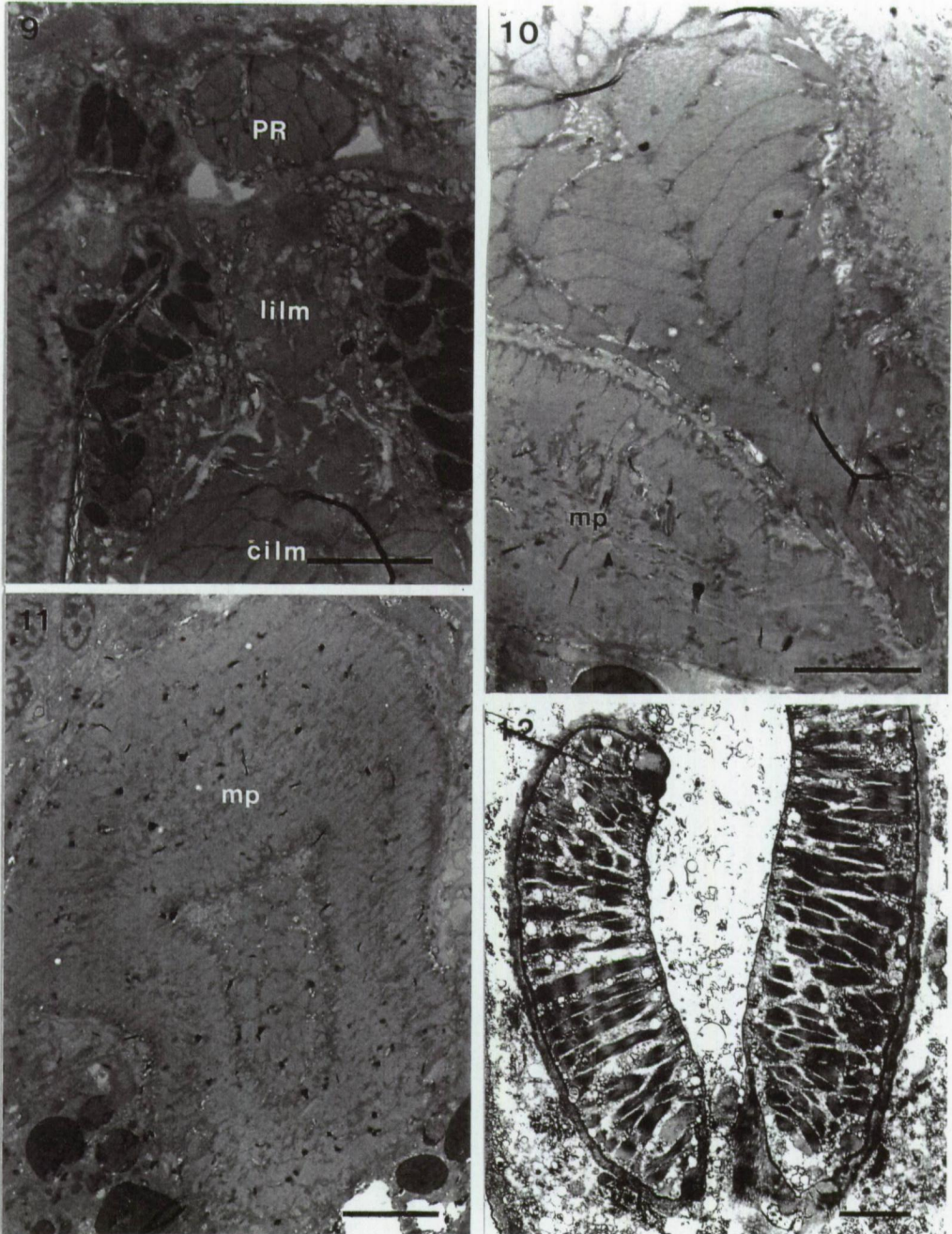
Figs 9-11. Placorhynchus octaculeatus .
