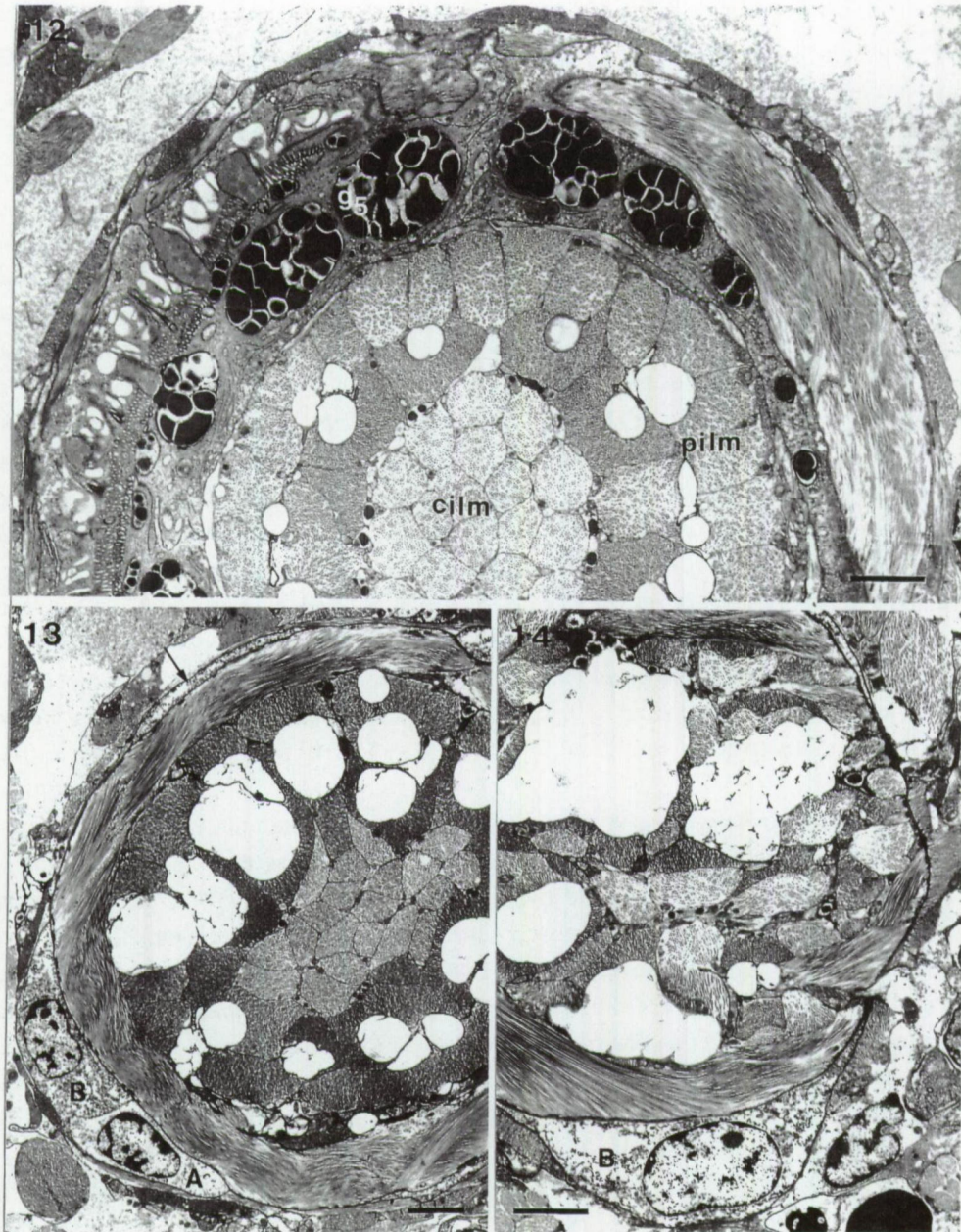
Figs 12-14. Toia calceformis .
