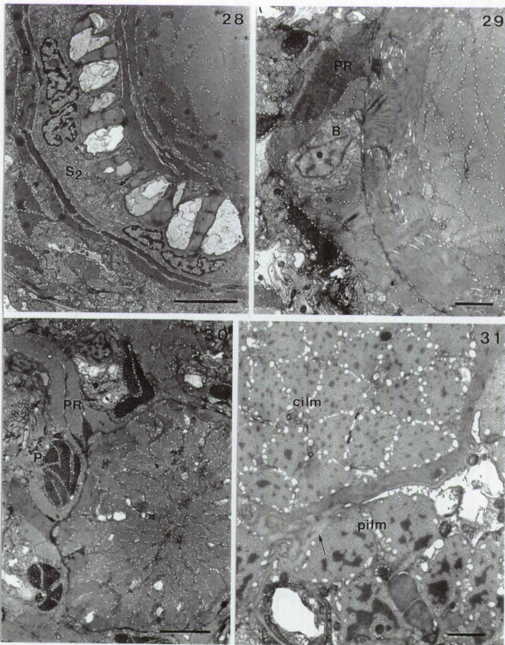
Figs 28-31. Zonorhynchus seminascatus .
