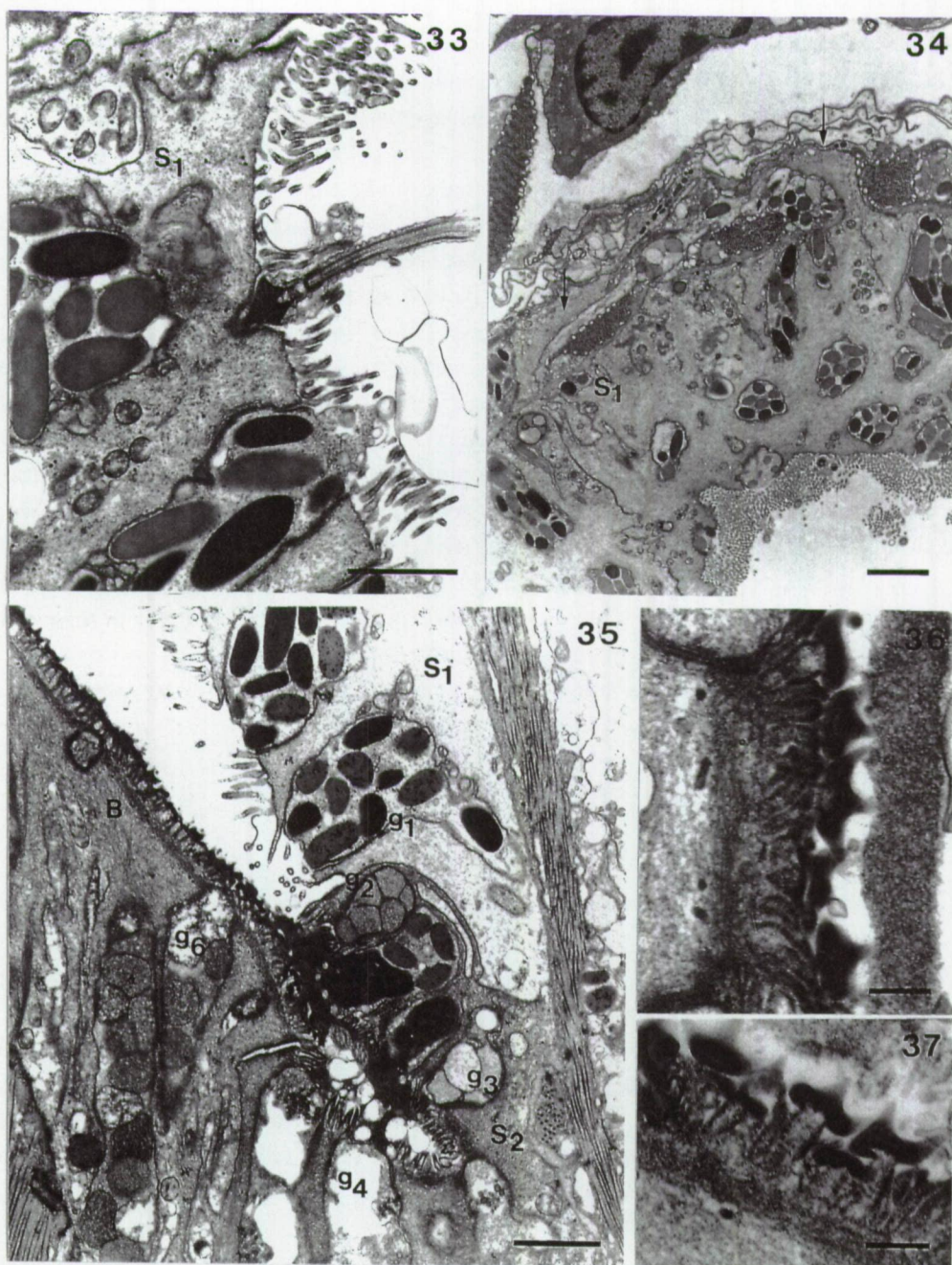
Figs 33-37. Ethmorhynchus anophthalmus .
