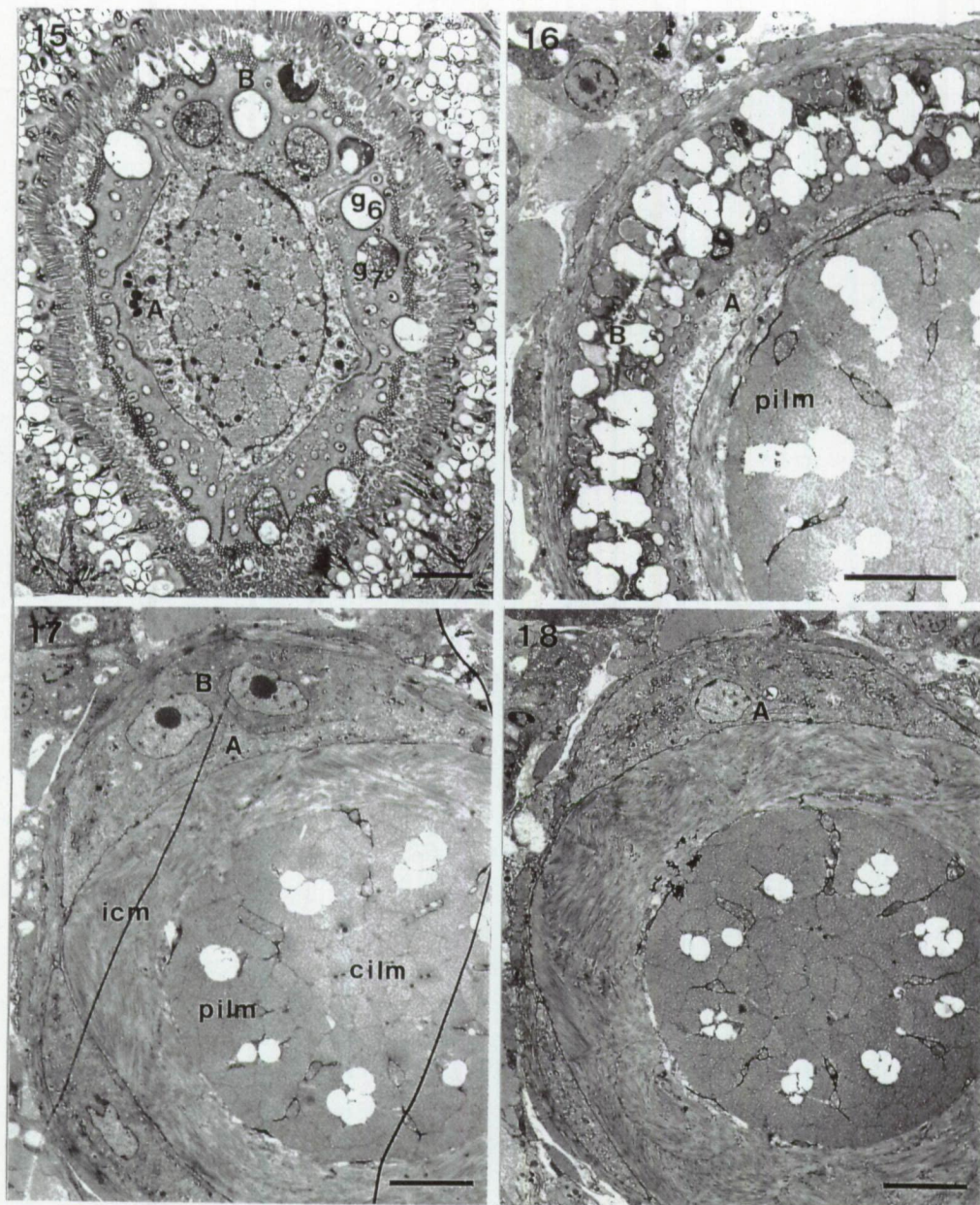
Figs 15-18. Nannorhynchides herdlaensis .
