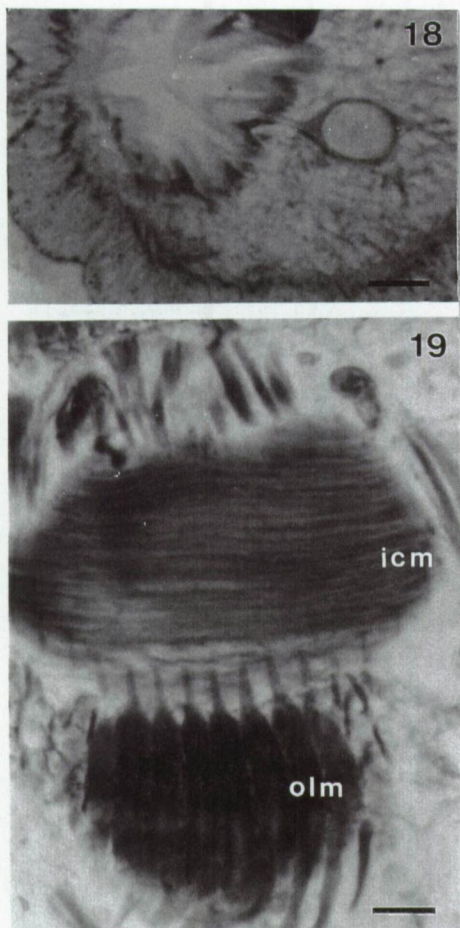
Figs. 18-19. Crassicollum musculare .
