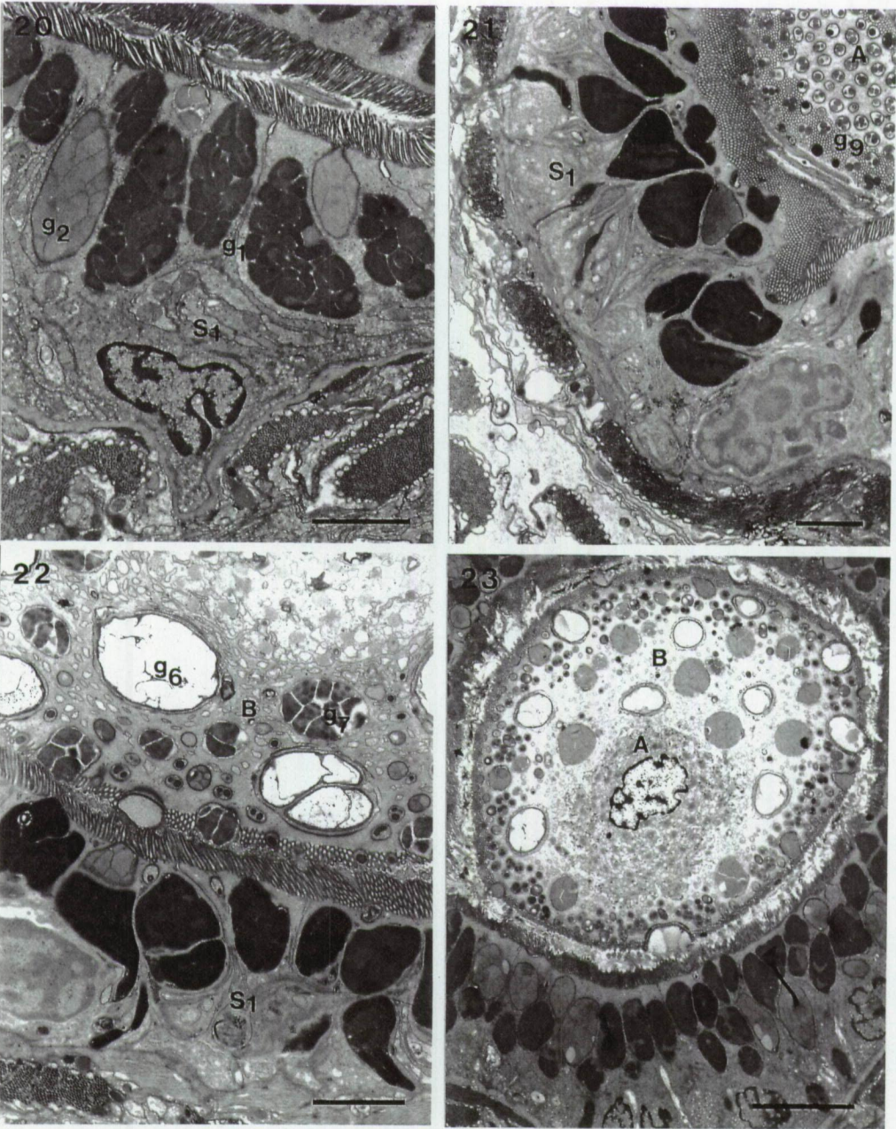
Figs 20-21. Zonorynchus seminascatus .
