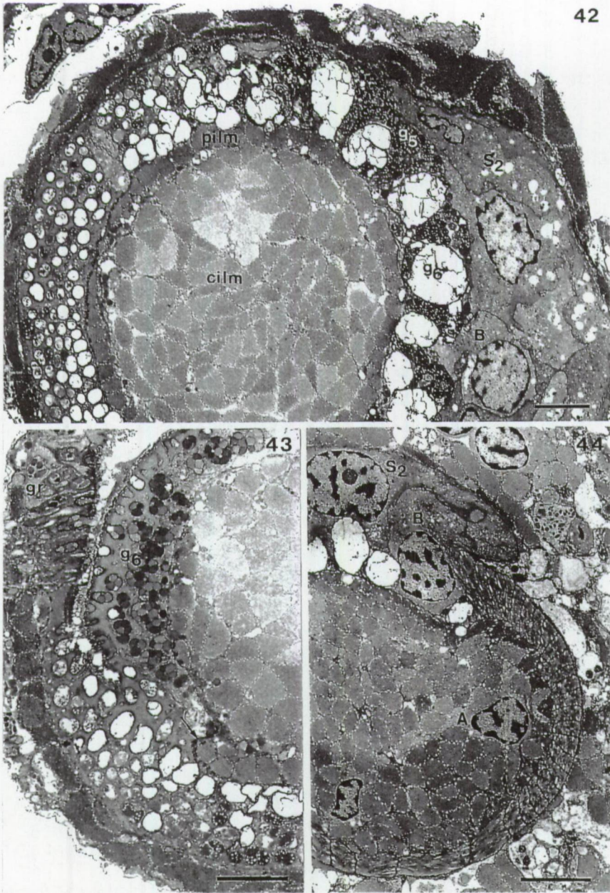
Figs 42-44. Ethmorhynchus anophthalmus .
