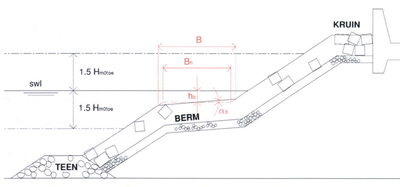
Figuur 5 Bepaling van B , B_b , \tan \alpha_b en h_b
