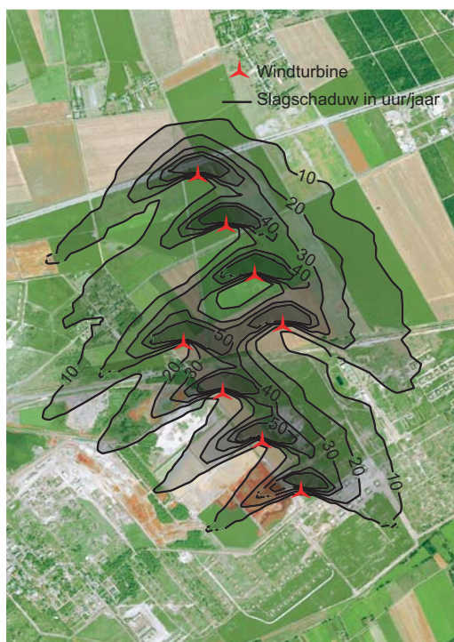
Schaduwcontour rond windmolenpark van 8 windturbines (Bron: Aspiravi)
