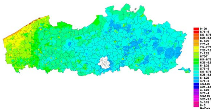
Windplan Vlaanderen Gemiddelde windsnelheid [m/s] op 75 m ashoogte
